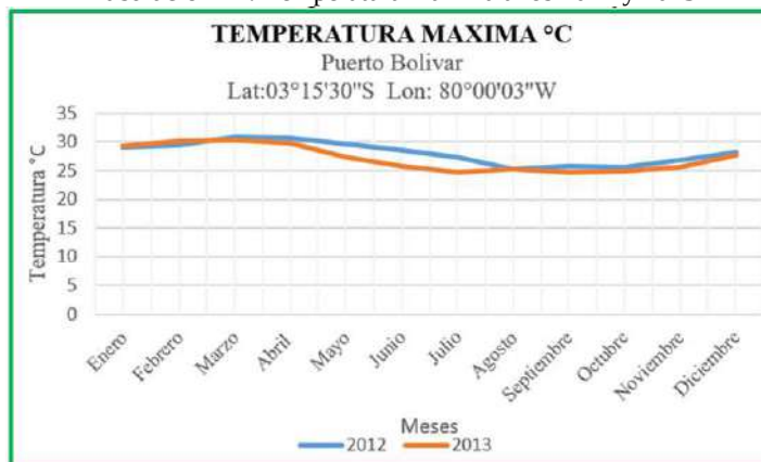
Ilustración 11: Temperatura máxima años 2012 y 2013
