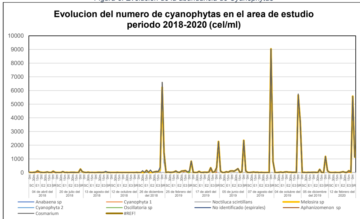
Figura 5. Evolución de la abundancia de Cyanophytas
