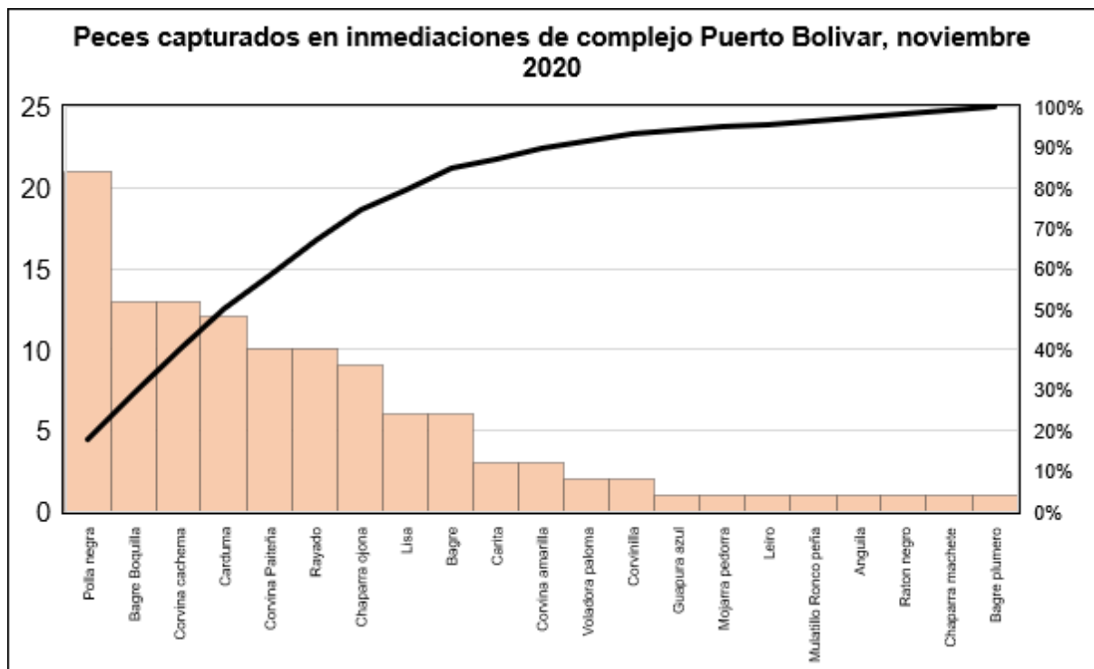
Figura 49. Abundancia de recursos pesqueros capturados en las inmediaciones de Puerto Bolívar
