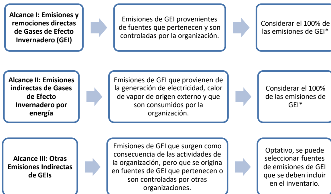
Figura 3. Definiciones y requisitos según la ISO 14064-1.
