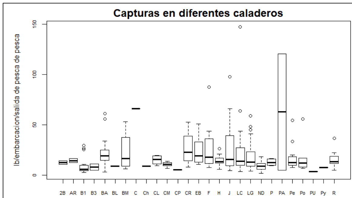
Figura 7. Capturas categorizadas en diferentes caladeros en noviembre 2020: 2B= 2 boyas, AR=Afuera del rio, B1= Boya 1, B3= Boya 3, BA= Bajo Alto, BM= Boya Amarilla, C= El Coco, Ch=Chupadores, CL= Cabeza de Loma, CM= Canal del medio, CP= Caña Parada, CR= Costa Rica, EB=El Bravo, F= El faro, H= Las Huacas, J= Jambelí, LC= Loma Chica, LG=Loma Grande, ND=No determinado, P= La Poza, PA= Punta Arena, Pe= El Petrolero, Po= La Polanca, PU= La Puntilla, PY= Punta Payana, R= El Rio
