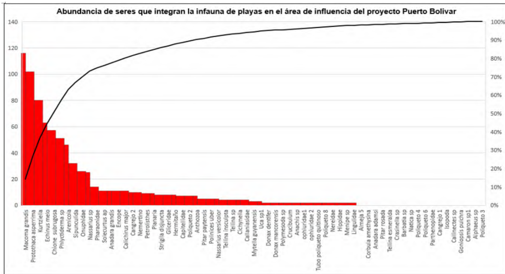
Figura 39. Seres de la infauna más abundantes en el área de influencia del Proyecto
