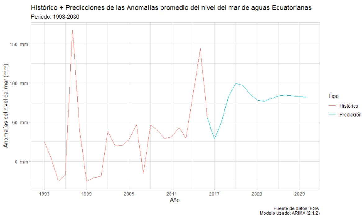
Figura 2. Series de tiempo de Anomalías del nivel del mar en aguas ecuatorianas
