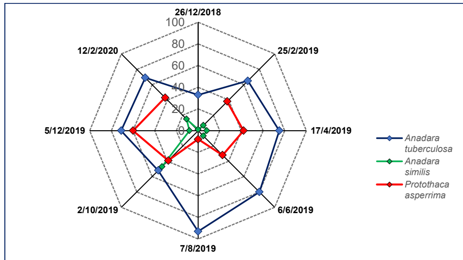
Figura 1. Fluctuación de abundancia de bivalvos comerciales colectados en el periodo 2018-2020 en la AUSCEM "Vikingos del Mar"
