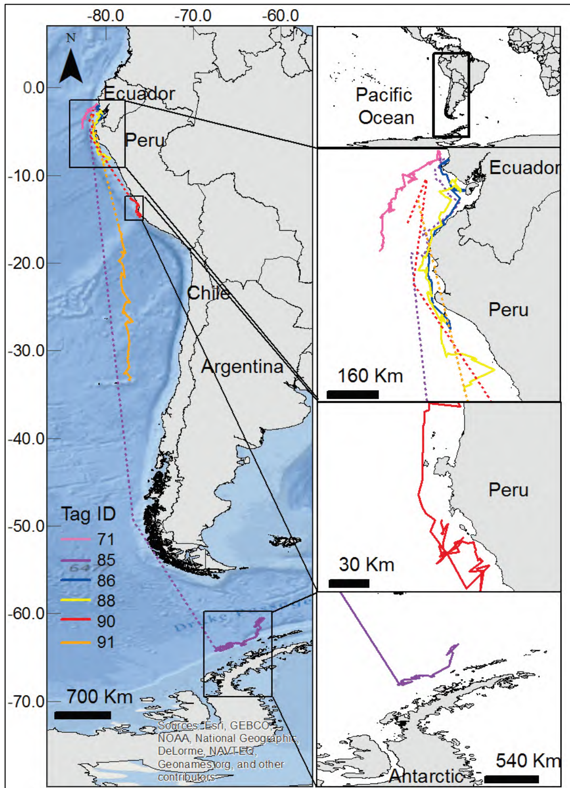
Figura 52. Rutas migratorias de Megaptera novangliae obtenidas mediante monitoreo satelital (Felix y Guzman, 2014).
