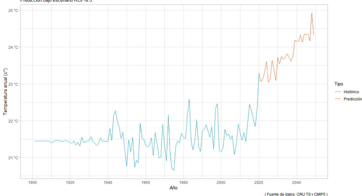
Serie de tiempo de Temperatura anual de Ecuador (Histórico + Predicción) Predicción bajo escenario RCP-8.5
