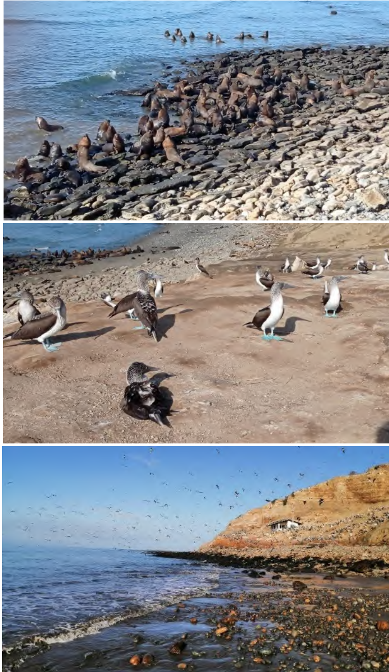
Registro Fotográfico 3. Lobos marinos Otaria flavescens, central Piqueros Patas azules Sula nebouxi y abajo abundancia de aves en Isla Santa Clara, 10 de abril 2021
