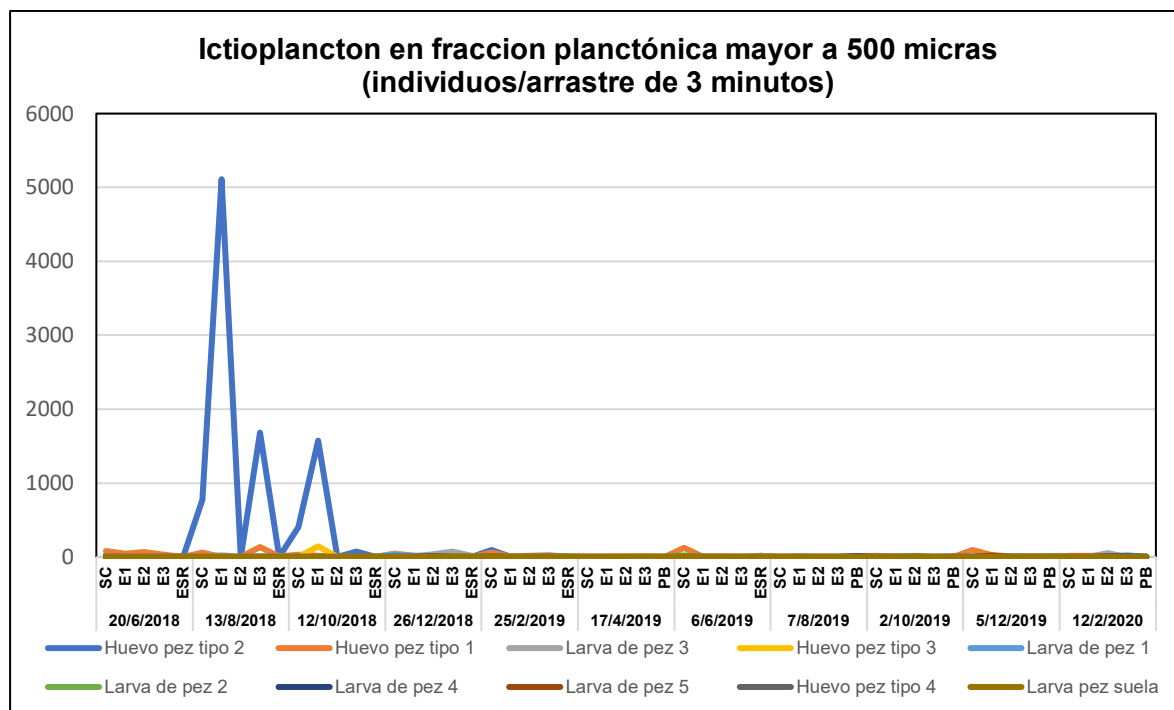
Figura 21. Ictioplanctones más abundantes dentro de fracción superior a 500 micras de zooplancton
