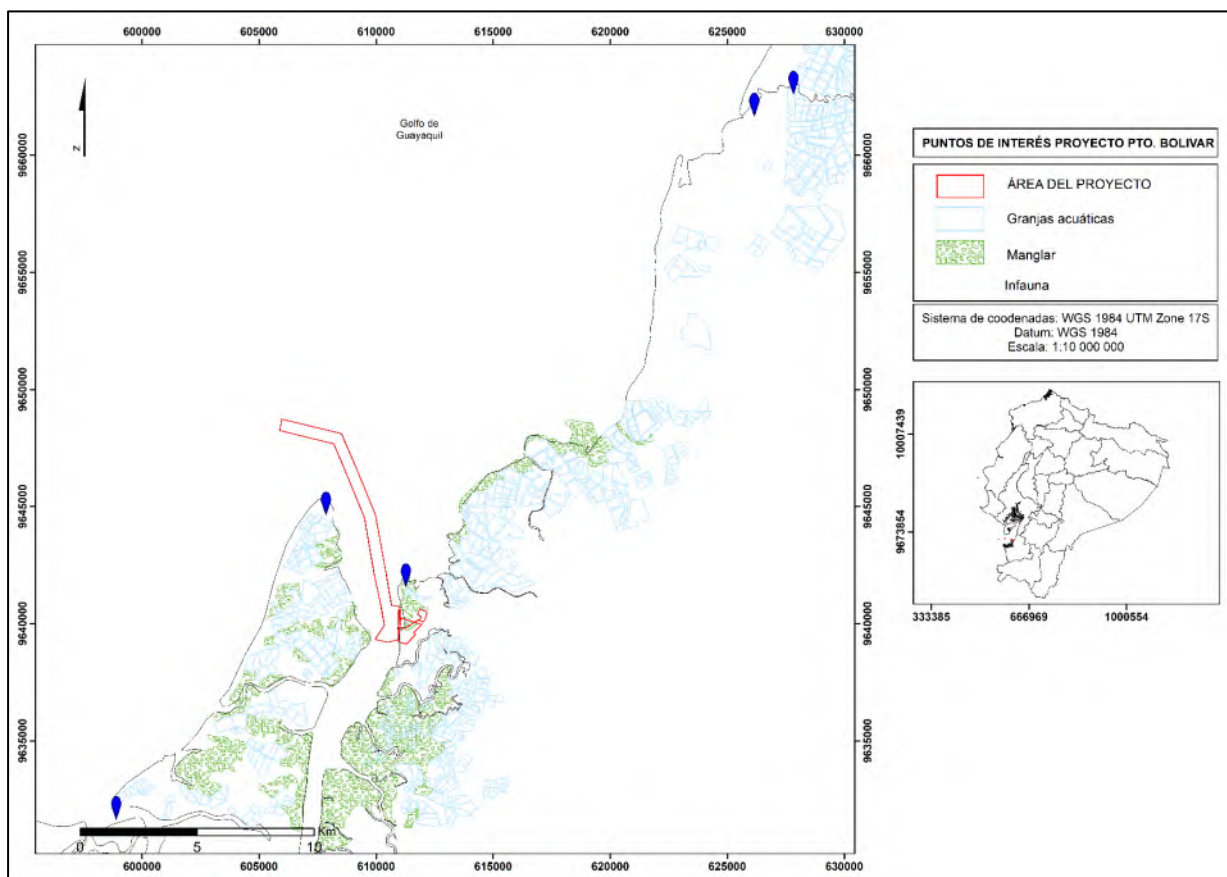
Figura 38. Ubicación de playas donde se analizó infauna.
