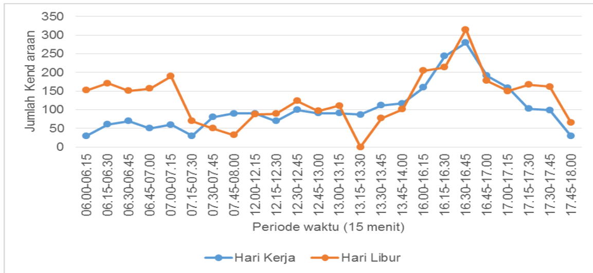
Gambar 2.157. Fluktuasi Arus Lalu lintas di Simpang 3 Tak Bersinyal Tubanan (Sumber: Survei Lapangan, 2015)
