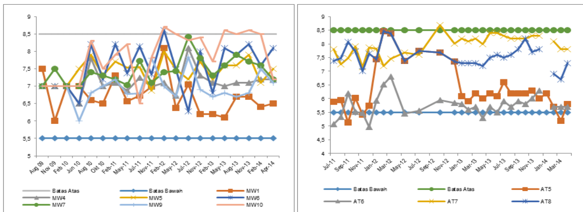
Gambar 2.40. Grafik kualitas air tanah parameter pH hasil pemantauan Unit 1&2 (kiri) dan Unit 3&4 (kanan) (sumber: Hasil pemantauan Unit 1-4, 2010-2014)
