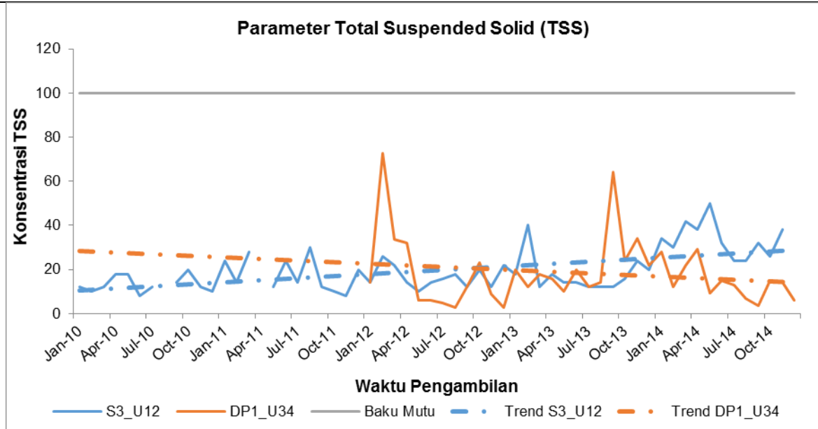
Gambar 2.20. Profil TSS pada PLTU Tanjung Jati B Unit 1&2 dan PLTU Tanjung Jati B Unit 3&4
