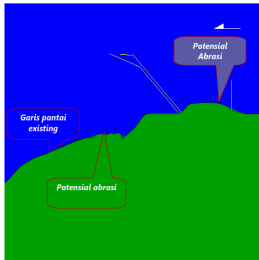
Gambar 2.127. Hasil Model Musim Peralihan 1 Perubahan Garis Pantai di Perairan Tanjung Jati, Jepara, Kondisi Eksisting Tahun Pertama
