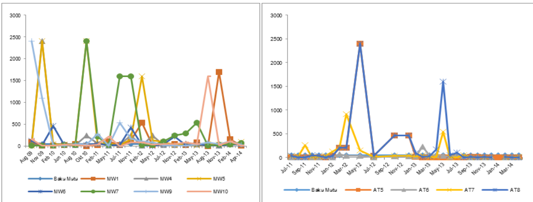
Gambar 2.39. Grafik kualitas air tanah parameter Total Coliform hasil pemantauan Unit 1&2 (kiri) dan Unit 3&4 (kanan) (sumber: Hasil pemantauan Unit 1-4, 2010-2014)
