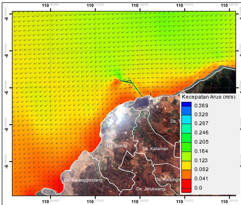
Gambar 2.102. Hasil permodelan arus musim peralihan 1 zona 1 kondisi eksisting (surut menuju pasang) (Sumber : Hasil Pemodelan, September 2015)
