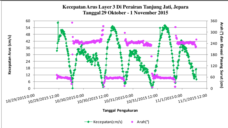
Gambar 2.77. Kecepatan arus kedalaman 5,4 – 7,2 meter ( layer 3 ) di Perairan Tanjung Jati, Jepara Tanggal 29 Oktober - 1 November 2015 (Sumber: Analisis Data, November 2015)
