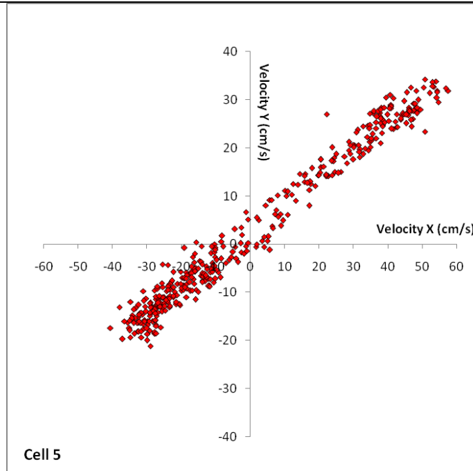
Gambar 2.93. Scatter plot kecepatan arus kedalaman 1,8 – 3,6 meter ( layer 5 ) di Perairan Tanjung Jati, Jepara Tanggal 29 Oktober - 1 November 2015 (Sumber : Analisis Data, November 2015)
