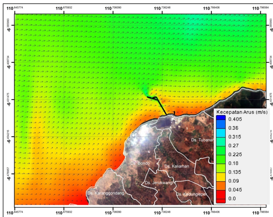
Gambar 2.105. Hasil permodelan arus musim timur zona 1 kondisi eksisting (pasang menuju surut) (Sumber: Hasil Pemodelan, September 2015)
