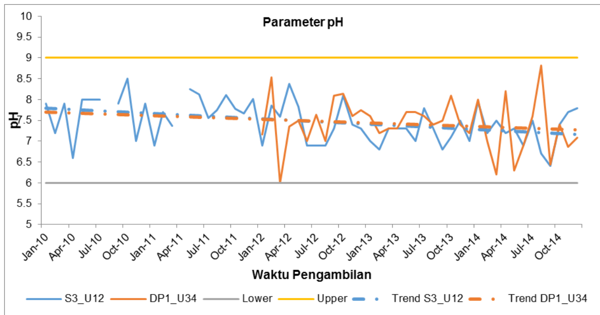
Gambar 2.21. Profil pH pada PLTU Tanjung Jati B Unit 1&2 dan PLTU Tanjung Jati B Unit 3&4
