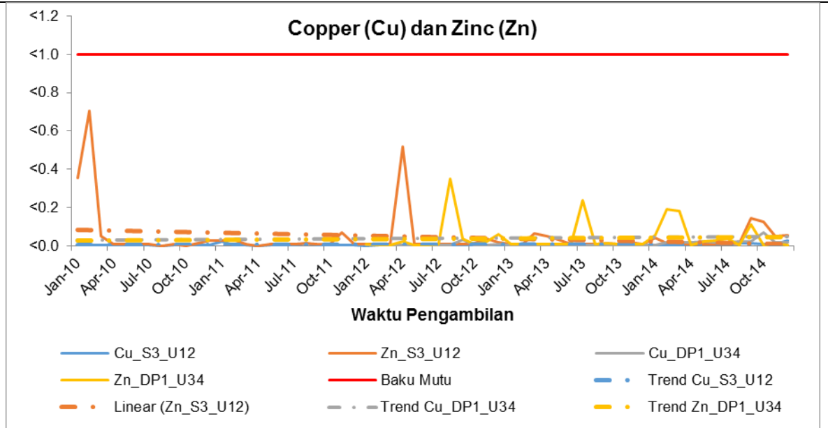
Gambar 2.25. Profil Cu dan Zn pada PLTU Tanjung Jati B Unit 1&2 dan PLTU Tanjung Jati B Unit 3&4 (sumber: hasil pemantauan PLTU Tanjung Jati B Unit 1&2 dan PLTU Tanjung Jati B Unit 3&4, 2010 – 2014)
