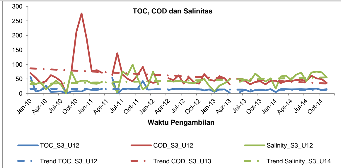
Gambar 2.27. Profil TOC, COD dan Salinitas pada PLTU Tanjung Jati B Unit 1&2 (sumber: hasil pemantauan PLTU Tanjung Jati B Unit 1&2, 2010 – 2014)
