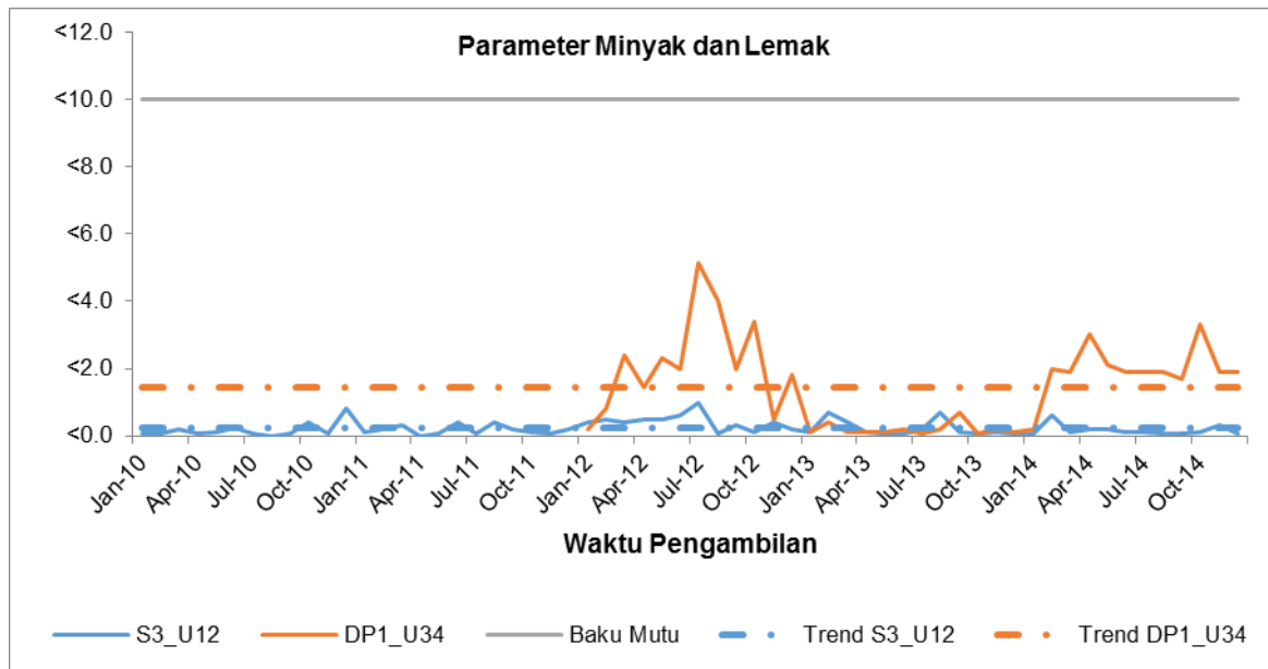
Gambar 2.26. Profil Minyak dan Lemak pada PLTU Tanjung Jati B Unit 1&2 dan PLTU Tanjung Jati B Unit 3&4 (sumber: hasil pemantauan PLTU Tanjung Jati B Unit 1&2 dan PLTU Tanjung Jati B Unit 3&4, 2010 – 2014)
