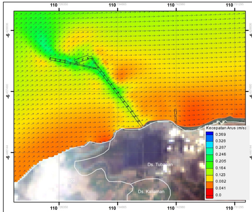
Gambar 2.103. Hasil permodelan arus musim peralihan 1 zona 2 kondisi eksisting (pasang menuju surut) (Sumber : Hasil Pemodelan, September 2015)
