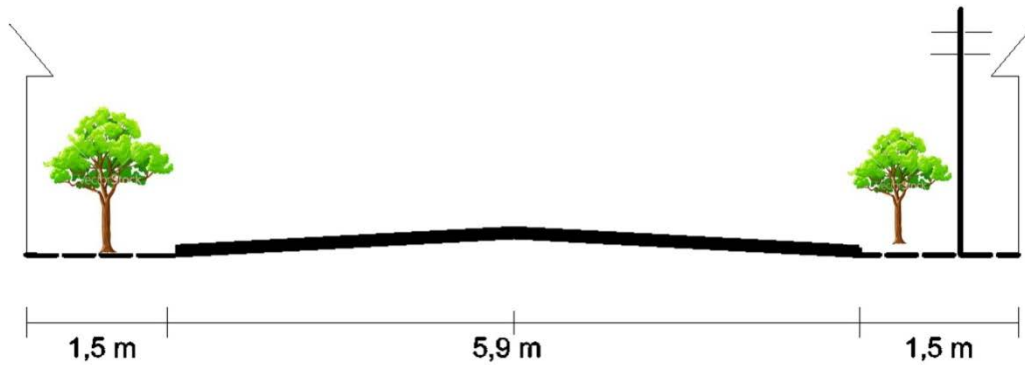
Gambar 2.149. Potongan Melintang Ruas Jalan Lokal Wedelan – Tubanan (Jalan Akses PLTU) Sumber : Survei Lapangan, 2015
