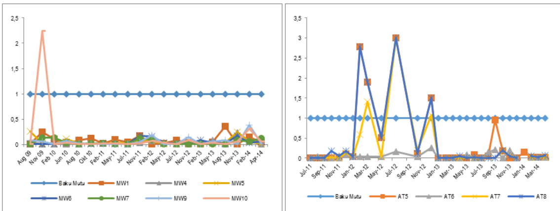
Gambar 2.36. Grafik Kualitas Air Tanah parameter Fe hasil pemantauan Unit 1&2 (kiri) dan Unit 3&4 (kanan) (sumber: Hasil pemantauan Unit 1-4, 2010-2014)
