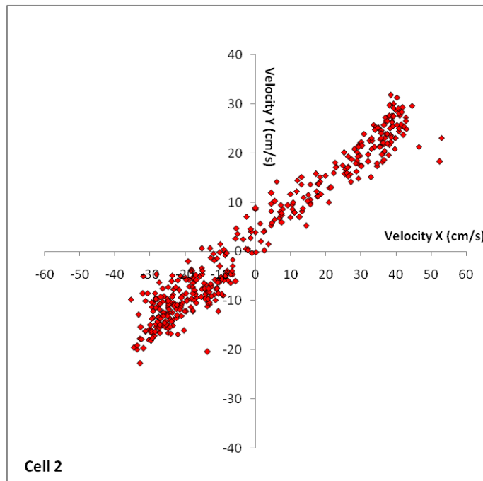
Gambar 2.90. Scatter plot kecepatan arus kedalaman 7,2 - 9 meter ( layer 2 ) di Perairan Tanjung Jati, Jepara Tanggal 29 Oktober - 1 November 2015 (Sumber : Analisis Data, November 2015)
