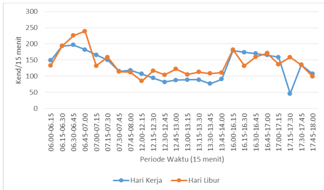
Gambar 2.151. Perbandingan Volume Lalu lintas pada Hari Kerja dan hari Libur di Ruas Jalan Lokal Wedelan – Tubanan (Jalan Akses PLTU) Sumber : Data Primer, 2015
