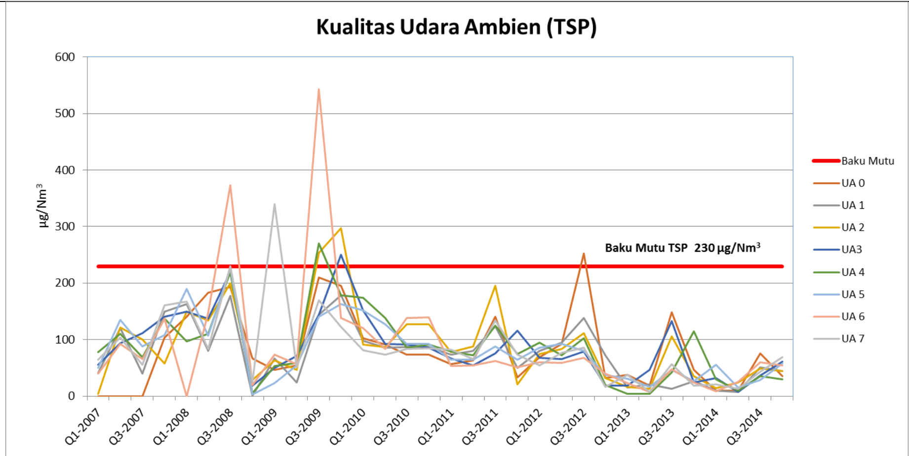
Gambar 2.8. Gambar Profil kualitas udara ambien (TSP) PLTU Tanjung Jati B Unit 1&2 (sumber: Hasil Pemantauan PLTU Tanjung Jati B Unit 1&2, 2007-2014)
