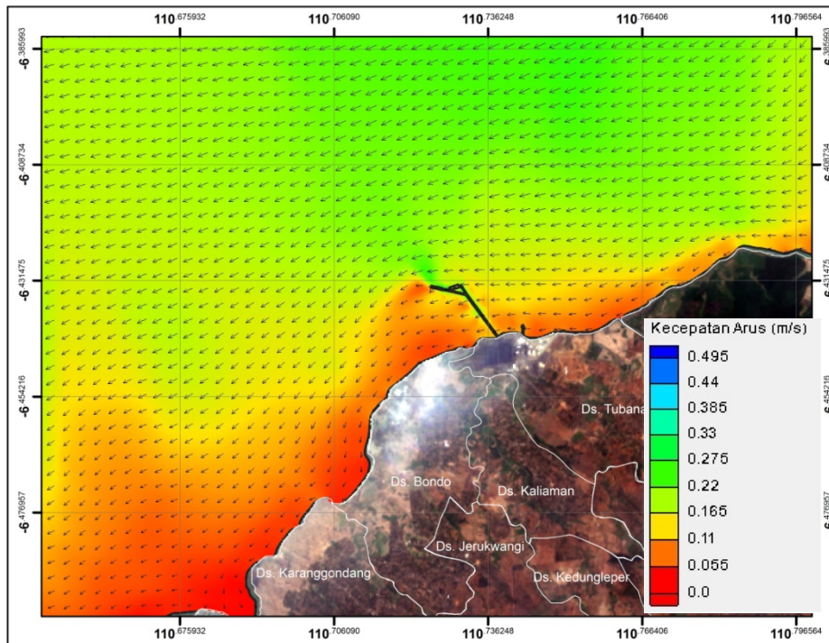
Gambar 2.98. Hasil permodelan arus musim barat zona 1 kondisi eksisting (surut menuju pasang) (Sumber: Hasil Pemodelan, September 2015)
