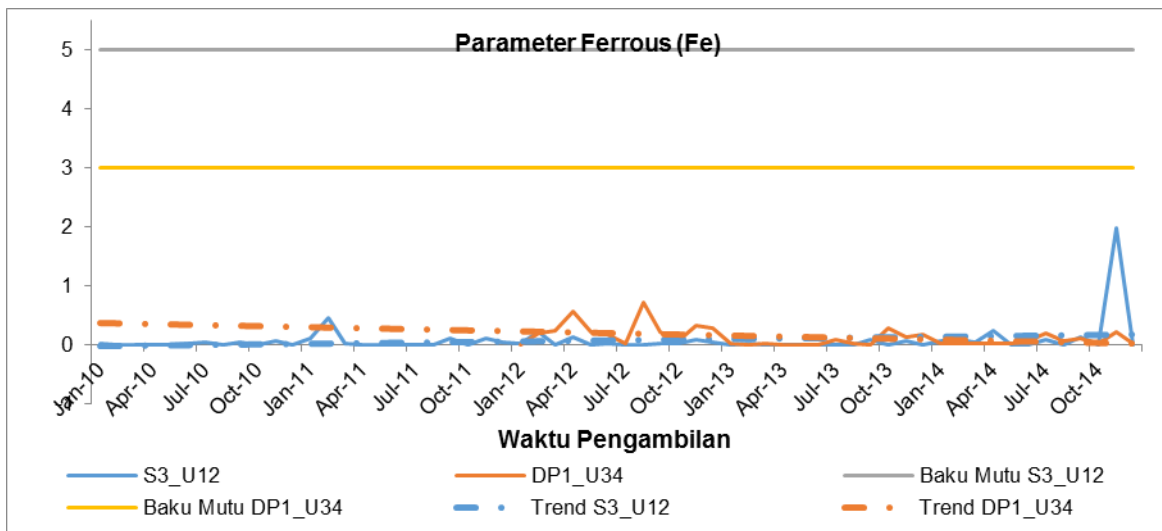
Gambar 2.23. Profil Fe pada PLTU Tanjung Jati B Unit 1&2 dan PLTU Tanjung Jati B Unit 3&4 (sumber: hasil pemantauan Unit 1&2 dan Unit 3&4, 2010 – 2014)
