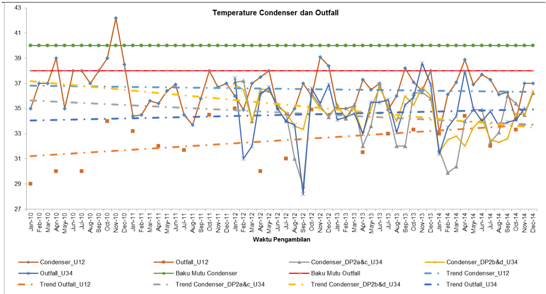
Gambar 2.29. Profil Temperatur di kondensor dan Outfall PLTU Tanjung Jati B Unit 1&2 dan PLTU Tanjung Jati B Unit 3&4 (sumber: hasil pemantauan PLTU Tanjung Jati B Unit 1-4, 2010 – 2014)
