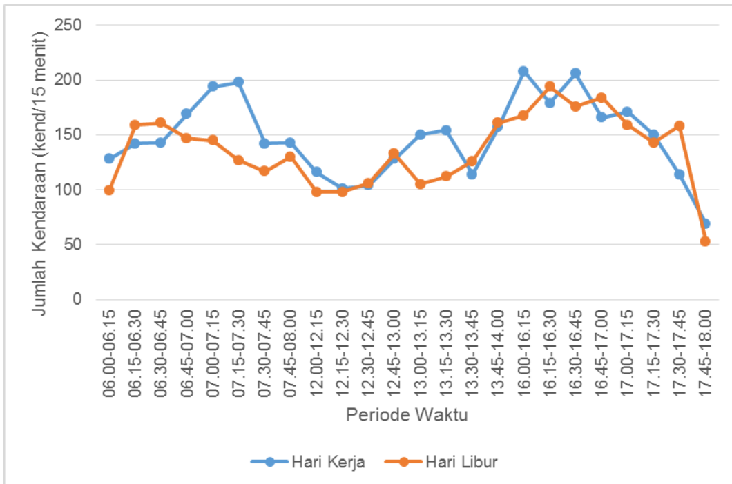
Gambar 2.160. Fluktuasi Arus Lalu lintas di Simpang 4 Tak Bersinyal Kaliaman (Sumber: Survei Lapangan, 2015)
