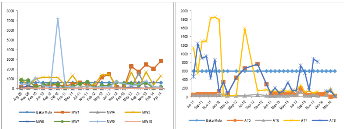
Gambar 2.37. Grafik kualitas air tanah parameter Cl hasil pemantauan Unit 1&2 (kiri) dan Unit 3&4 (kanan) (sumber: Hasil pemantauan Unit 1-4, 2010-2014)
