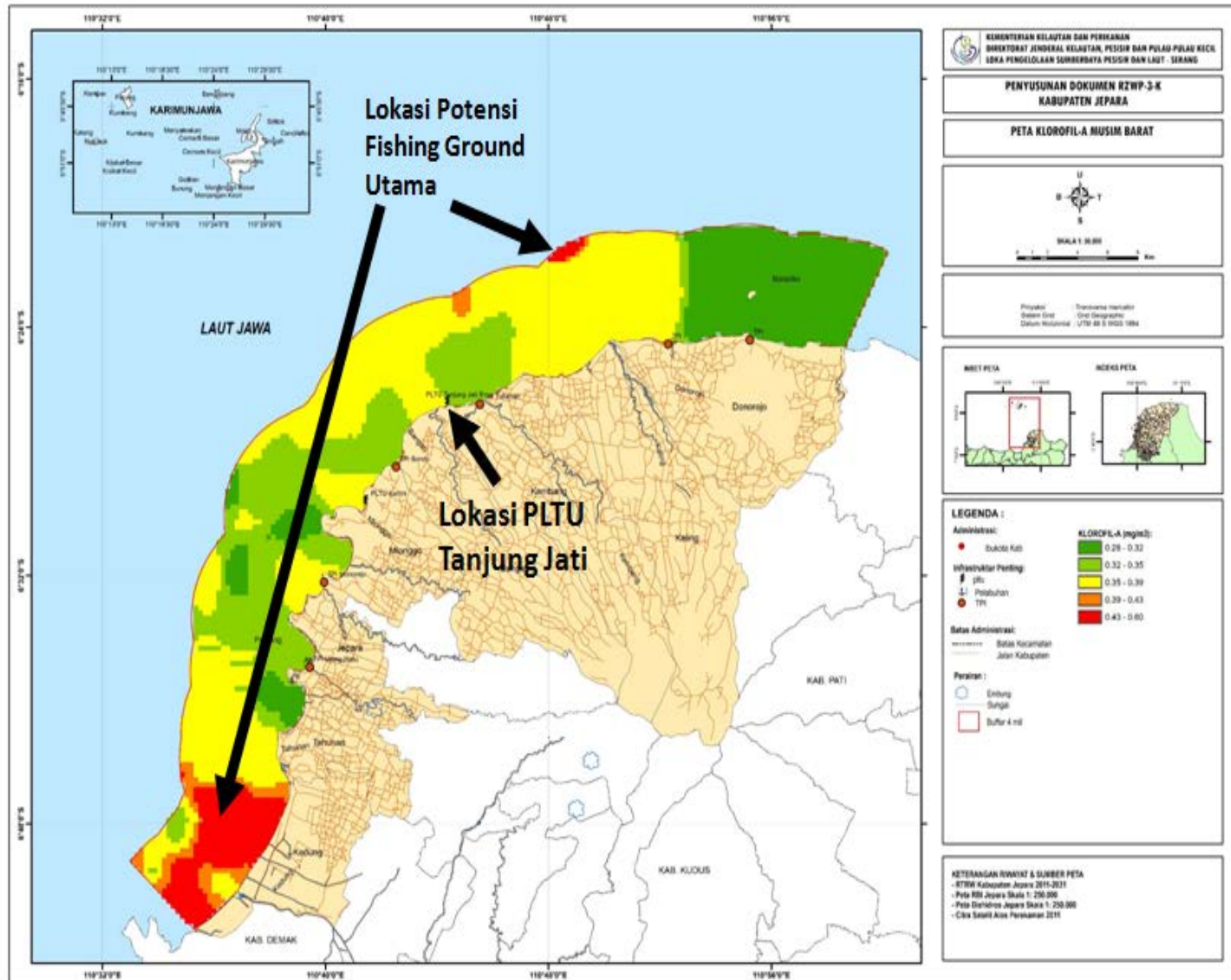
Gambar 2.168. Peta Klorofil A Perairan Kabupaten Jepara Pada Musim Barat
