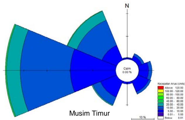
Gambar 2.68. Kondisi arus (currentrose) musim timur tahun 2007-2014 (Sumber data: BMKG-SMM Semarang, 2007-2014)
