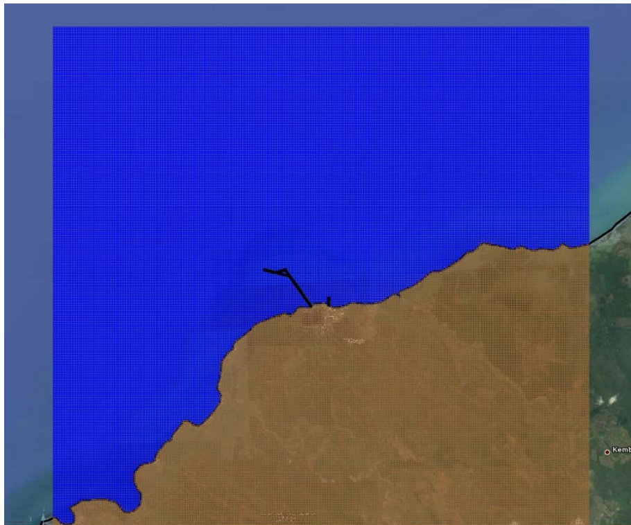
Gambar 2.55. Grid permodelan gelombang kondisi eksisting (Sumber : Hasil Pemodelan, September 2015)
