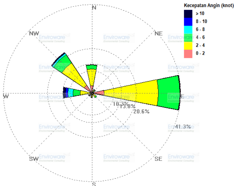
Gambar 2.4. Windrose tahun 2005 - 2014 di wilayah studi (BMKG, 2014)
