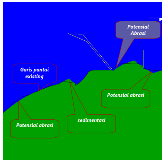
Gambar 2.122. Hasil Model Musim Barat Perubahan Garis Pantai di Perairan Tanjung Jati, Jepara, Kondisi Eksisting Tahun Ketiga
