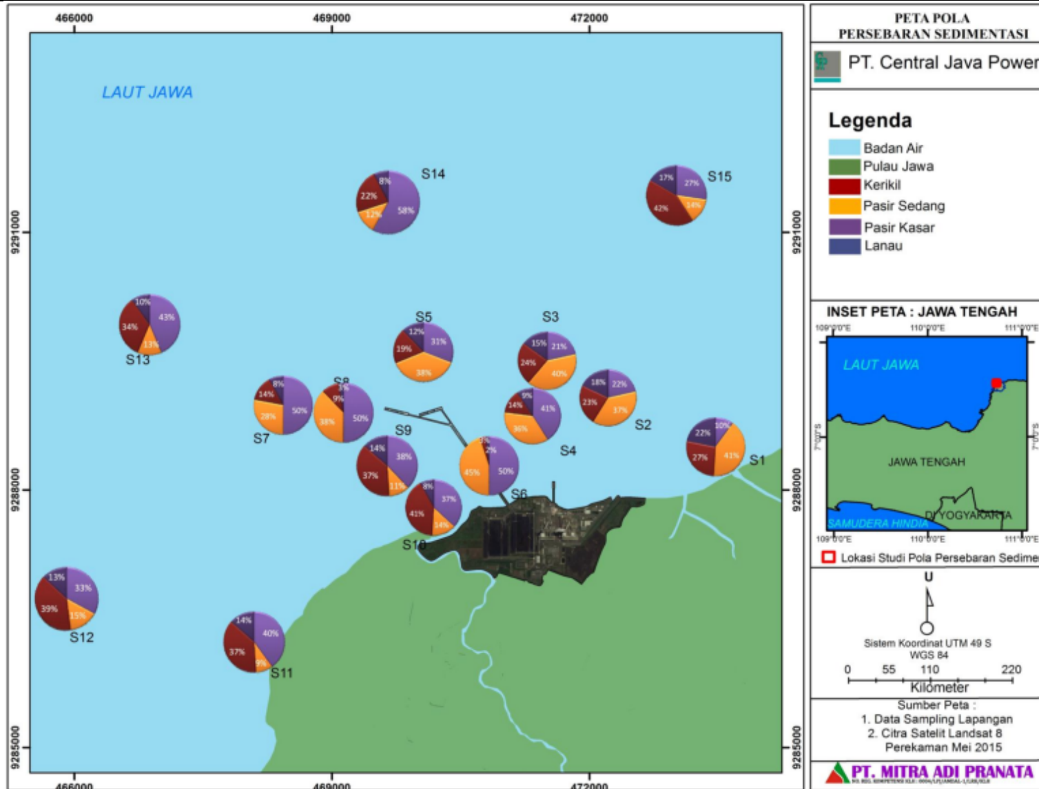
Gambar 2.147. Peta Persebaran Sedimen di Perairan Tanjung Jati Jepara
