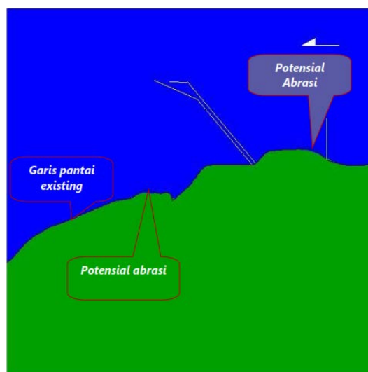
Gambar 2.141. Hasil Model Musim Peralihan 2 Perubahan Garis Pantai di Perairan Tanjung Jati, Jepara, Kondisi Eksisting Tahun Pertama
