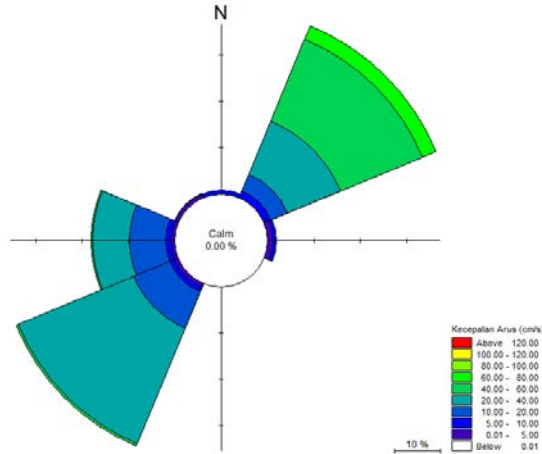
Gambar 2.86. Current rose kedalaman 1,8 – 3,6 meter ( layer 5 ) di Perairan Tanjung Jati, Jepara Tanggal 29 Oktober - 1 November 2015 (Sumber: Analisis Data, November 2015)
