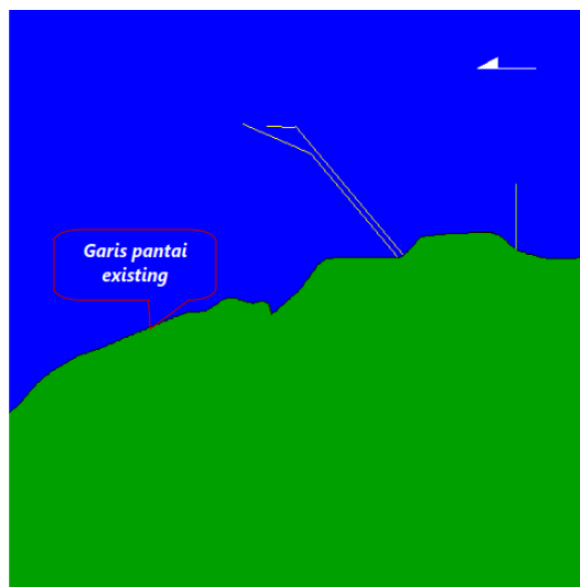
Gambar 2.133. Hasil Model Musim Timur Perubahan Garis Pantai di Perairan Tanjung Jati, Jepara, Kondisi Eksisting
