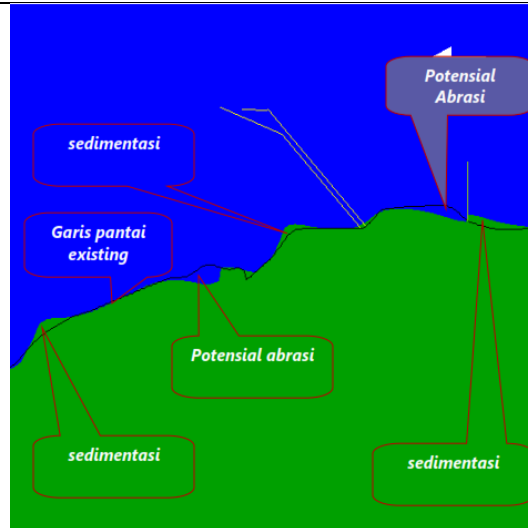
Gambar 2.129. Hasil Model Musim Peralihan 1 Perubahan Garis Pantai di Perairan Tanjung Jati, Jepara, Kondisi Eksisting Tahun Ketiga
