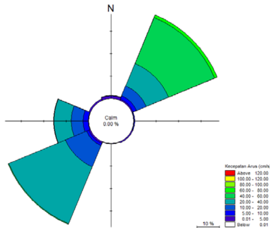
Gambar 2.85. Current rose kedalaman 3,6 – 5,4 meter ( layer 4 ) di Perairan Tanjung Jati, Jepara Tanggal 29 Oktober - 1 November 2015 (Sumber: Analisis Data, November 2015)
