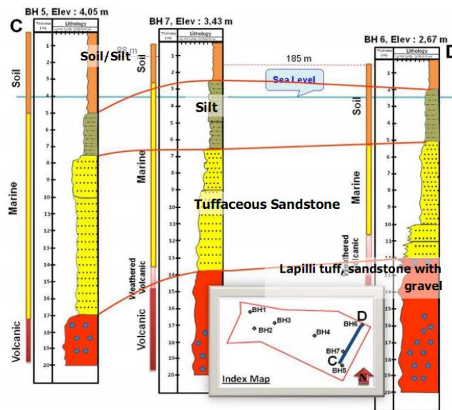
Gambar 2.19. Penampang C-D, menunjukkan korelasi borehole berarah Utara-Selatan.
