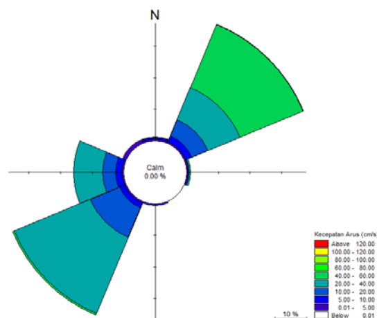
Gambar 2.84. Current rose kedalaman 5,4 – 7,2 meter ( layer 3 ) di Perairan Tanjung Jati, Jepara Tanggal 29 Oktober - 1 November 2015 (Sumber: Analisis Data, November 2015)
