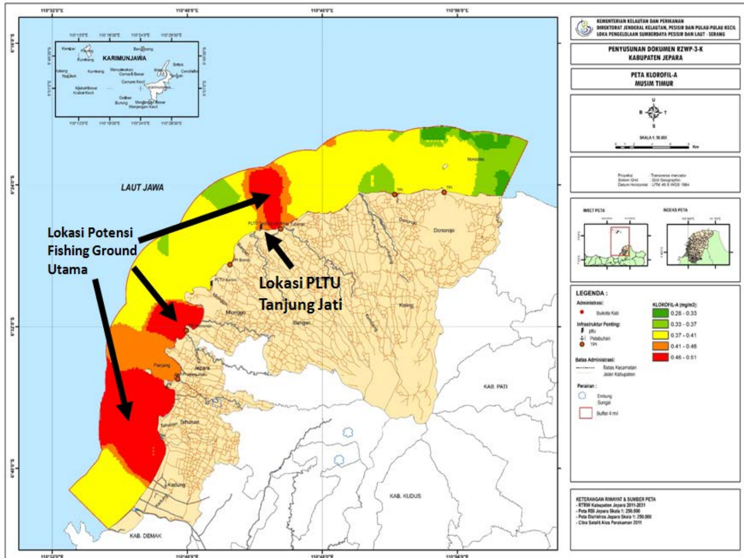
Gambar 2.166. Peta Klorofil A Perairan Kabupaten Jepara Pada Musim Timur
