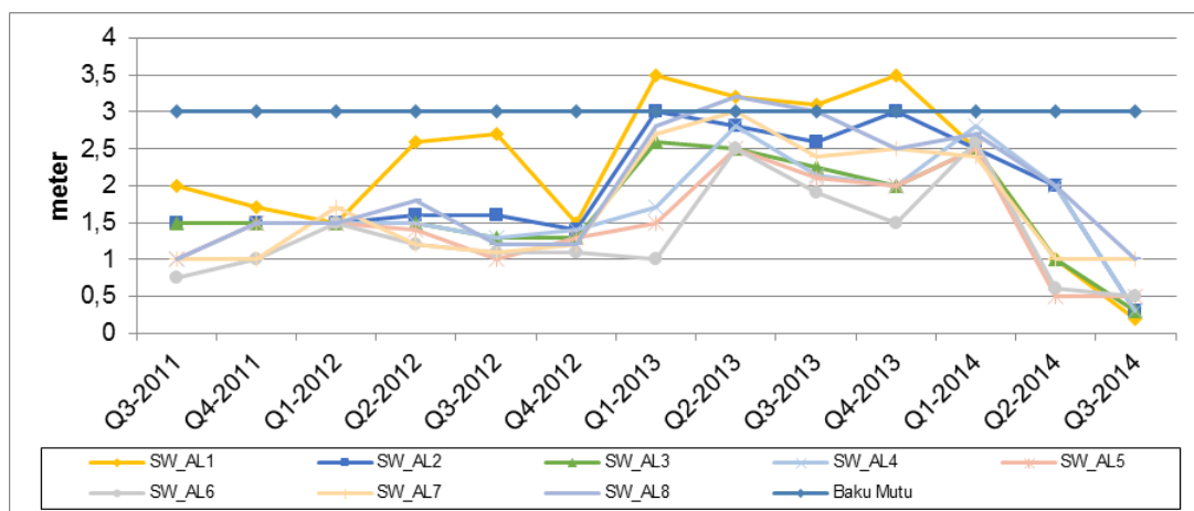
Gambar 2.30. Kualitas air laut ( Brightness ) pemantauan PLTU Tanjung Jati B Unit 3&4 tahun 2011-2014 (sumber: Hasil pemantauan PLTU Tanjung Jati B Unit 1-4, 2010-2014)
