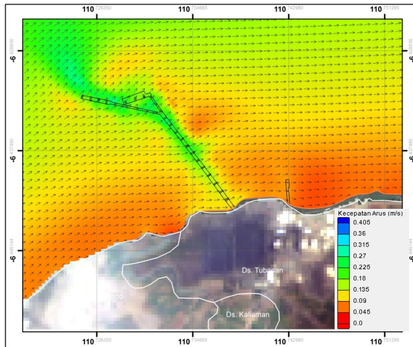
Gambar 2.111. Hasil permodelan arus musim peralihan 2 zona 2 kondisi eksisting (pasang menuju surut) (Sumber : Hasil Pemodelan, September 2015)
