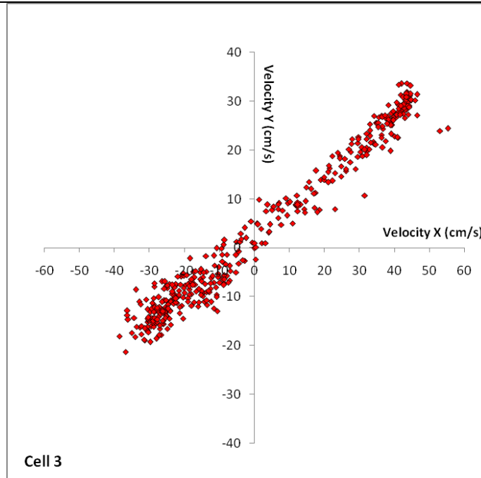
Gambar 2.91. Scatter plot kecepatan arus kedalaman 5,4 – 7,2 meter ( layer 3 ) di Perairan Tanjung Jati, Jepara Tanggal 29 Oktober - 1 November 2015 (Sumber : Analisis Data, November 2015)
