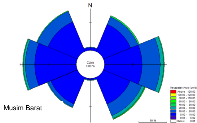
Gambar 2.67. Kondisi arus (currentrose) musim barat tahun 2007-2014 (Sumber data: BMKG-SMM Semarang, 2007-2014)
