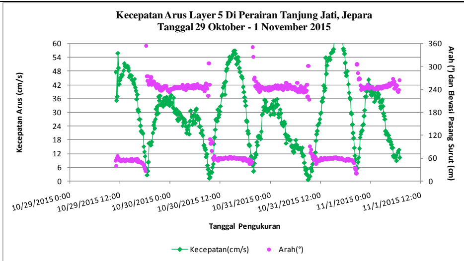
Gambar 2.79. Kecepatan arus kedalaman 1,8 - 3,6 meter ( layer 5 ) di Perairan Tanjung Jati, Jepara Tanggal 29 Oktober - 1 November 2015 (Sumber: Analisis Data, November 2015)
