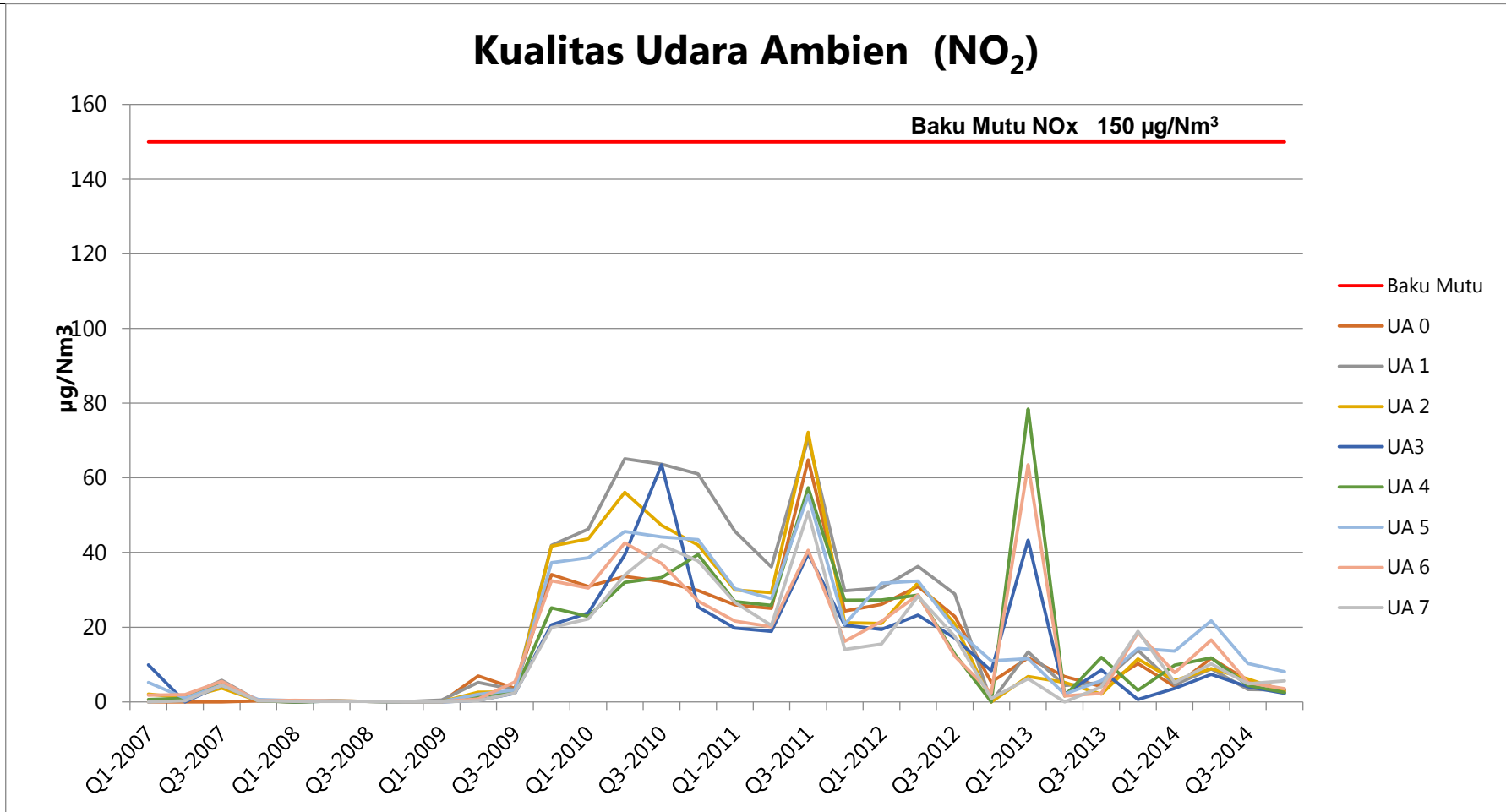
Gambar 2.12. Profil kualitas udara ambien (NO 2 ) PLTU Tanjung Jati B Unit 1&2 Sumber: Hasil Pemantauan PLTU Tanjung Jati B Unit 1&2, 2007-2014 yang dimodifikasi
