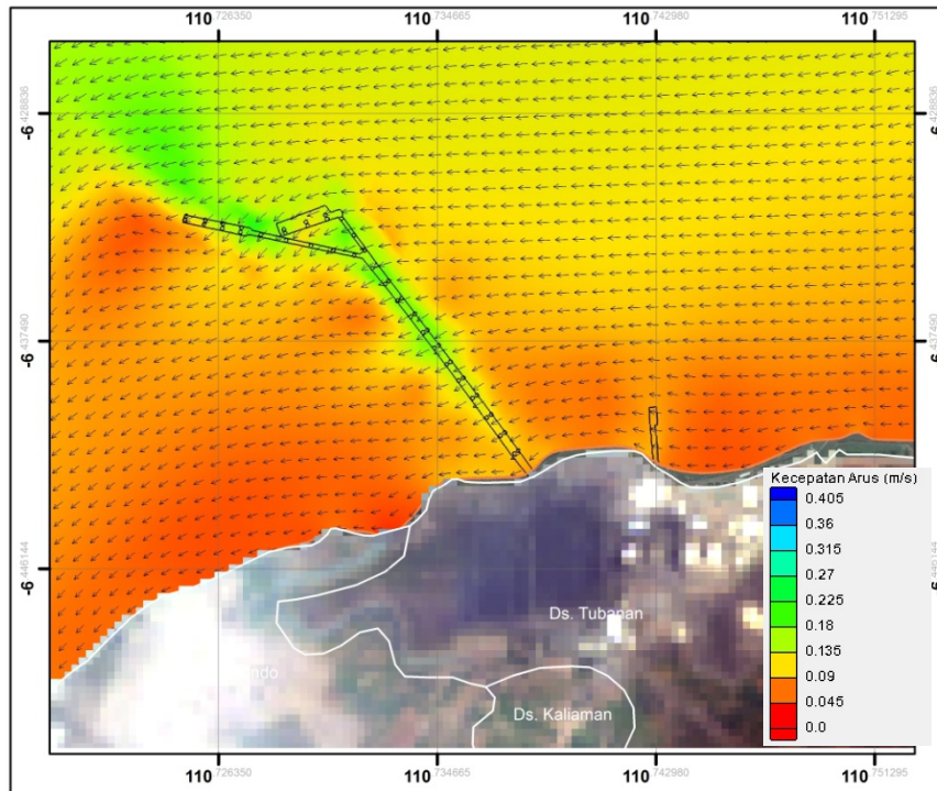
Gambar 2.112. Hasil permodelan arus musim peralihan 2 zona 2 kondisi eksisting (surut menuju pasang) (Sumber : Hasil Pemodelan, September 2015)
