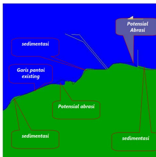
Gambar 2.144. Hasil Model Musim Peralihan 2 Perubahan Garis Pantai di Perairan Tanjung Jati, Jepara, Kondisi Eksisting Tahun Keempat
