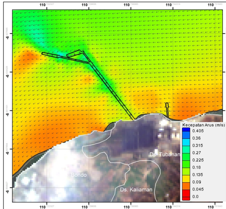
Gambar 2.108. Hasil permodelan arus musim timur zona 2 kondisi eksisting (surut menuju pasang) (Sumber: Hasil Permodelan, September 2015)
