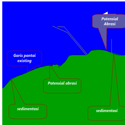
Gambar 2.135. Hasil Model Musim Timur Perubahan Garis Pantai di Perairan Tanjung Jati, Jepara, Kondisi Eksisting Tahun Kedua
