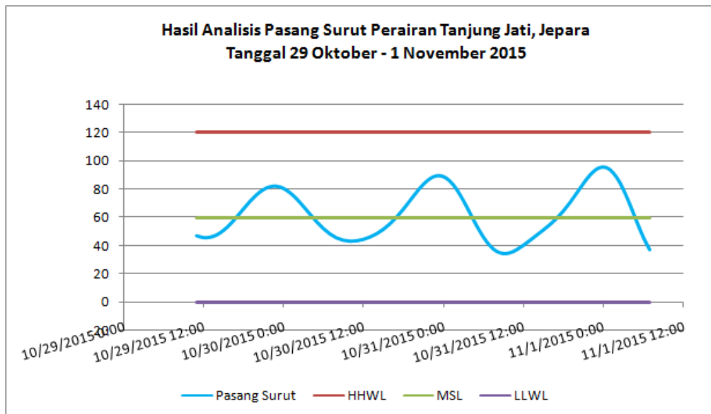
Gambar 2.66. Grafik hasil analisis pasang surut di Perairan Tanjung Jati tanggal 29 Oktober-1 November 2015, Jepara (Sumber : Analisis Data, November 2015)
