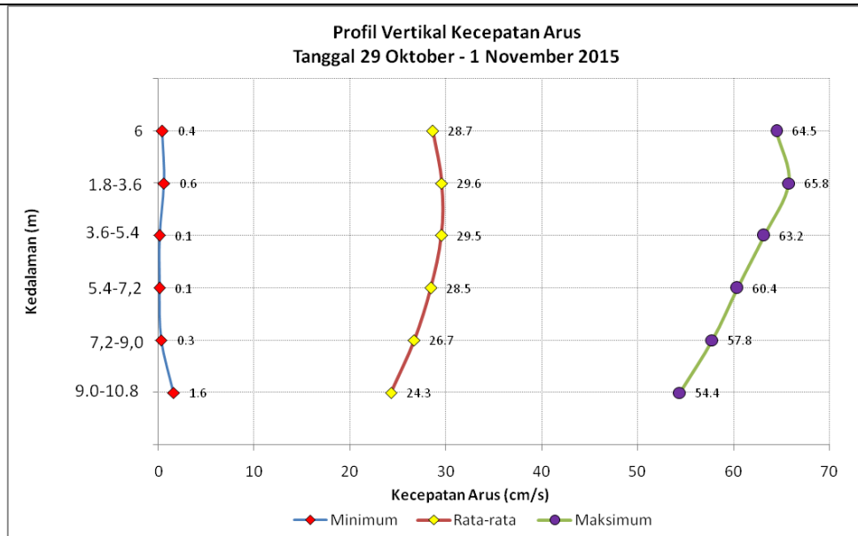
Gambar 2.73. Profil Vertikal Kecepatan Arus di Perairan Tanjung Jati, Jepara Tanggal 29 Oktober - 1 November 2015 (Sumber : Analisis Data, November 2015)
