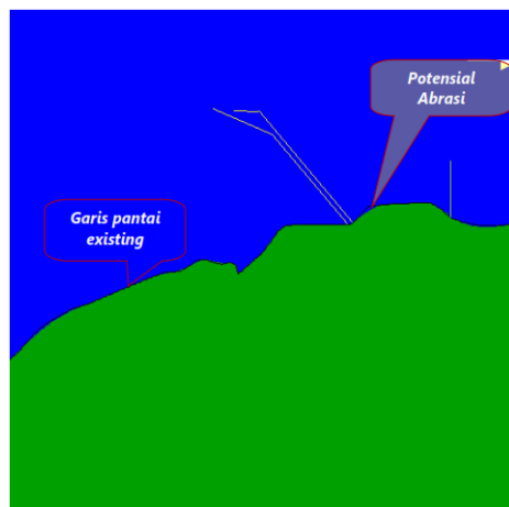
Gambar 2.120. Hasil Model Musim Barat Perubahan Garis Pantai di Perairan Tanjung Jati, Jepara, Kondisi Eksisting Tahun Pertama
