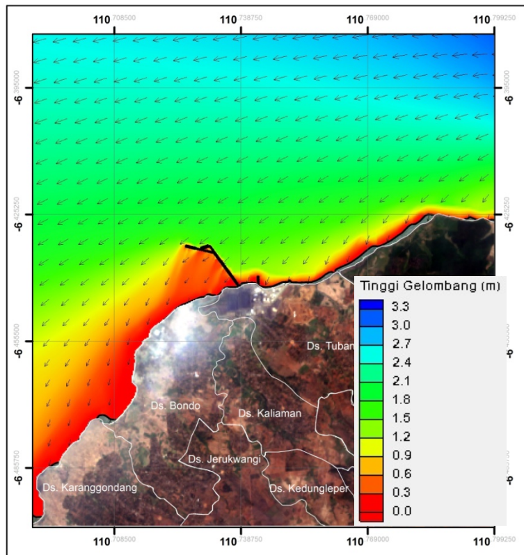
Gambar 2.63. Hasil permodelan gelombang zona 1 pada musim peralihan 2 kondisi eksisting (Sumber : Hasil Pemodelan, September 2015)
