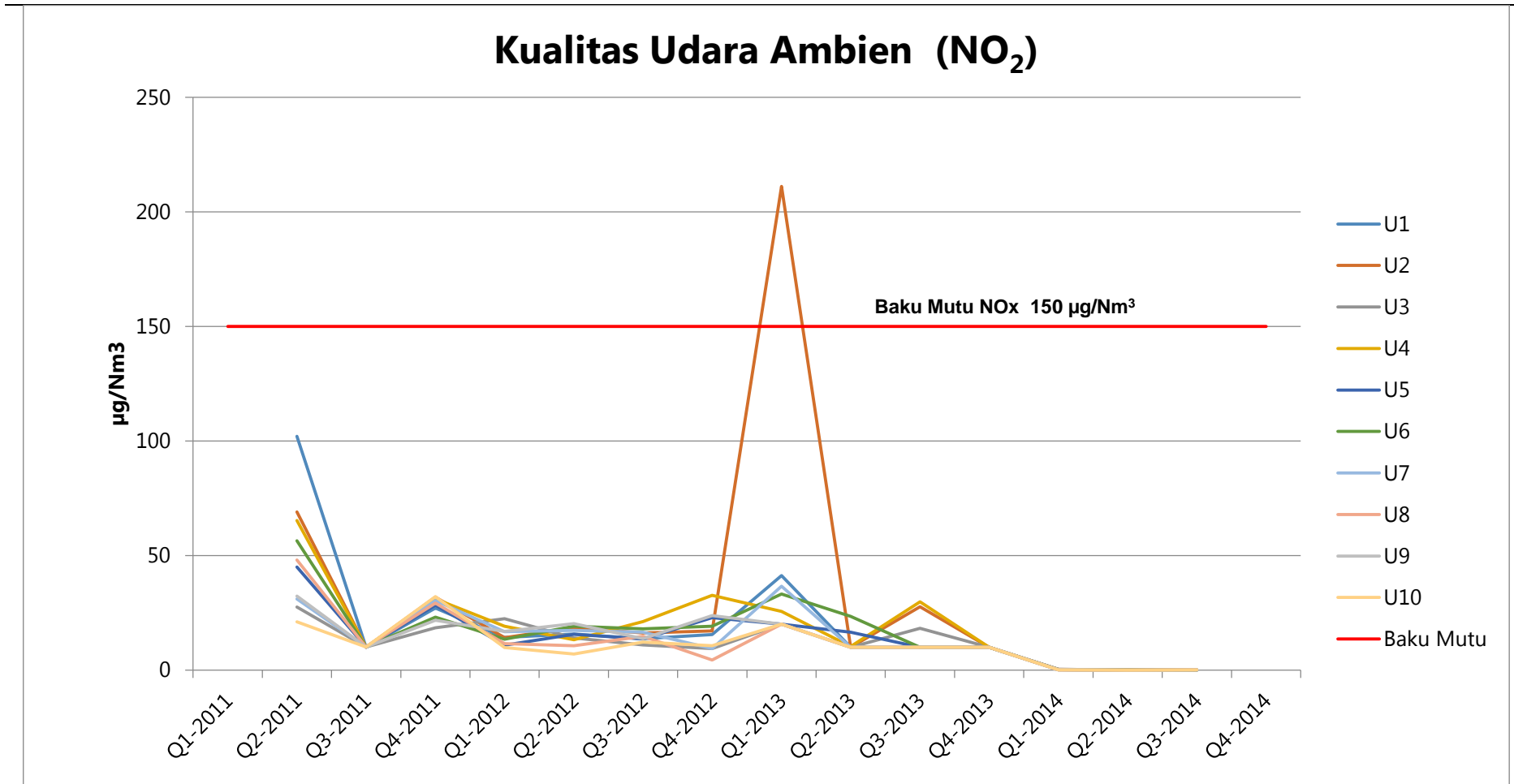
Gambar 2.13. Profil kualitas udara ambien (NO 2 ) PLTU Tanjung Jati B Unit 3&4 (sumber: Hasil Pemantauan PLTU Tanjung Jati B Unit 3&4, 2011-2014)
