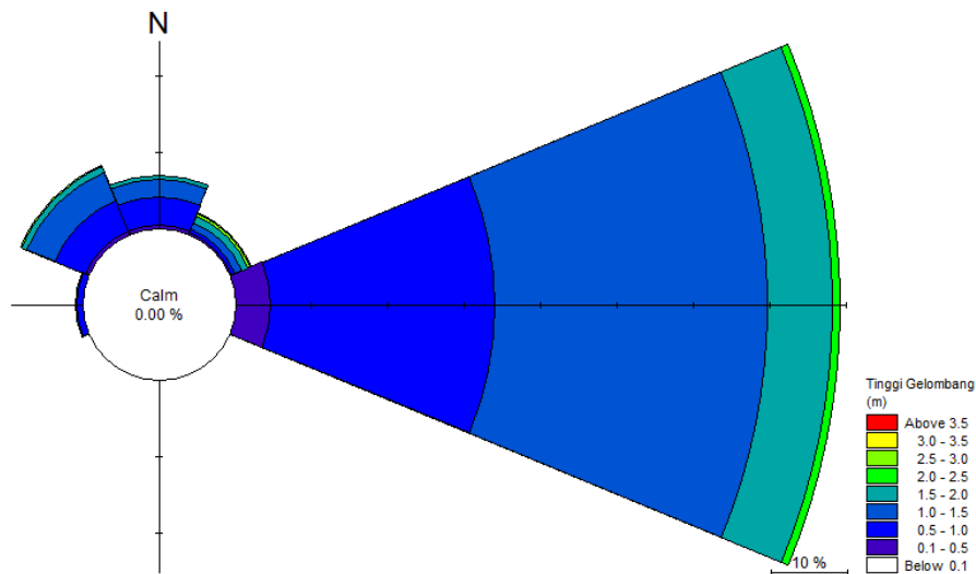
Gambar 2.49. Kondisi gelombang ( waverose ) musim timur tahun 2005-2014 (Sumber data: BMKG-SMM Semarang, 2005-2014)
