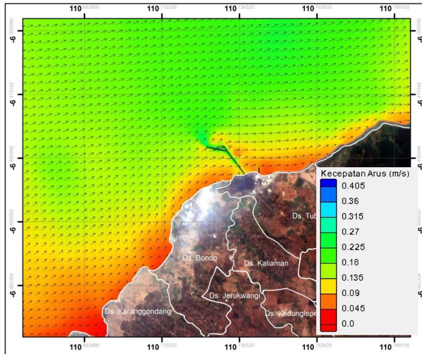
Gambar 2.109. Hasil permodelan arus musim peralihan 2 zona 1 kondisi eksisting (pasang menuju surut) (Sumber : Hasil Pemodelan, September 2015)
