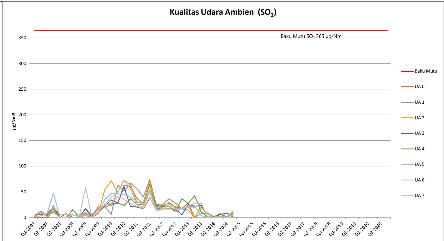
Gambar 2.10. Profil kualitas udara ambien (SO 2 ) PLTU Tanjung Jati B Unit 1&2 (sumber: Hasil Pemantauan PLTU Tanjung Jati B Unit 1&2, 2007-2014)
