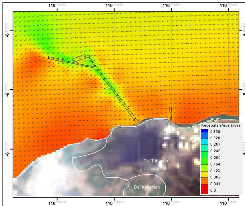
Gambar 2.104. Hasil permodelan arus musim peralihan 1 zona 2 kondisi eksisting (surut menuju pasang) (Sumber : Hasil Pemodelan, September 2015)
