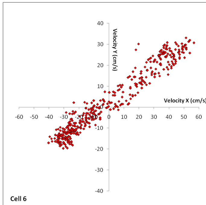
Gambar 2.94. Scatter plot kecepatan arus kedalaman 0 – 1,8 meter ( layer 6 ) di Perairan Tanjung Jati, Jepara Tanggal 29 Oktober - 1 November 2015 (Sumber : Analisis Data, November 2015)
