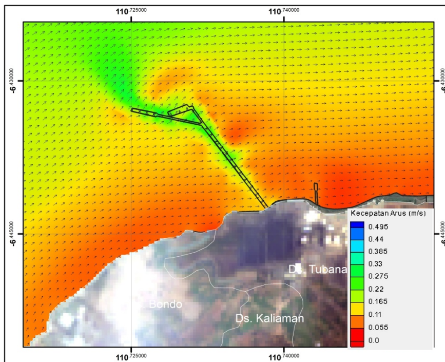
Gambar 2.100. Hasil permodelan arus musim barat zona 2 kondisi eksisting (surut menuju pasang) (Sumber: Hasil Pemodelan, September 2015)
