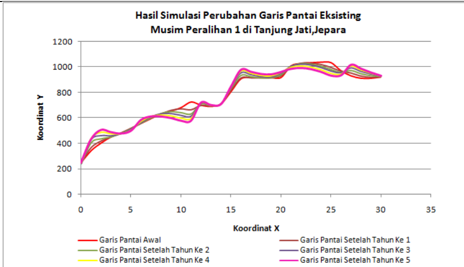
Gambar 2.132. Hasil Simulasi Perubahan Garis Pantai Eksisting Musim Peralihan 1 di Perairan Tanjung Jati, Jepara
