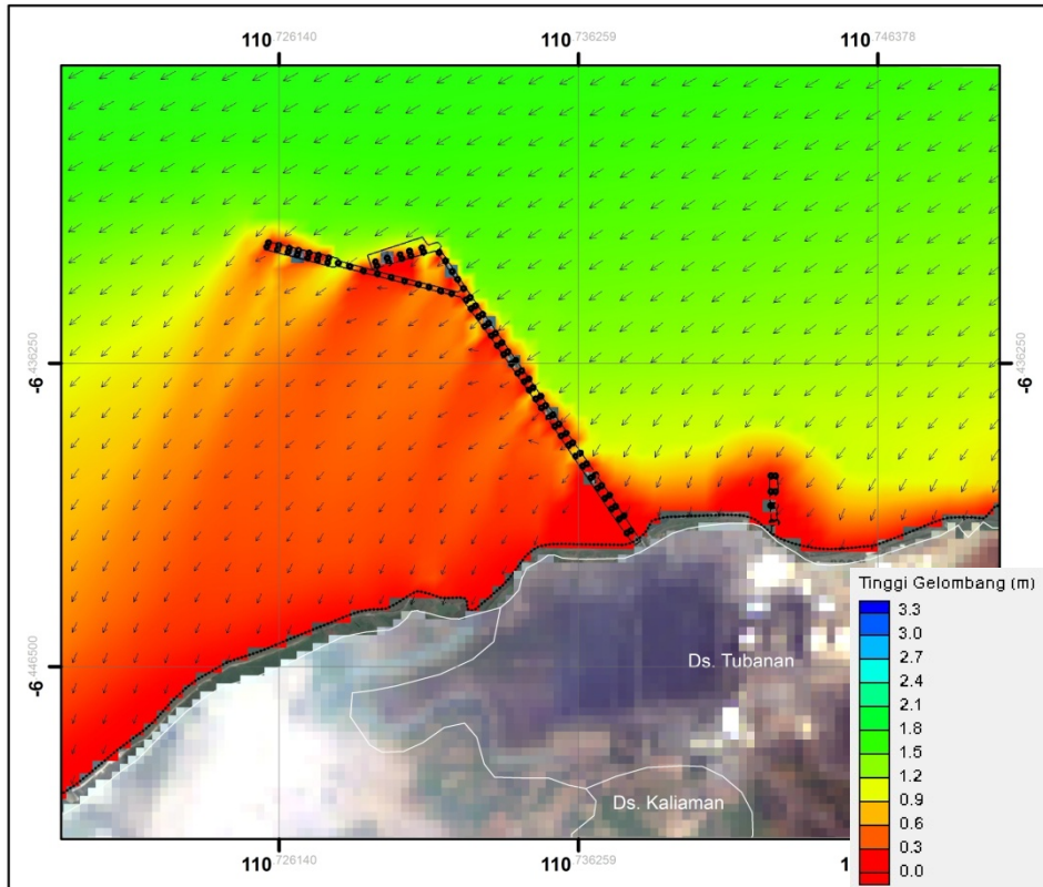
Gambar 2.62. Hasil permodelan gelombang zona 2 pada musim timur kondisi eksisting (Sumber : Hasil Pemodelan, September 2015)
