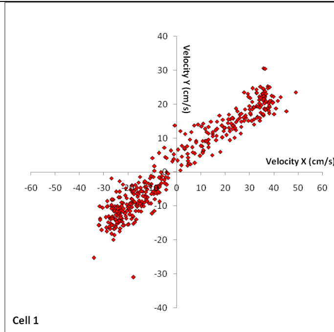
Gambar 2.89. Scatter plot kecepatan arus kedalaman 9 - 10,8 meter ( layer 1 ) di Perairan Tanjung Jati, Jepara Tanggal 29 Oktober - 1 November 2015 (Sumber : Analisis Data, November 2015)
