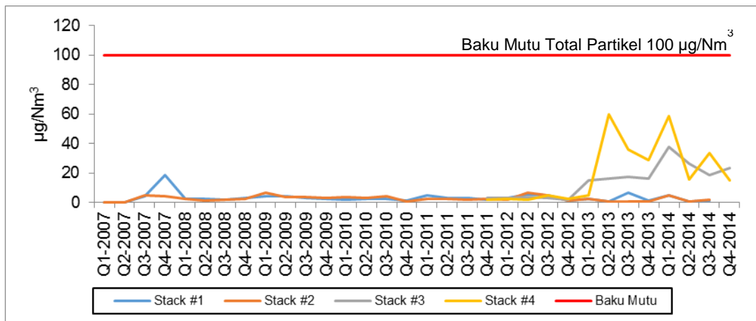
Gambar 2.7. Emisi Total Partikel di Cerobong PLTU Tanjung Jati B Unit 1-4 Tahun 2007-2014 (Sumber: hasil pemantauan PLTU Tanjung Jati B Unit 1-4, 2007-2014)
