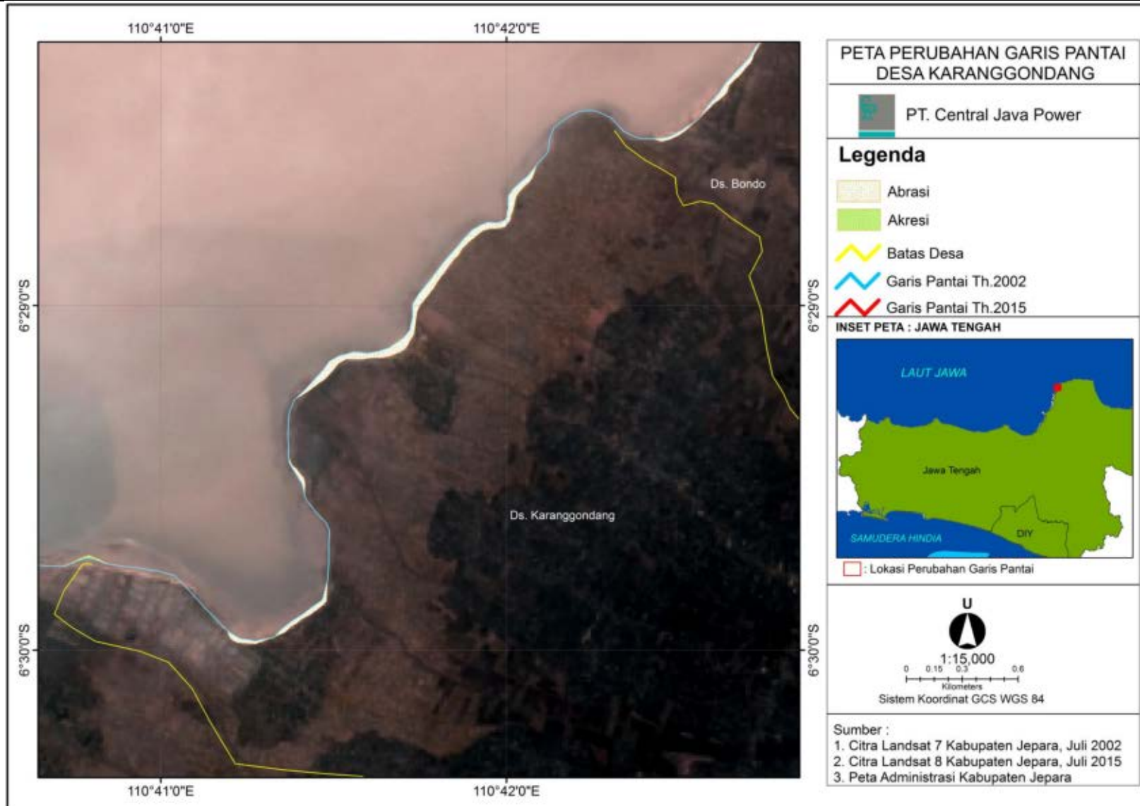
Gambar 2.114. Perubahan Garis Pantai di Desa Karanggondang Jepara pada Perode Tahun 2002-2015
