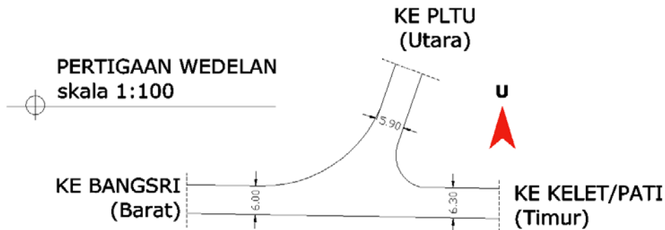
Gambar 2.152. Geometri Simpang 3 Tak Bersinyal Wedelan (Sumber: Survei Lapangan, 2015)
