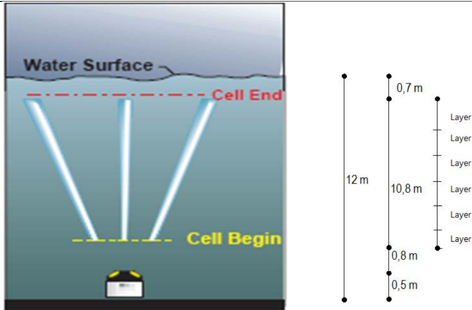
Gambar 2.71. Ilustrasi Pengukuran (Perekaman Data) Kecepatan dan Arah Arus menggunakan ADCP Argonaut XR (Sumber : User's Manual, Sontek Argonaut XR )
