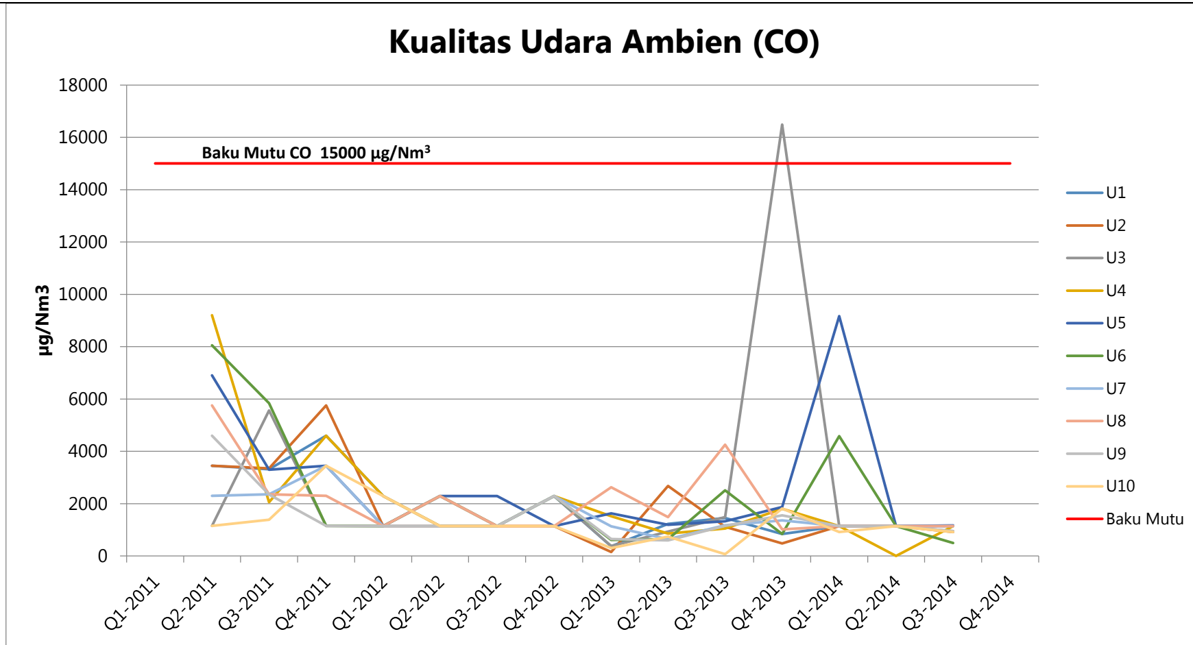
Gambar 2.15. Profil kualitas udara ambien (CO) PLTU Tanjung Jati B Unit 3&4 (sumber: Hasil Pemantauan PLTU Tanjung Jati B Unit 3&4, 2011-2014 Yang dimodifikasi)
