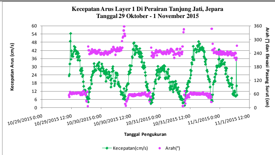
Gambar 2.75. Kecepatan arus kedalaman 9 - 10,8 meter ( layer 1 ) di Perairan Tanjung Jati, Jepara Tanggal 29 Oktober - 1 November 2015 (Sumber: Analisis Data, November 2015)
