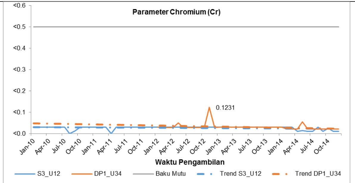
Gambar 2.24. Profil Cr pada PLTU Tanjung Jati B Unit 1&2 dan PLTU Tanjung Jati B Unit 3&4 (sumber: hasil pemantauan PLTU Tanjung Jati B Unit 1&2 dan PLTU Tanjung Jati B Unit 3&4, 2010 – 2014)
