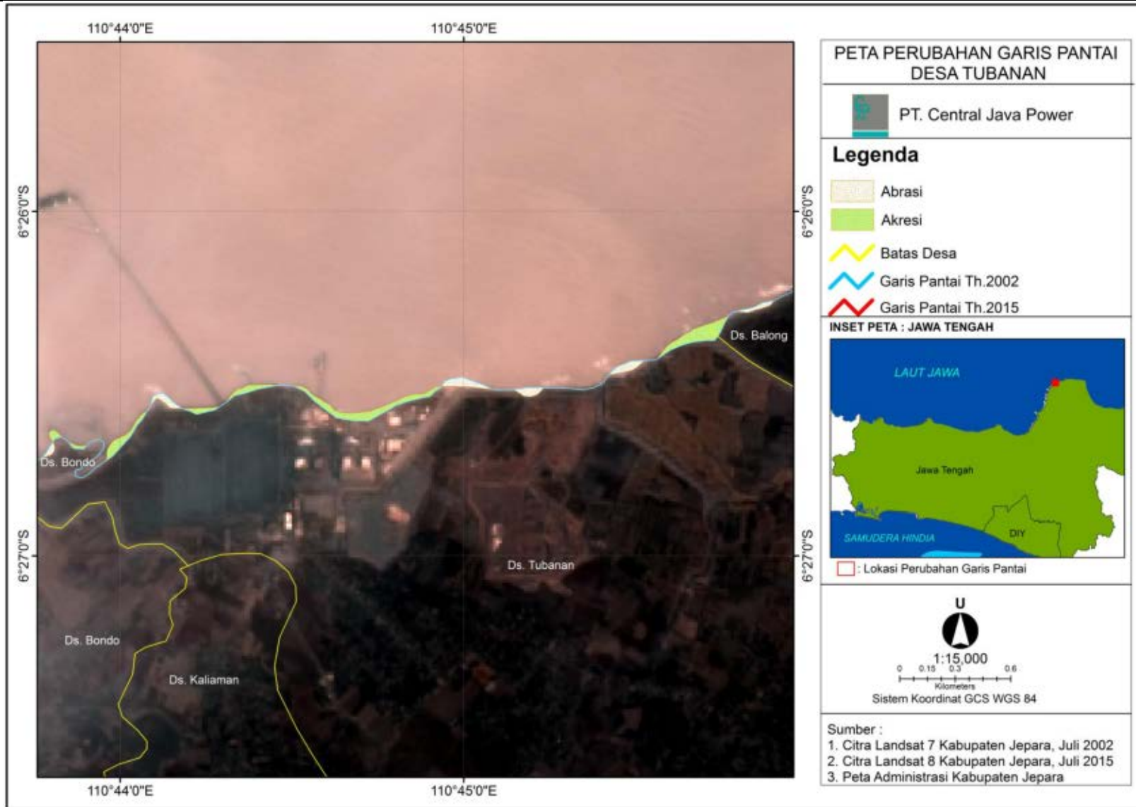
Gambar 2.116. Perubahan Garis Pantai di Desa Tubanan Jepara pada Perode Tahun 2002-2015
