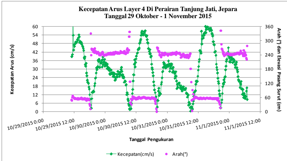
Gambar 2.78. Kecepatan arus kedalaman 3,6 - 5,4 meter ( layer 4 ) di Perairan Tanjung Jati, Jepara Tanggal 29 Oktober - 1 November 2015 (Sumber: Analisis Data, November 2015)
