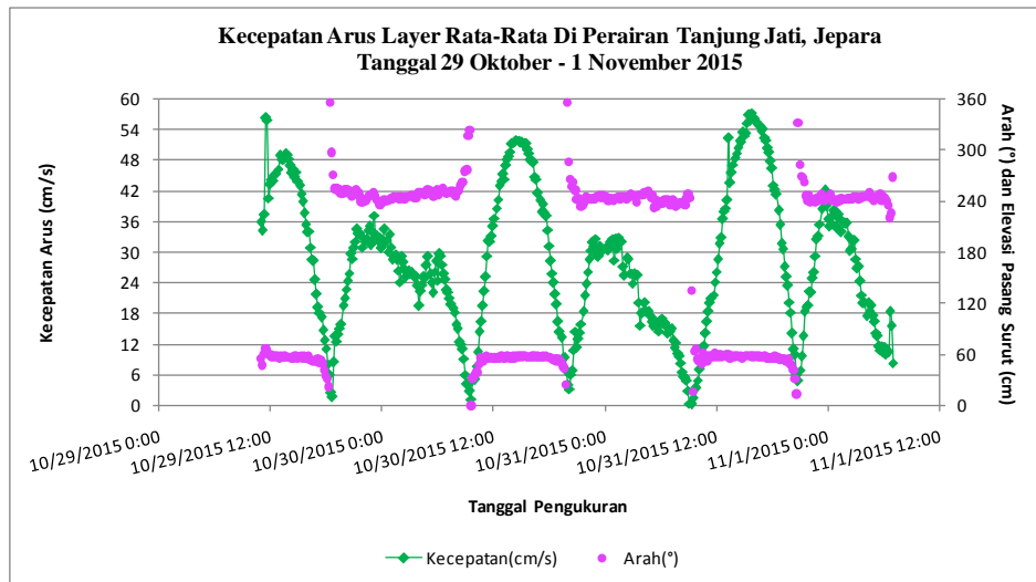
Gambar 2.74. Kecepatan arus kedalaman rata-rata di Perairan Tanjung Jati, Jepara Tanggal 29 Oktober - 1 November 2015 (Sumber: Analisis Data, November 2015)
