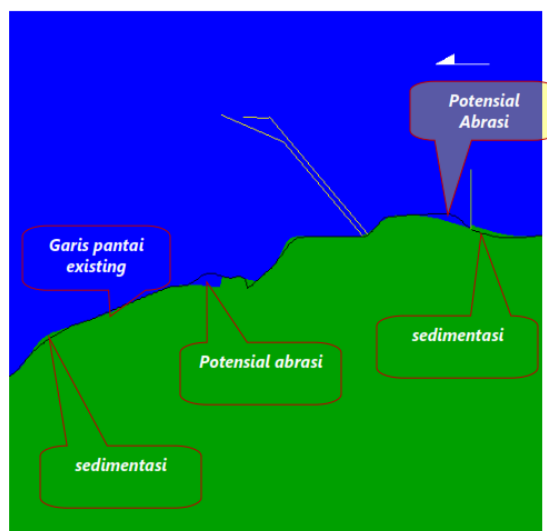
Gambar 2.136. Hasil Model Musim Timur Perubahan Garis Pantai di Perairan Tanjung Jati, Jepara, Kondisi Eksisting Tahun Ketiga
