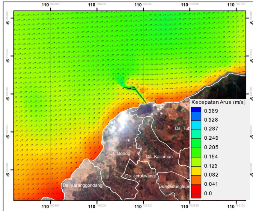
Gambar 2.101. Hasil permodelan arus musim peralihan 1 zona 1 kondisi eksisting (pasang menuju surut) (Sumber : Hasil Pemodelan, September 2015)
