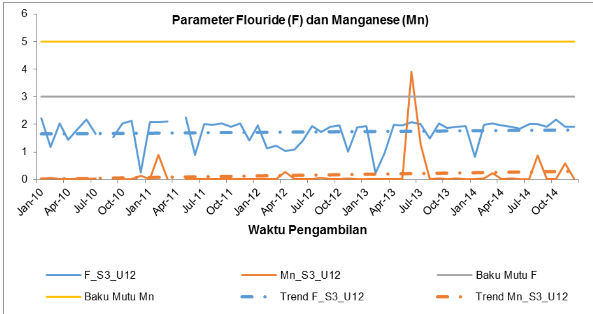
Gambar 2.22. Profil F dan Mn pada PLTU Tanjung Jati B Unit 1&2 (sumber: hasil pemantauan PLTU Tanjung Jati B Unit 1&2, 2010 – 2014)
