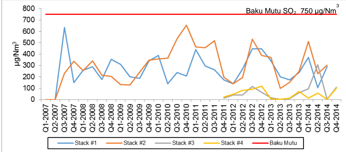
Gambar 2.5. Emisi SO 2 di Cerobong PLTU Tanjung Jati B Unit 1-4 Tahun 2007 - 2014 (Sumber: hasil pemantauan PLTU Tanjung Jati B Unit 1-4, 2007 - 2014)
