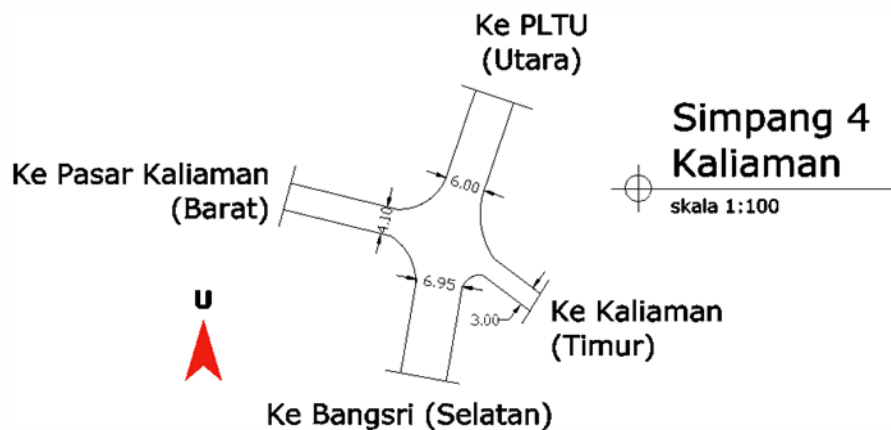
Gambar 2.158. Geometri Simpang 4 Tak Bersinyal Kaliaman (Sumber: Survei Lapangan, 2015)
