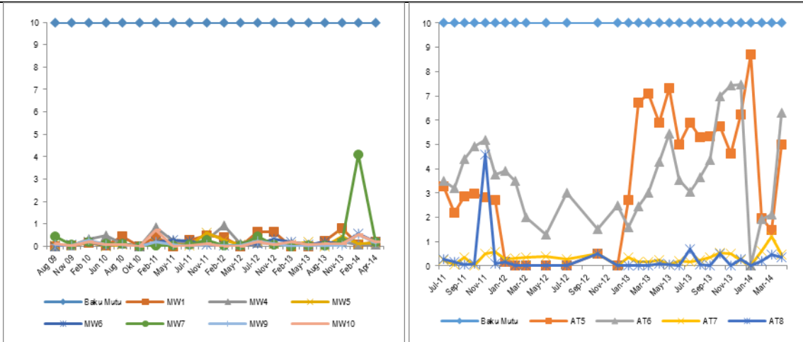
Gambar 2.41. Grafik kualitas air tanah parameter Nitrat hasil pemantauan Unit 1&2 (kiri) dan Unit 3&4 (kanan)(sumber: Hasil pemantauan Unit 1-4, 2010-2014)
