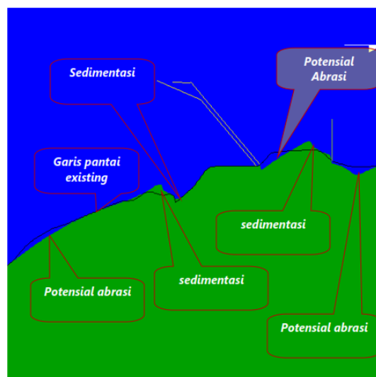
Gambar 2.123. Hasil Model Musim Barat Perubahan Garis Pantai di Perairan Tanjung Jati, Jepara, Kondisi Eksisting Tahun Keempat
