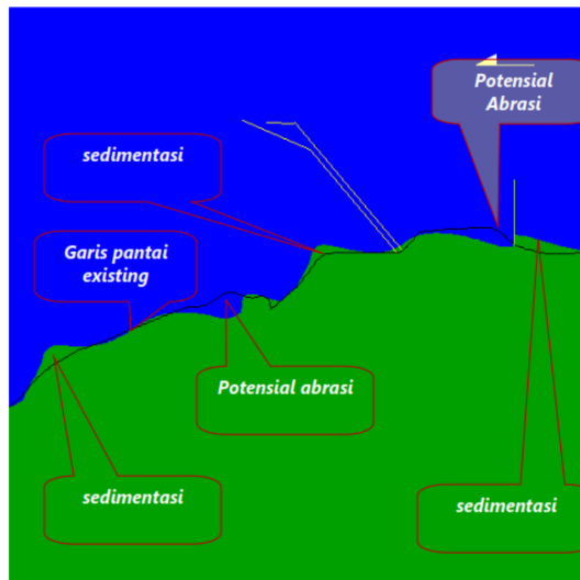
Gambar 2.130. Hasil Model Musim Peralihan 1 Perubahan Garis Pantai di Perairan Tanjung Jati, Jepara, Kondisi Eksisting Tahun Keempat
