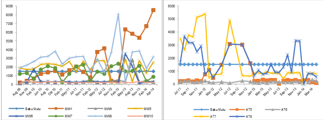
Gambar 2.35. Grafik kualitas air tanah parameter TDS hasil pemantauan Unit 1&2 (kiri) dan Unit 3&4 (kanan) (sumber: Hasil pemantauan Unit 1-4, 2010-2014)
