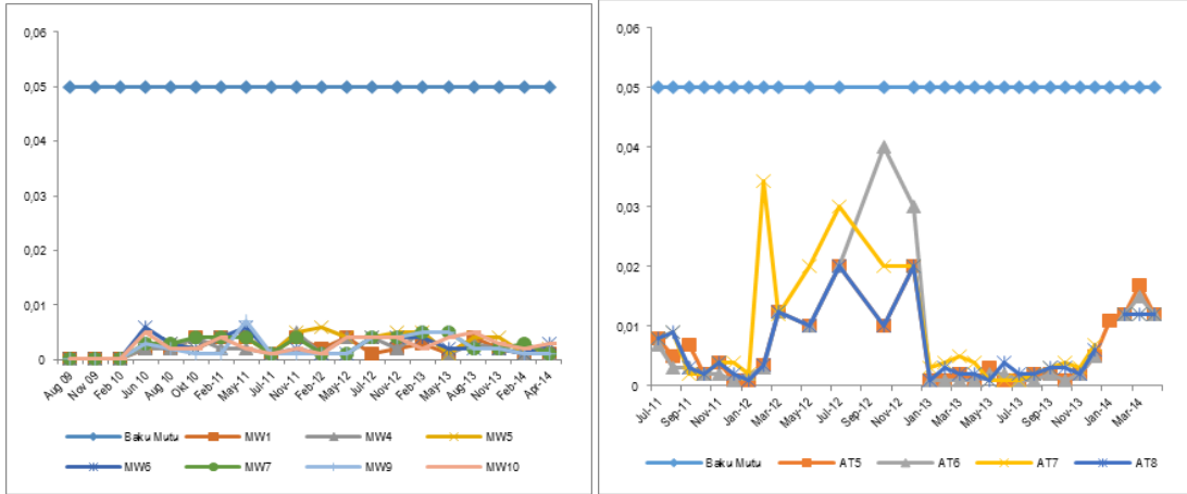
Gambar 2.38. Grafik kualitas air tanah parameter Cr^{6+} hasil pemantauan Unit 1&2 (kiri) dan Unit 3&4 (kanan) (sumber: Hasil pemantauan Unit 1-4, 2010-2014)
