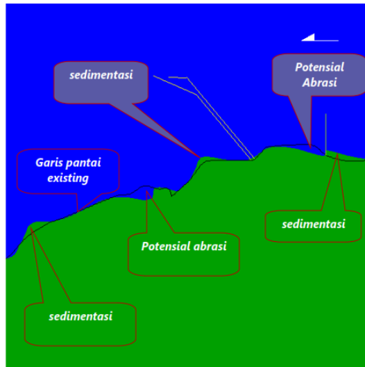
Gambar 2.138. Hasil Model Musim Timur Perubahan Garis Pantai di Perairan Tanjung Jati, Jepara, Kondisi Eksisting Tahun Kelima
