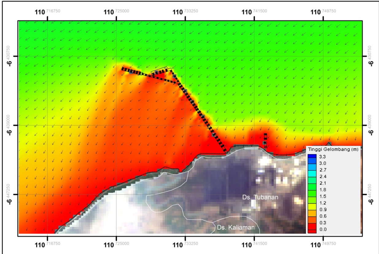
Gambar 2.64. Hasil permodelan gelombang zona 2 pada musim peralihan 2 kondisi eksisting (Sumber : Hasil Pemodelan, September 2015)
