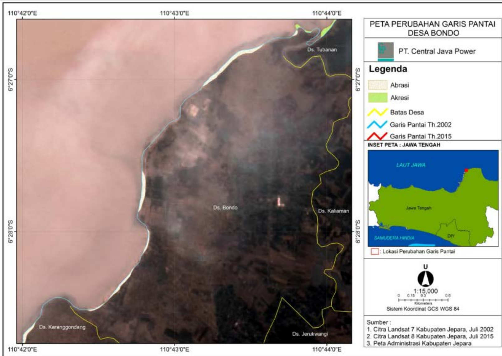
Gambar 2.115. Perubahan Garis Pantai di Desa Bondo Jepara pada Perode Tahun 2002-2015
