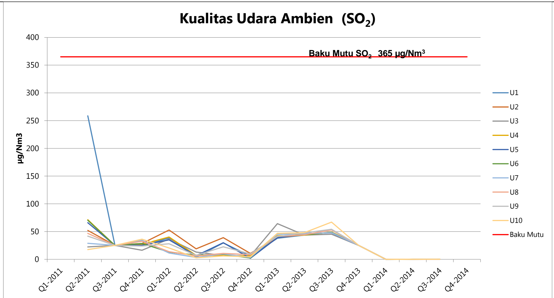
Gambar 2.11. Profil kualitas udara ambien (SO 2 ) PLTU Tanjung Jati B Unit 3&4 Sumber: Hasil Pemantauan PLTU Tanjung Jati B Unit 3&4, 2011-2014 yang dimodifikasi
