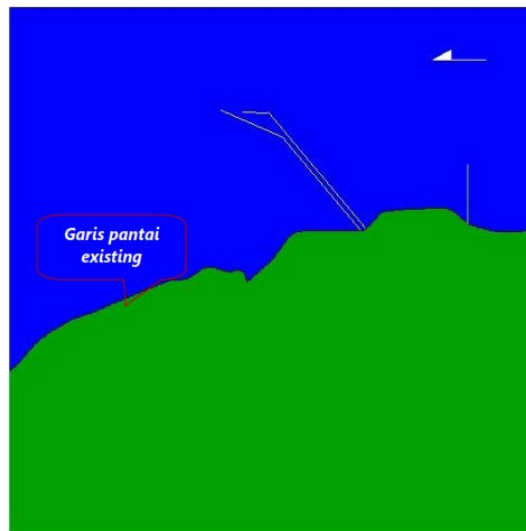
Gambar 2.140. Hasil Model Musim Peralihan 2 Perubahan Garis Pantai di Perairan Tanjung Jati, Jepara, Kondisi Eksisting
