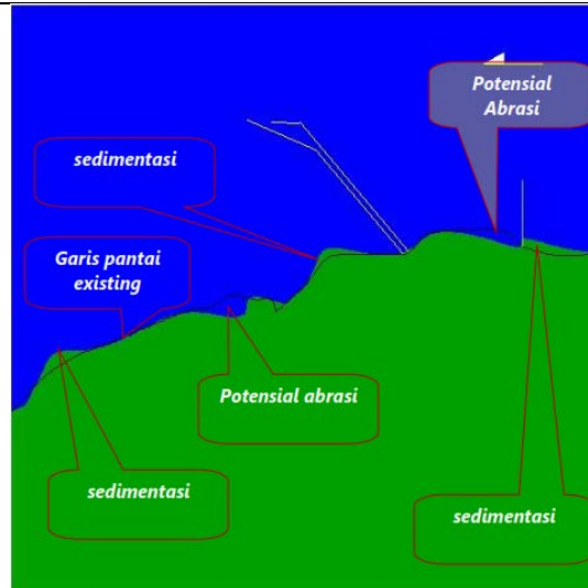
Gambar 2.145. Hasil Model Musim Peralihan 2 Perubahan Garis Pantai di Perairan Tanjung Jati, Jepara, Kondisi Eksisting Tahun Kelima
