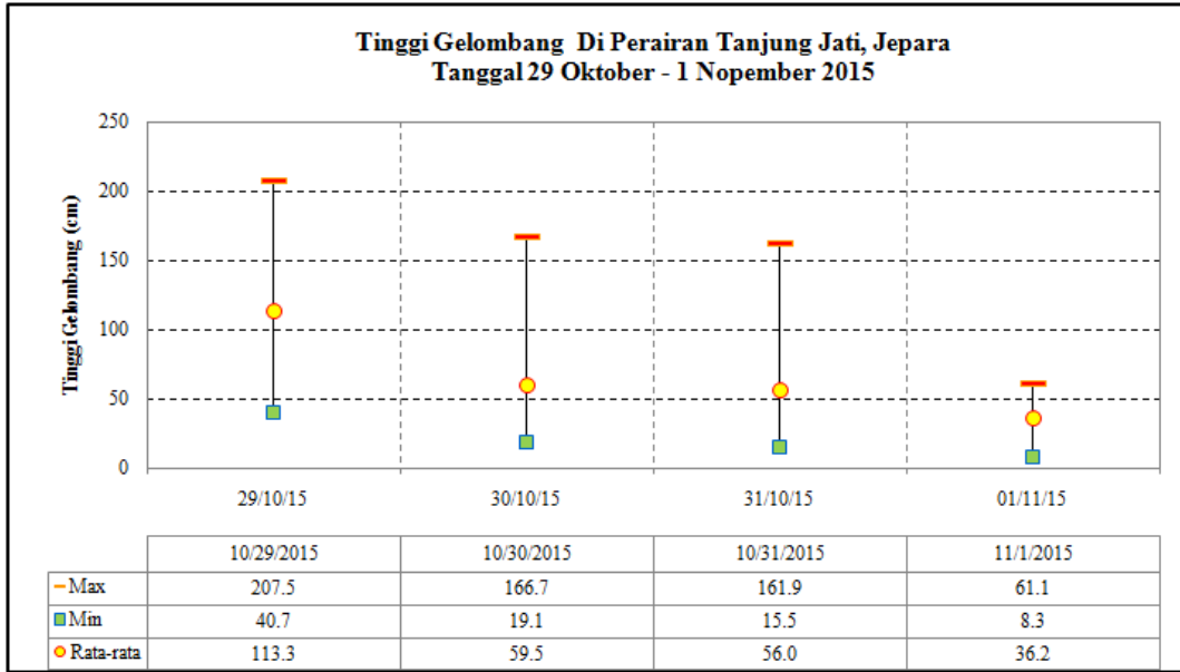
Gambar 2.51. Tinggi Gelombang harian hasil pembacaan ADCP pada permukaan air di Perairan Tanjung Jati, Jepara Tanggal 29 Oktober - 1 November 2015 (Sumber: Analisis Data, November 2015)
