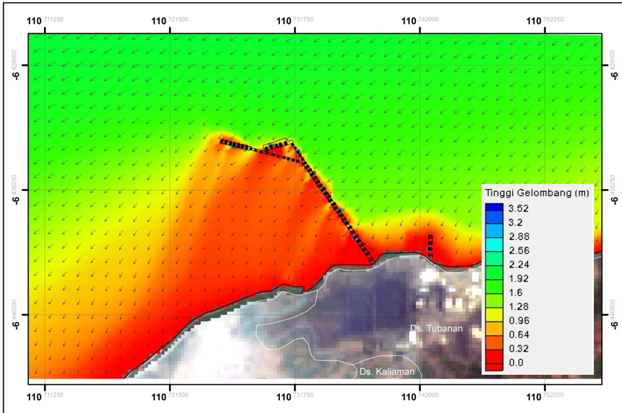
Gambar 2.60. Hasil permodelan gelombang zona 2 pada musim peralihan 1 kondisi eksisting (Sumber : Hasil Pemodelan, September 2015)
