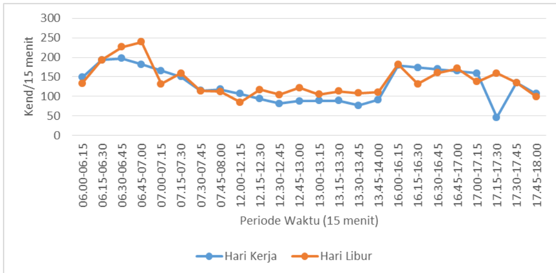
Gambar 2.154. Fluktuasi Arus Lalu lintas di Simpang 3 Tak Bersinyal Wedelan (Sumber: Survei Lapangan, 2015)
