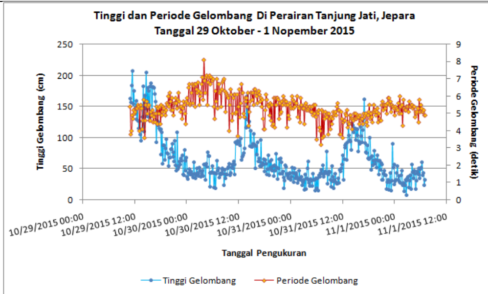
Gambar 2.53. Raw Data Tinggi dan Periode Gelombang hasil pembacaan ADCP pada permukaan air di Perairan Tanjung Jati, Jepara Tanggal 29 Oktober - 1 November 2015 (Sumber: Analisis Data, November 2015)
