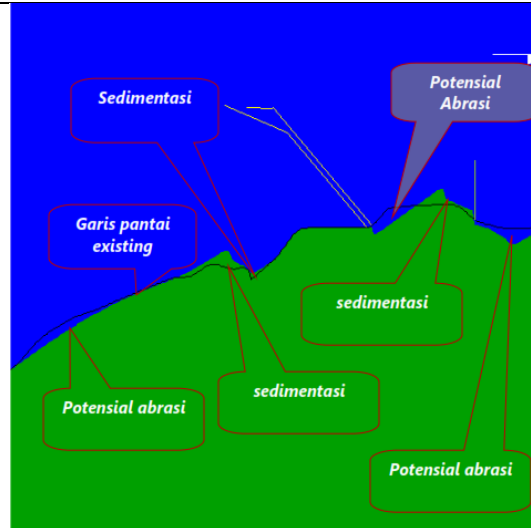
Gambar 2.124. Hasil Model Musim Barat Perubahan Garis Pantai di Perairan Tanjung Jati, Jepara, Kondisi Eksisting Tahun Kelima
