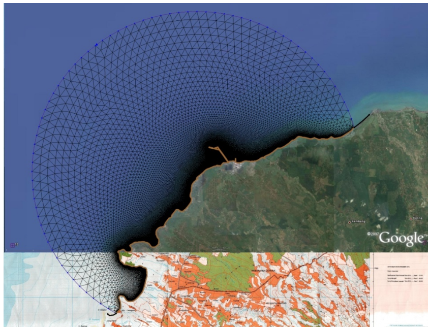
Gambar 2.95. Grid Fleksibel Pemodelan Pada Kondisi Eksisting (Sumber: Hasil Pemodelan, September 2015)
