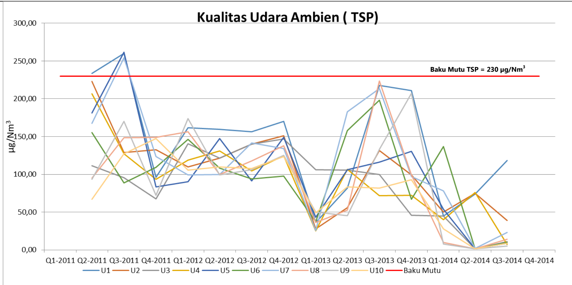
Gambar 2.9. Profil kualitas udara(TSP) Pemantauan PLTU Tanjung Jati B Unit 3&4 Sumber: Hasil Pemantauan PLTU Tanjung Jati B Unit 3&4, 2011-2014 yang dimodifikasi
