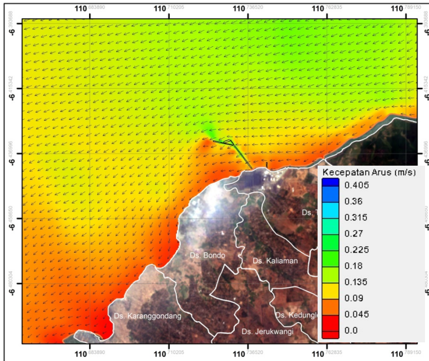
Gambar 2.110. Hasil permodelan arus musim peralihan 2 zona 1 kondisi eksisting (surut menuju pasang) (Sumber : Hasil Pemodelan, September 2015)
