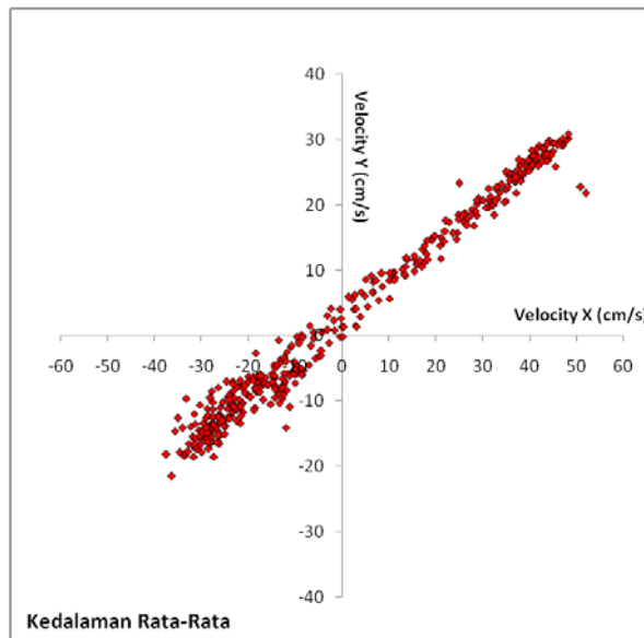
Gambar 2.88. Scatter plot kecepatan arus kedalaman Rata-rata di Perairan Tanjung Jati, Jepara Tanggal 29 Oktober - 1 November 2015 (Sumber: Analisis Data, November 2015)
