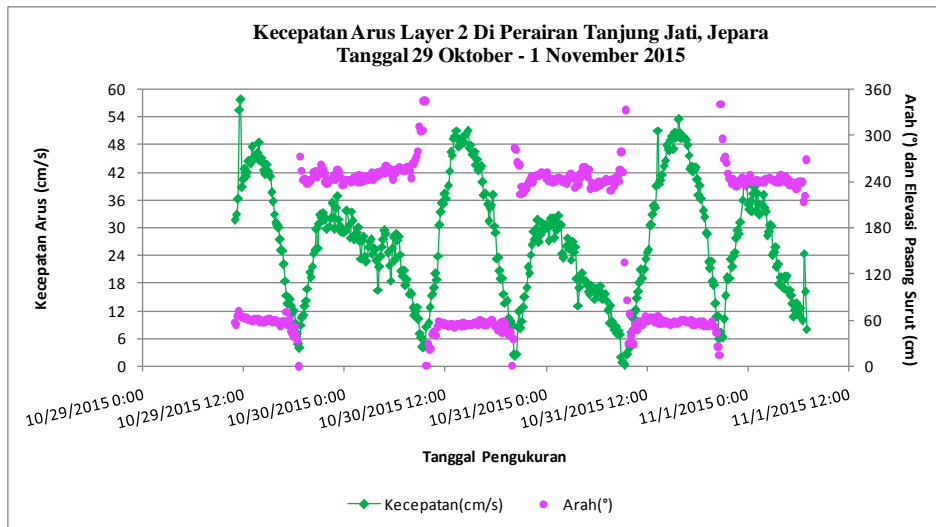
Gambar 2.76. Kecepatan arus kedalaman 7,2 - 9 meter ( layer 2 ) di Perairan Tanjung Jati, Jepara Tanggal 29 Oktober - 1 November 2015 (Sumber: Analisis Data, November 2015)
