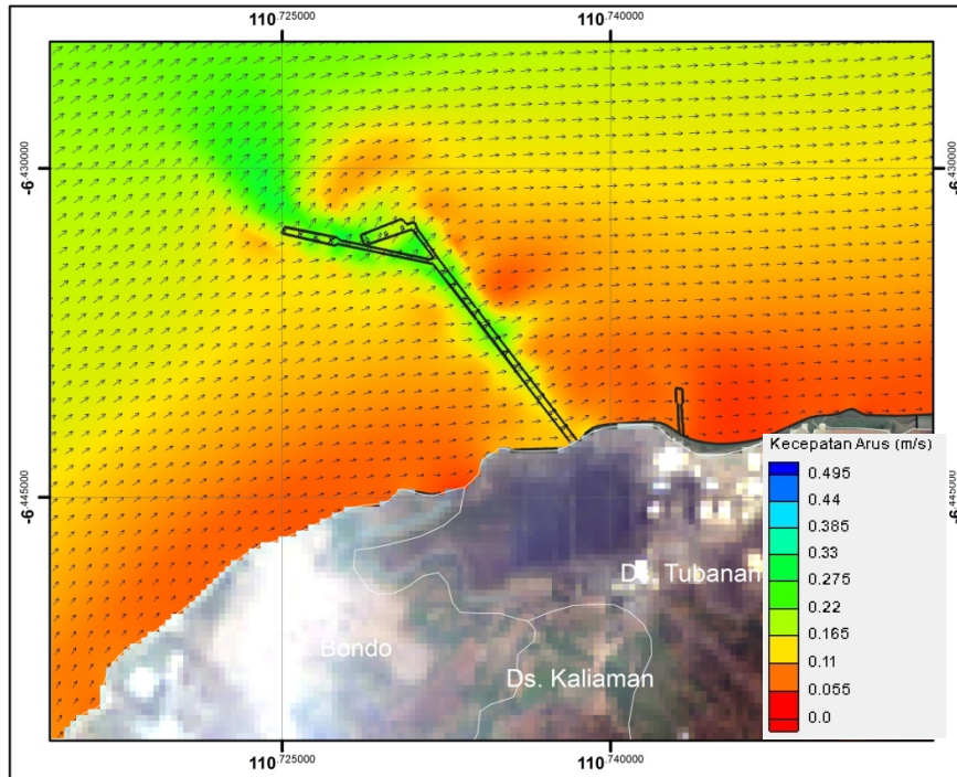
Gambar 2.99. Hasil permodelan arus musim barat zona 2 kondisi eksisting (pasang menuju surut) (Sumber: Hasil Pemodelan, September 2015)
