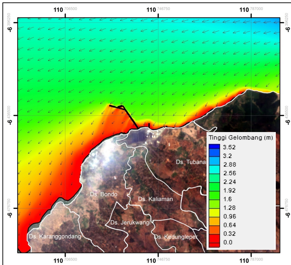
Gambar 2.59. Hasil permodelan gelombang zona 1 pada musim peralihan 1 kondisi eksisting (Sumber : Hasil Pemodelan, September 2015)
