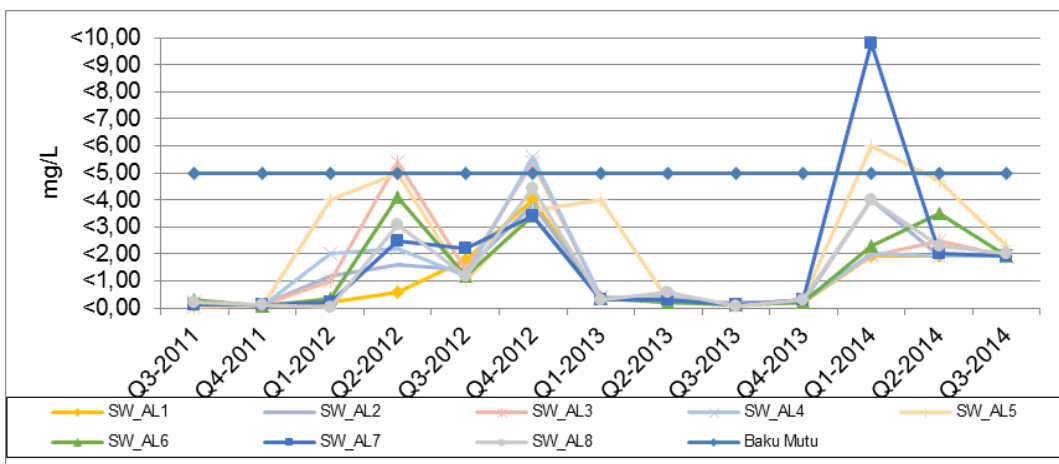
Gambar 2.32. Kualitas Air Laut ( Oils and Fats ) pemantauan PLTU Tanjung Jati B Unit 3 & 4 pada tahun 2011-2014 (sumber: Hasil pemantauan PLTU Tanjung Jati B Unit 1-4, 2010-2014)
