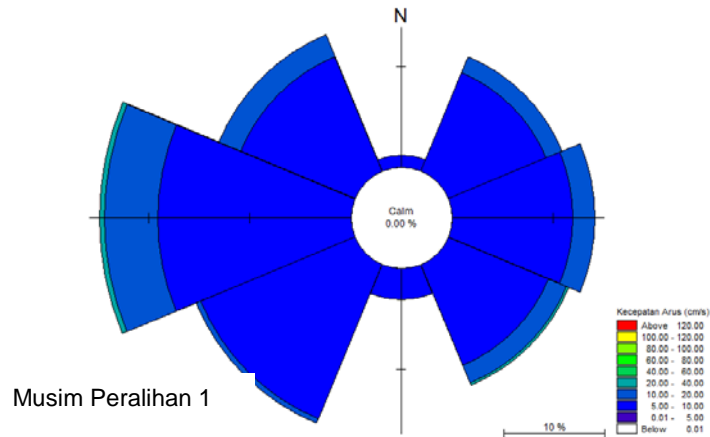
Gambar 2.69. Kondisi arus ( currentrose ) musim peralihan 1 tahun 2007-2014 (Sumber data: BMKG-SMM Semarang, 2007-2014)
