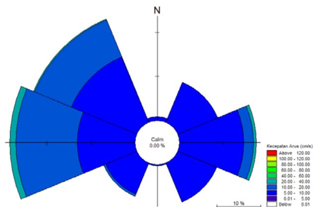
Gambar 2.70. Kondisi arus ( currentrose ) musim peralihan 2 tahun 2007-2014 (Sumber data: BMKG-SMM Semarang, 2007-2014)
