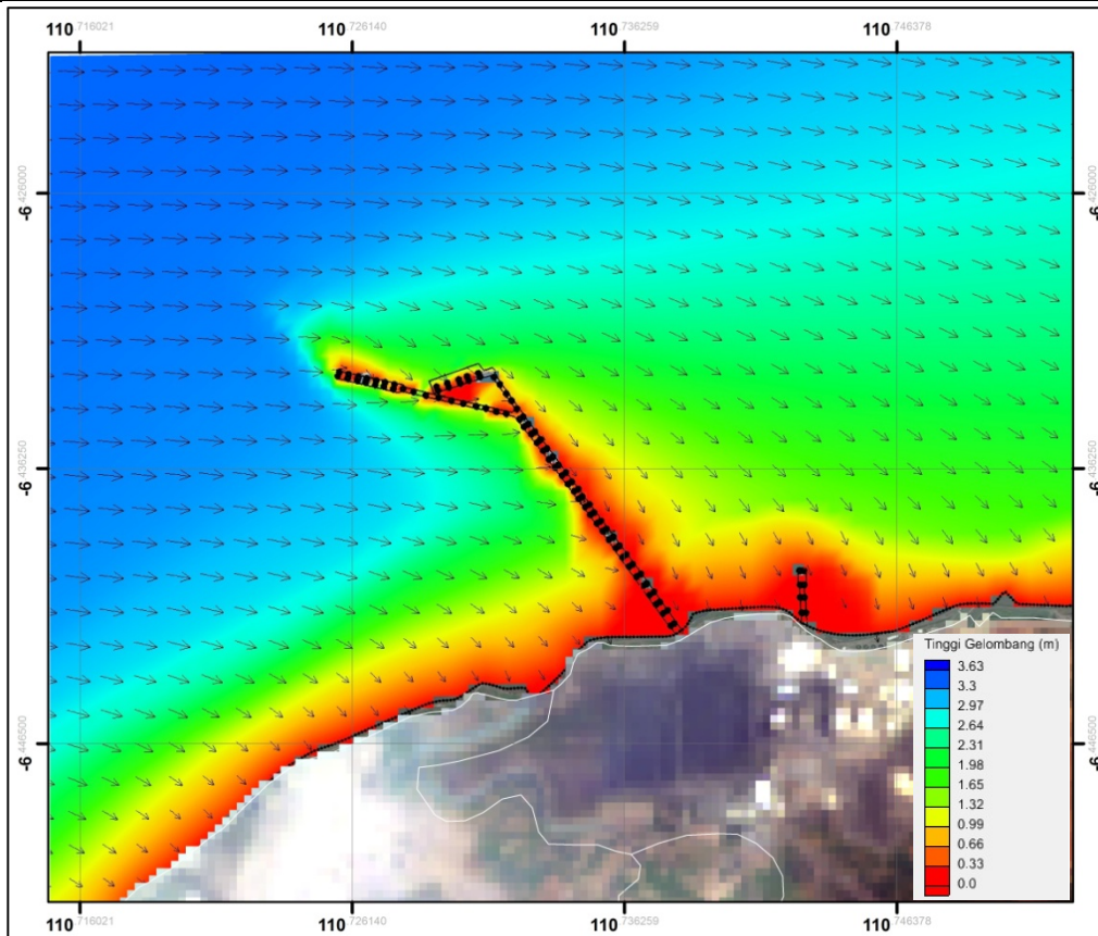
Gambar 2.58. Hasil permodelan gelombang zona 2 pada musim barat kondisi eksisting (Sumber : Hasil Pemodelan, September 2015)
