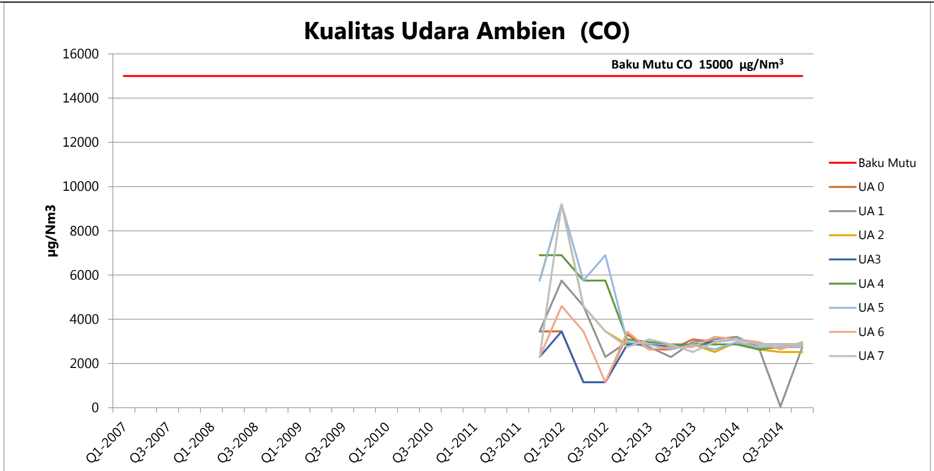
Gambar 2.14. Profil kualitas udara ambien (CO) PLTU Tanjung Jati B Unit 1&2 (sumber: Hasil Pemantauan PLTU Tanjung Jati B Unit 1&2, 2011-2014 Yang dimodifikasi)
