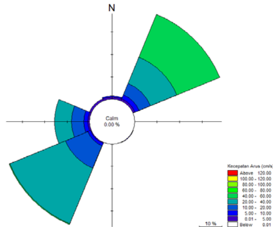
Gambar 2.81. Current rose kedalaman rata-rata di Perairan Tanjung Jati, Jepara Tanggal 29 Oktober - 1 November 2015 (Sumber: Analisis Data, November 2015)
