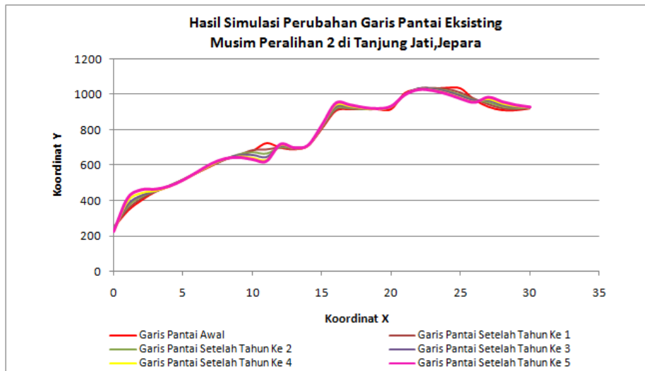
Gambar 2.146. Hasil Simulasi Perubahan Garis Pantai Eksisting Musim Peralihan 2 di Perairan Tanjung Jati, Jepara
