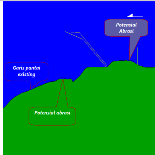
Gambar 2.134. Hasil Model Musim Timur Perubahan Garis Pantai di Perairan Tanjung Jati, Jepara, Kondisi Eksisting Tahun Pertama
