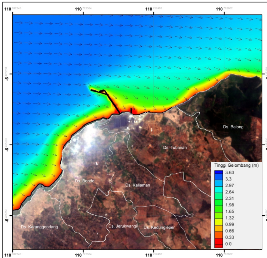
Gambar 2.57. Hasil permodelan gelombang zona 1 pada musim barat kondisi eksisting (Sumber: Hasil Pemodelan, September 2015)
