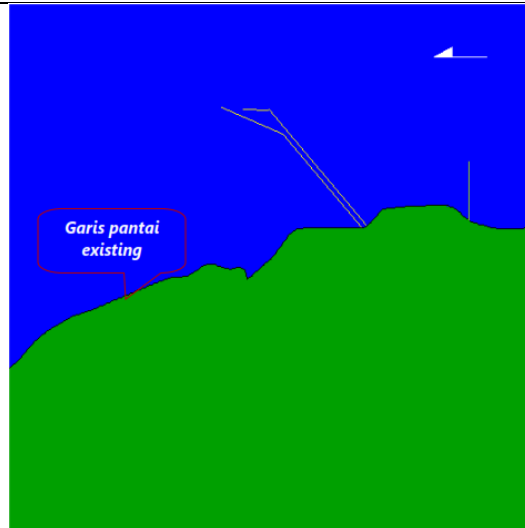
Gambar 2.126. Hasil Model Musim Peralihan 1 Perubahan Garis Pantai di Perairan Tanjung Jati, Jepara, Kondisi Eksisting
