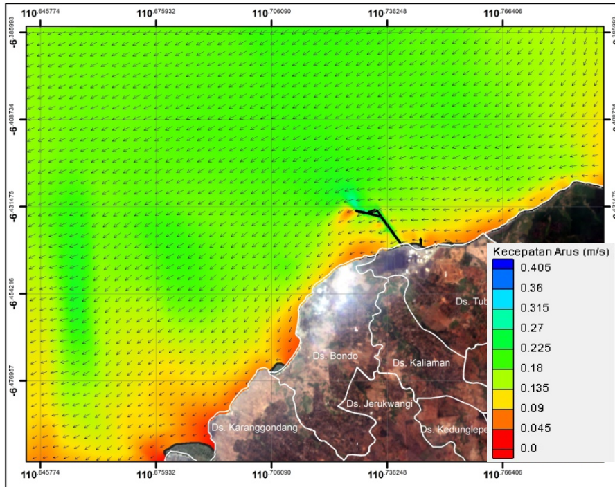
Gambar 2.106. Hasil permodelan arus musim timur zona 1 kondisi eksisting (surut menuju pasang) (Sumber: Hasil Pemodelan, September 2015)
