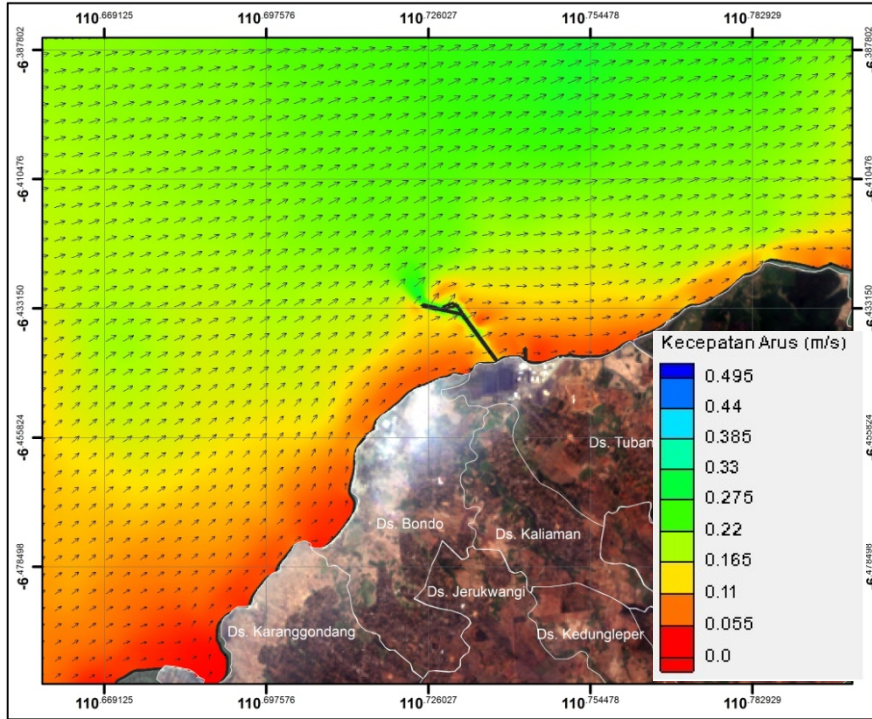
Gambar 2.97. Hasil permodelan arus musim barat zona 1 kondisi eksisting (pasang menuju surut) (Sumber: Hasil Pemodelan, September 2015)
