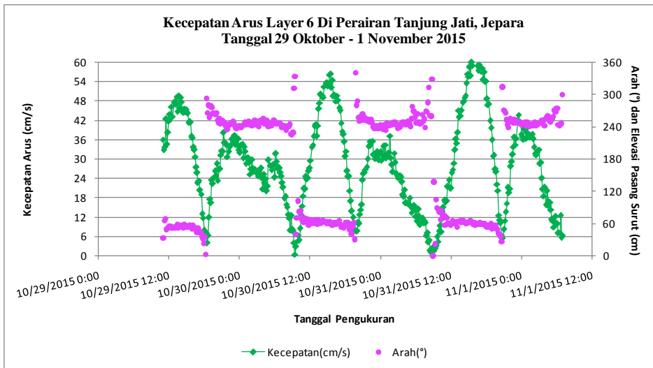
Gambar 2.80. Kecepatan arus kedalaman 0 - 1,8 meter ( layer 6 ) di Perairan Tanjung Jati, Jepara Tanggal 29 Oktober - 1 November 2015 (Sumber: Analisis Data, November 2015)
