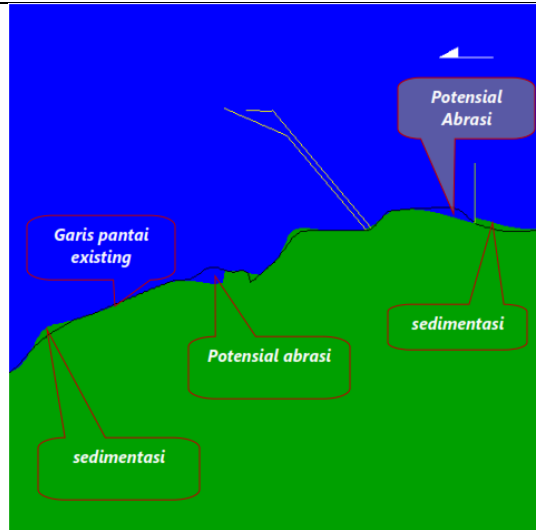
Gambar 2.137. Hasil Model Musim Timur Perubahan Garis Pantai di Perairan Tanjung Jati, Jepara, Kondisi Eksisting Tahun Keempat
