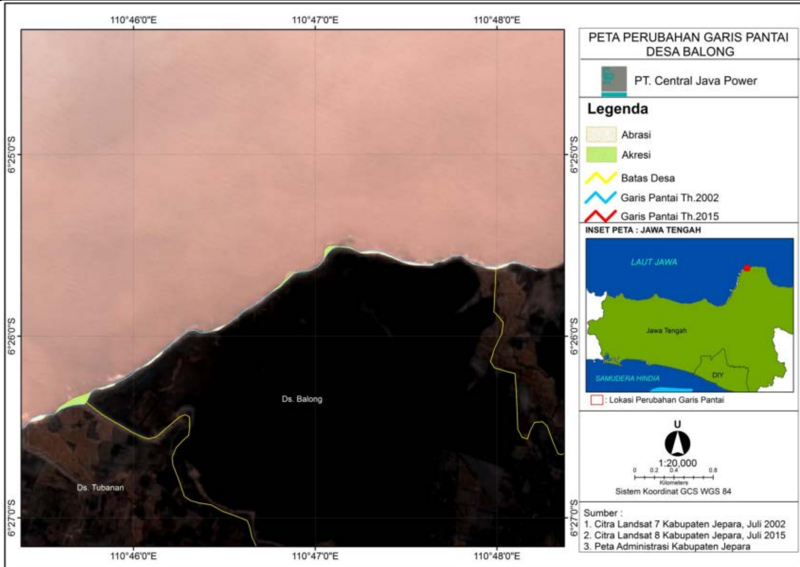
Gambar 2.117. Perubahan Garis Pantai di Desa Balong Jepara pada Perode Tahun 2002-2015
