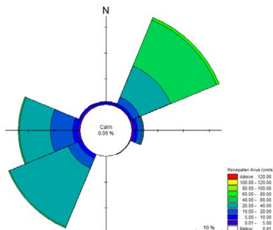
Gambar 2.87. Current rose kedalaman 0 - 1,8 meter ( layer 6 ) di Perairan Tanjung Jati, Jepara Tanggal 29 Oktober - 1 November 2015 (Sumber: Analisis Data, November 2015)
