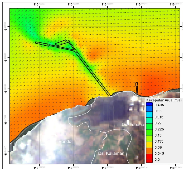
Gambar 2.107. Hasil permodelan arus musim timur zona 2 kondisi eksisting (pasang menuju surut) (Sumber: Hasil Pemodelan, September 2015)
