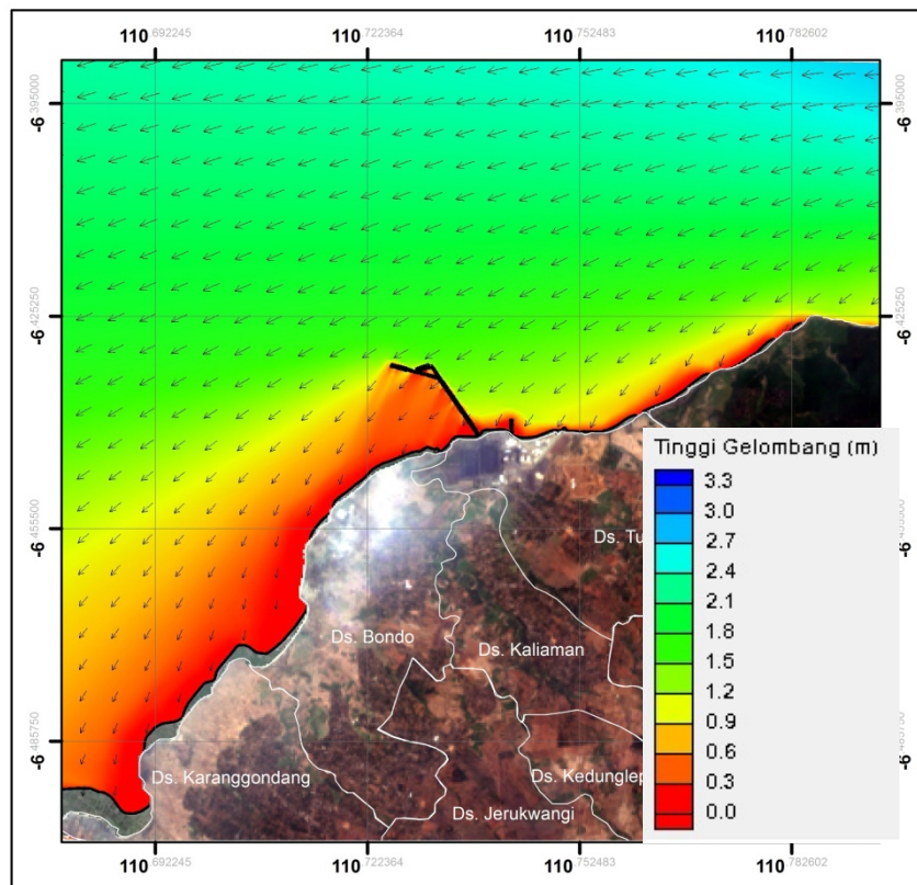
Gambar 2.61. Hasil permodelan gelombang zona 1 pada musim timur kondisi eksisting (Sumber : Hasil Pemodelan, September 2015)
