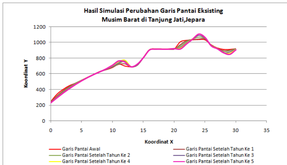
Gambar 2.125. Hasil Simulasi Perubahan Garis Pantai Eksisting Musim Barat di Perairan Tanjung Jati, Jepara
