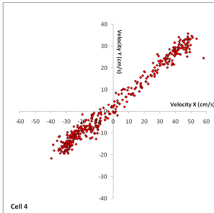
Gambar 2.92. Scatter plot kecepatan arus kedalaman 3,6 – 5,4 meter ( layer 4 ) di Perairan Tanjung Jati, Jepara Tanggal 29 Oktober - 1 November 2015 (Sumber : Analisis Data, November 2015)
