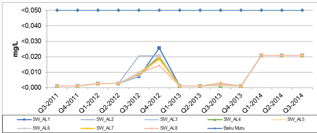
Gambar 2.33. Kualitas Air Laut ( Dissolved Metals - Copper ) pemantauan PLTU Tanjung Jati B Unit 3&4 pada tahun 2011-2014 (sumber: Hasil pemantauan PLTU Tanjung Jati B Unit 1-4, 2010-2014)
