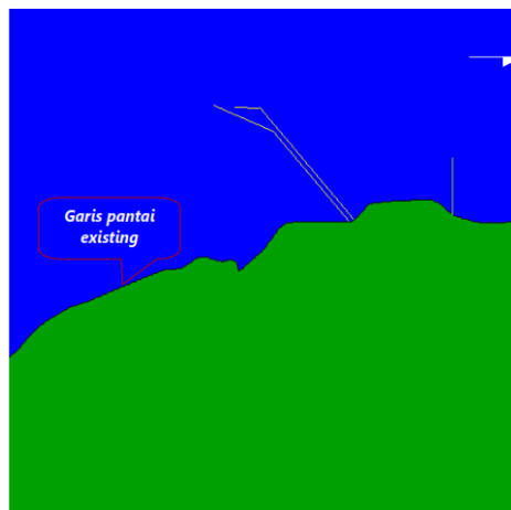
Gambar 2.119. Hasil Model Musim Barat Perubahan Garis Pantai di Perairan Tanjung Jati, Jepara, Kondisi Eksisting
