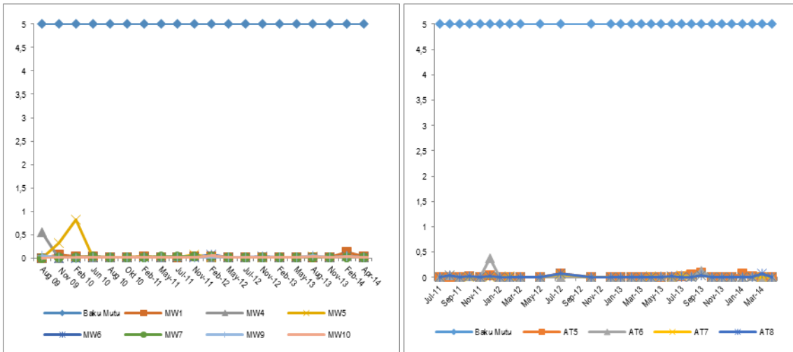
Gambar 2.42. Grafik kualitas air tanah parameter Zn hasil pemantauan Unit 1&2 (kiri) dan Unit 3&4 (kanan) (sumber: Hasil pemantauan Unit 1-4, 2010-2014)
