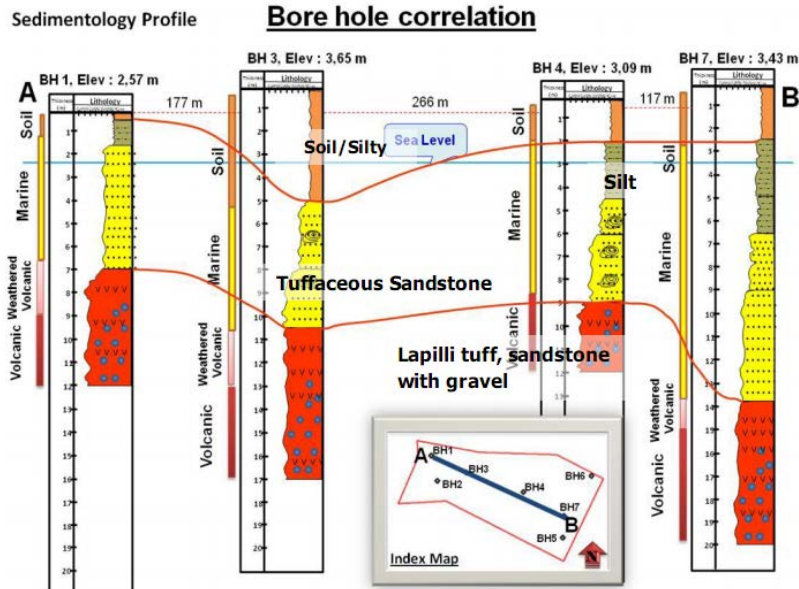
Gambar 2.18. Penampang A-B, menunjukkan korelasi borehole berarah Barat Laut-Tenggara
