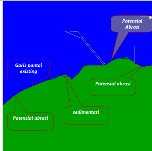
Gambar 2.121. Hasil Model Musim Barat Perubahan Garis Pantai di Perairan Tanjung Jati, Jepara, Kondisi Eksisting Tahun Kedua
