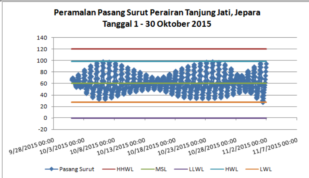
Gambar 2.65. Grafik peramalan pasang surut di Perairan Tanjung Jati, Jepara (Sumber : Analisis Data, November 2015)
