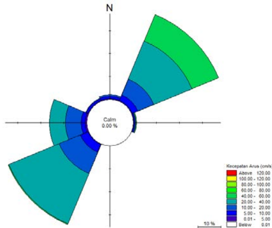
Gambar 2.82. Current rose kedalaman 9 - 10,8 meter ( layer 1 ) di Perairan Tanjung Jati, Jepara Tanggal 29 Oktober - 1 November 2015 (Sumber: Analisis Data, November 2015)
