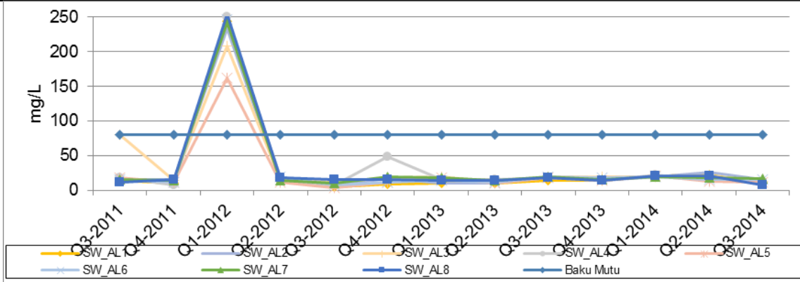
Gambar 2.31. Kualitas Air Laut ( Suspended Solids ) pemantauan PLTU Tanjung Jati B unit 3 & 4 pada tahun 2011-2014 (sumber: Hasil pemantauan PLTU Tanjung Jati B Unit 1-4, 2010-2014)
