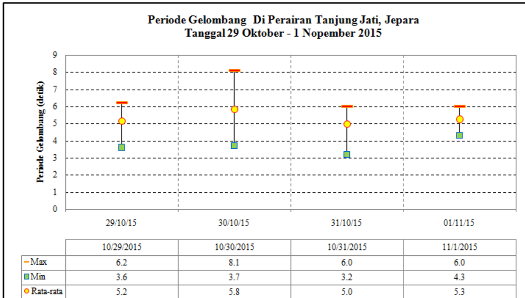
Gambar 2.52. Periode Gelombang harian hasil pembacaan ADCP pada permukaan air di Perairan Tanjung Jati, Jepara Tanggal 29 Oktober - 1 November 2015 (Sumber: Analisis Data, November 2015)
