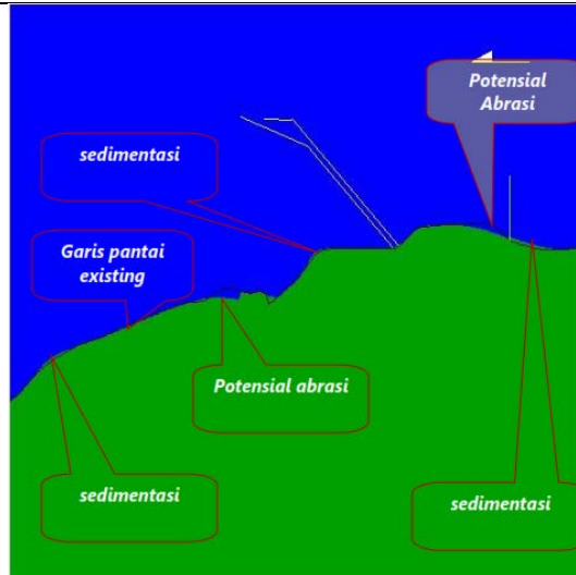
Gambar 2.142. Hasil Model Musim Peralihan 2 Perubahan Garis Pantai di Perairan Tanjung Jati, Jepara, Kondisi Eksisting Tahun Kedua
