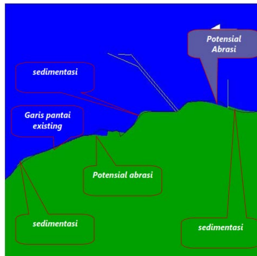
Gambar 2.143. Hasil Model Musim Peralihan 2 Perubahan Garis Pantai di Perairan Tanjung Jati, Jepara, Kondisi Eksisting Tahun Ketiga
