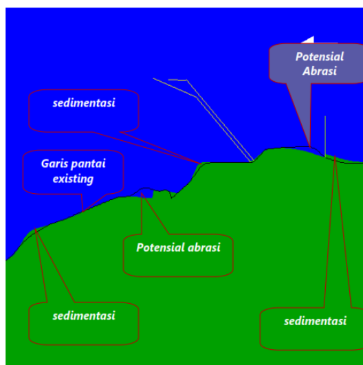
Gambar 2.128. Hasil Model Musim Peralihan 1 Perubahan Garis Pantai di Perairan Tanjung Jati, Jepara, Kondisi Eksisting Tahun Kedua
