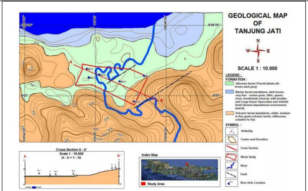
Gambar 2.16. Peta Geologi Tanjung Jati (Tapak Proyek) dan sekitarnya (Geoscience Exploration Consultant, 2011)
