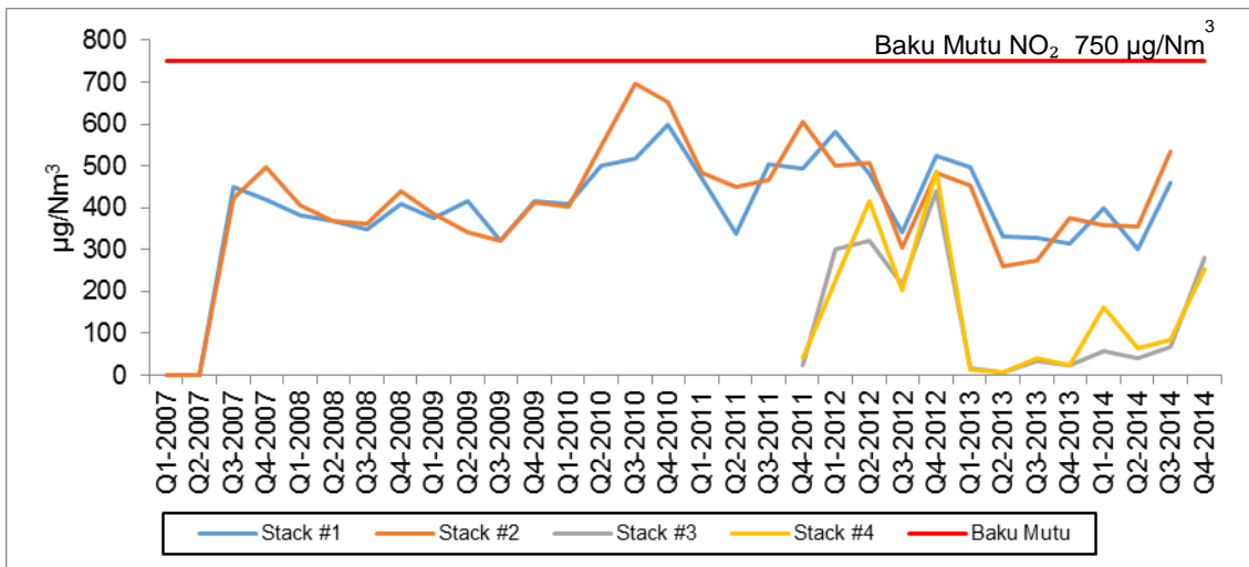
Gambar 2.6. Emisi NO 2 di Cerobong PLTU Tanjung Jati B Unit 1-4 Tahun 2007-2014 (Sumber: hasil pemantauan PLTU Tanjung Jati B Unit 1-4, 2007-2014)
