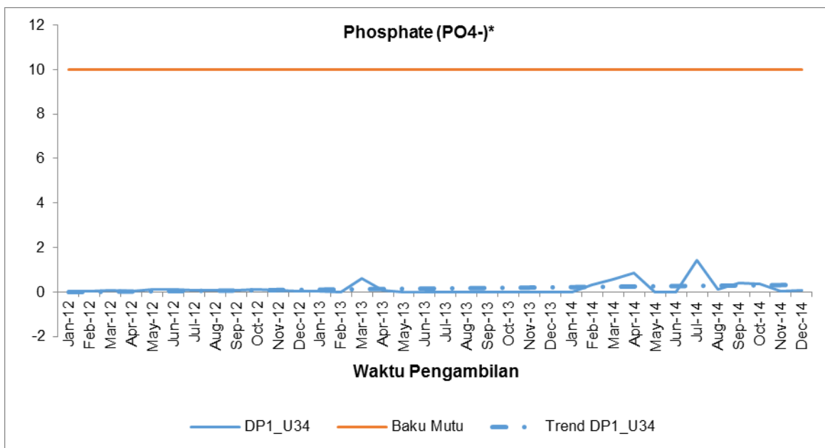
Gambar 2.28. Profil fosfat pada PLTU Tanjung Jati B Unit 3&4 (sumber: hasil pemantauan PLTU Tanjung Jati B Unit 3&4, 2010 – 2014)
