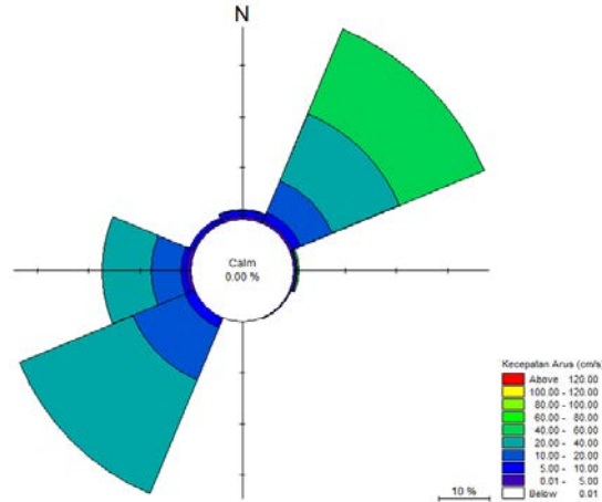
Gambar 2.83. Current rose kedalaman 7,2 - 9 meter ( layer 2 ) di Perairan Tanjung Jati, Jepara Tanggal 29 Oktober - 1 November 2015 (Sumber: Analisis Data, November 2015)
