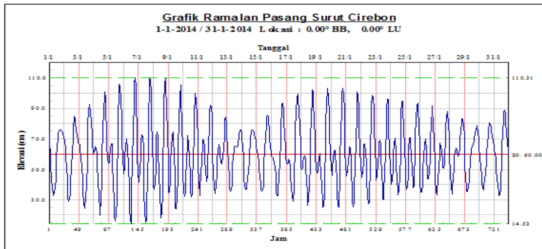
Gambar 2-16 Grafik fluktuasi pasang surut perairan Cirebon Januari 2014.
