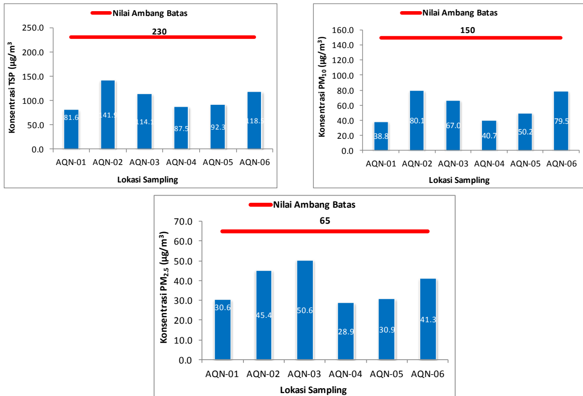
Gambar 2-7 Konsentrasi partikulat (TSP, PM 10 dan PM 2,5 ) di wilayah studi.
