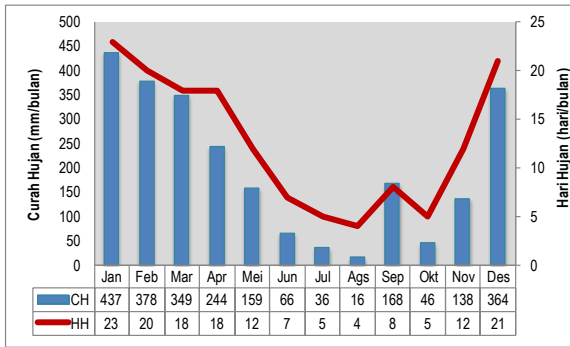
(a) Rata-rata bulanan curah dan hari hujan 2006-2015
