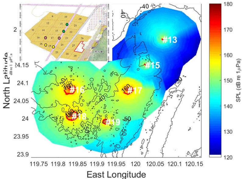
圖 1.2.2-2 環說階段與鄰近風場，假設 6 座風場各 1 部風機同時施工水下噪音模擬圖
