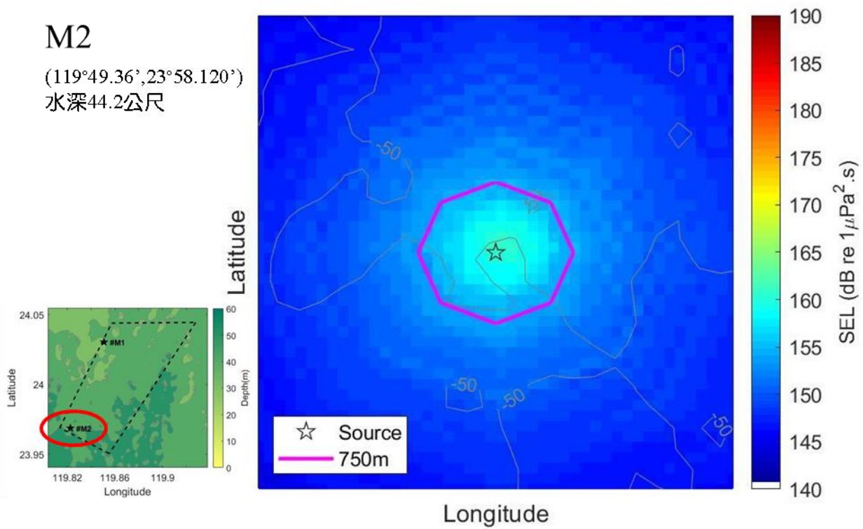
圖 1.4.7-2 M1~M2 點位打樁施工，距離 750 公尺之聲壓分布(減噪後)
