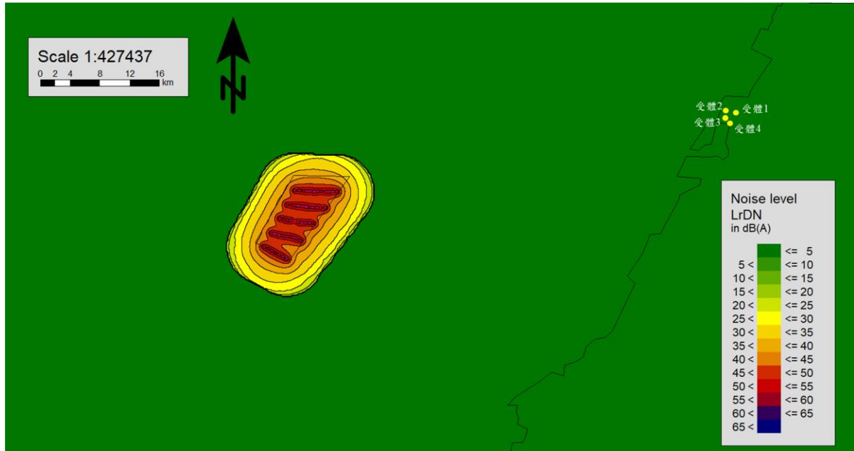
圖 1.9.2-3 變更後營運期間風力機組全頻噪音影響模擬圖
