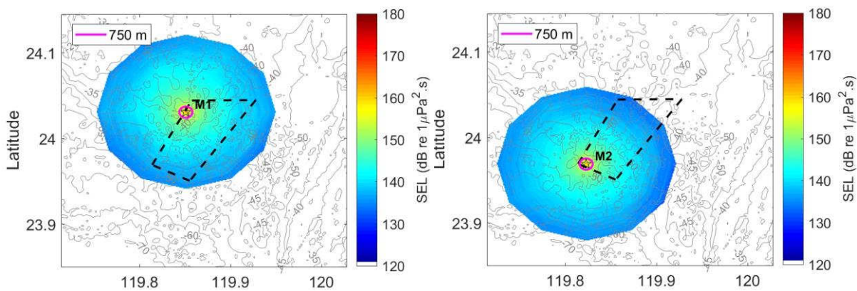
圖 1.9.1-6 原環說 M1~M2 點位打樁施工，經減噪措施後距離 750 公尺之聲壓分布
