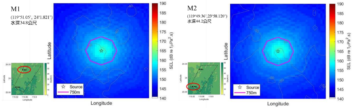
圖 1.8.1-2 M1~M2 點位打樁施工，距離 750 公尺之聲壓分布(減噪後)
