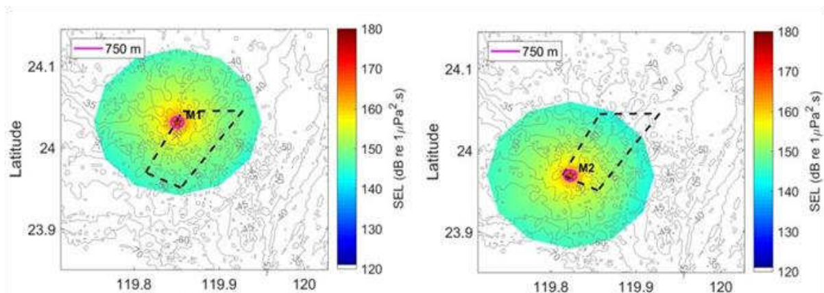
圖 1.9.2-5 原環說 M1~M2 點位打樁施工，距離 750 公尺之聲壓分布
