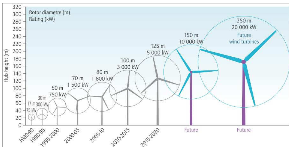
圖 1.2.1-1 國際間風機大型化趨勢
