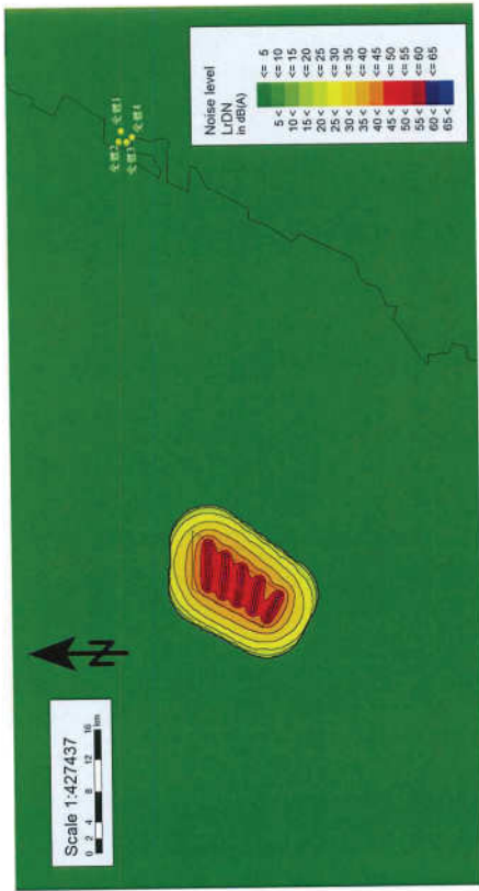
圖 1.1.5-1 營運期間風力機組全頻噪音影響模擬圖
