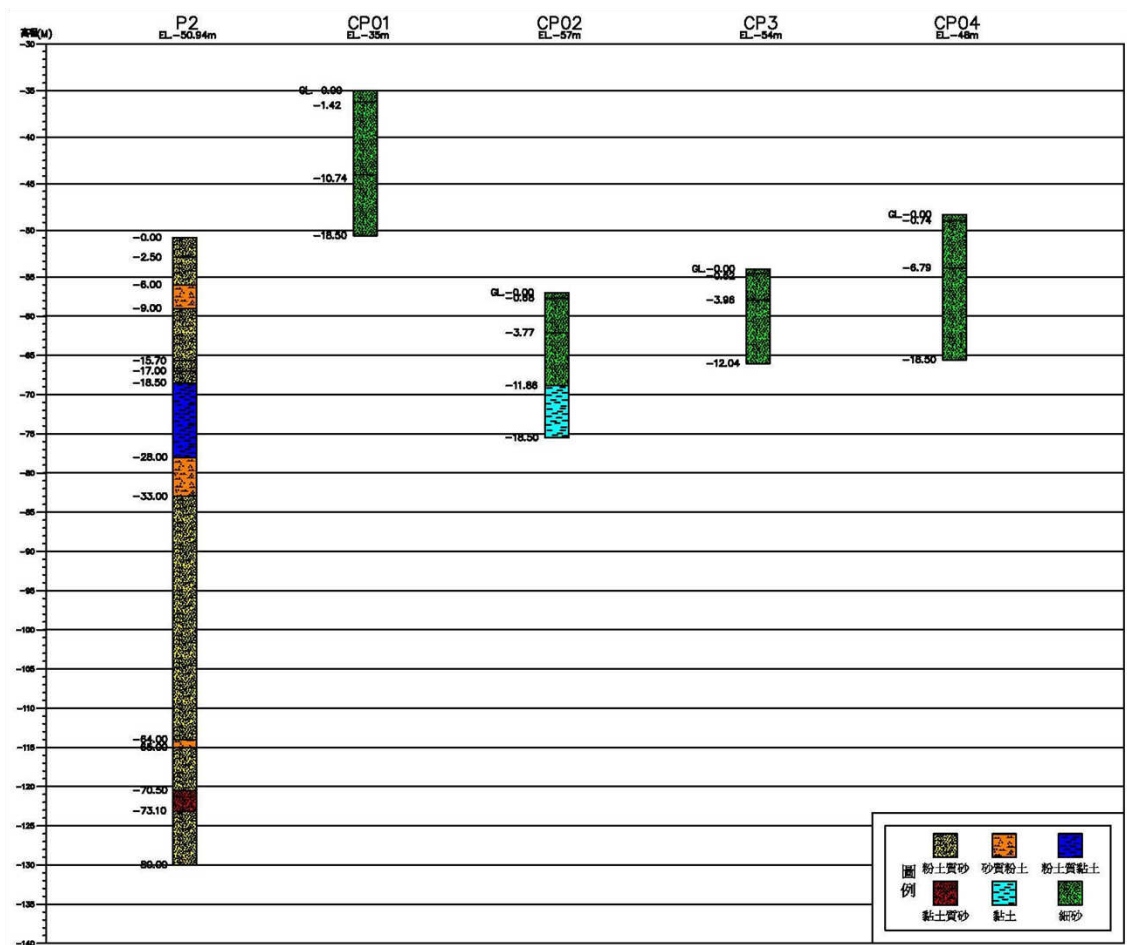
圖 1.6.2-3 地層地質柱狀圖
