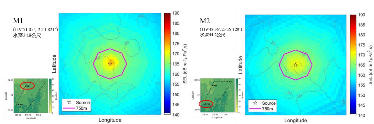
圖 1.8.1-1 M1~M2 點位打樁施工，距離 750 公尺之聲壓分布(減噪前)
