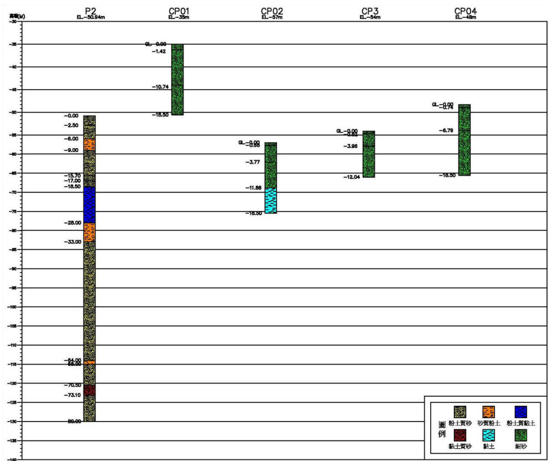
圖 1.8.1-5 地層地質柱狀圖
