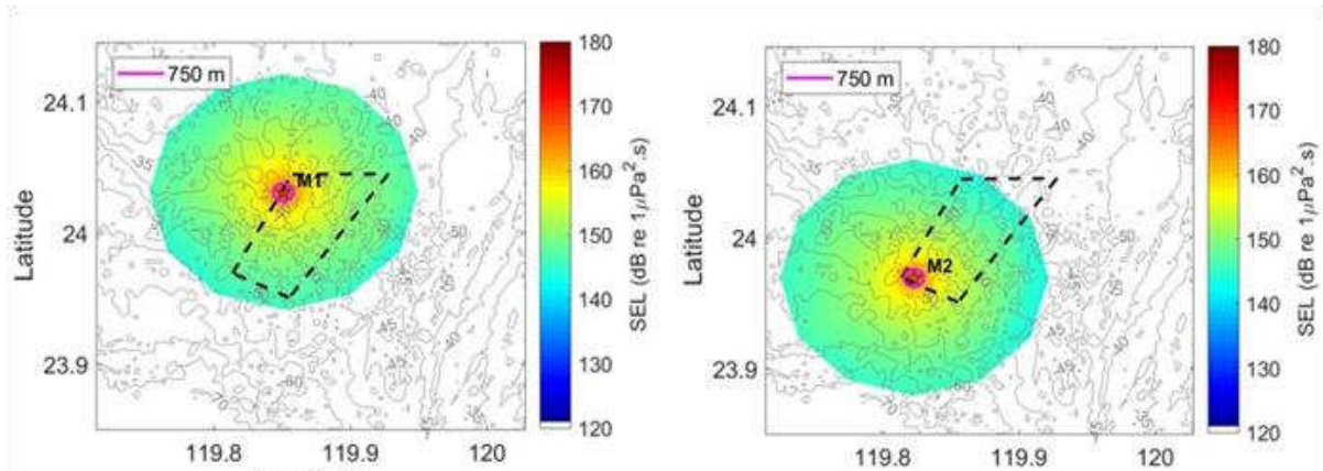
圖 1.7.3-1 原環說 M1~M2 點位打樁施工，距離 750 公尺之聲壓分布
