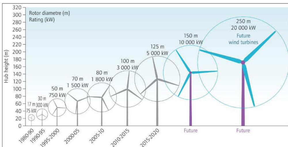
圖 1.5.4-1 國際間風機大型化趨勢
