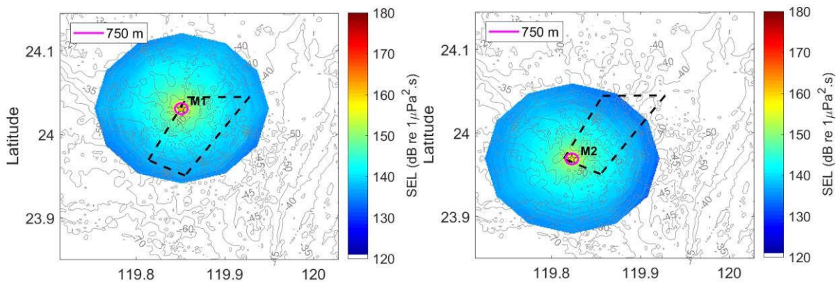
圖 1.7.3-2 原環說 M1~M2 點位打樁施工，經減噪措施後距離 750 公尺之聲壓分布
