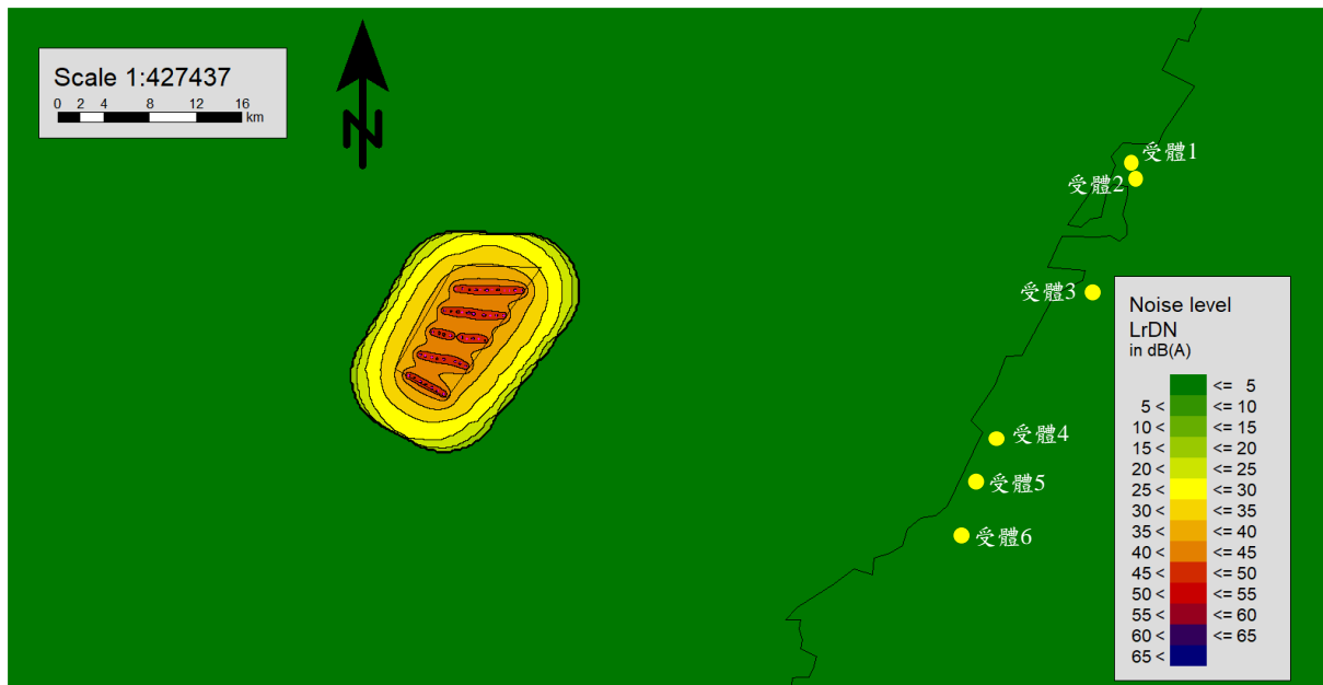
圖 1.1.5-2 變更後營運期間風力機組低頻噪音影響模擬圖
