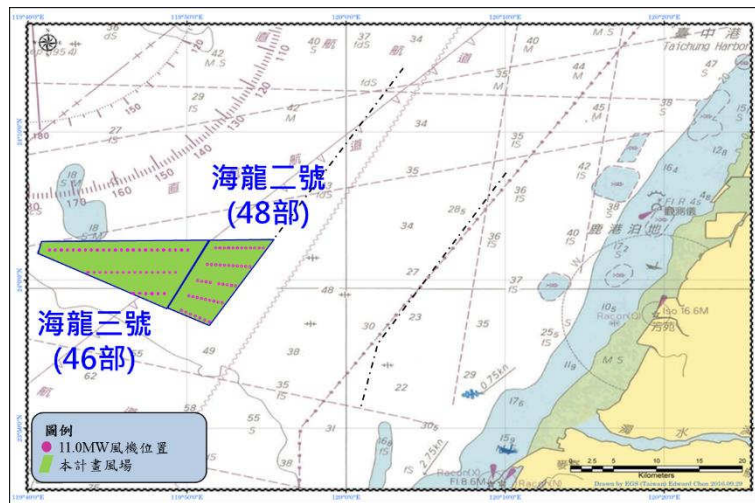
圖 1.9.1-1 原環說 6MW 風機配置示意圖(最多風機數量)
