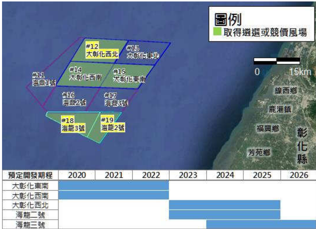
圖 1.2.2-1 彰化地區外海 9 座風場開發場址及預定開發期程示意圖
