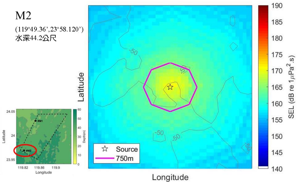
圖 2.2.1-1 M1~M2 點位打樁施工，距離 750 公尺之聲壓分布(減噪前)
