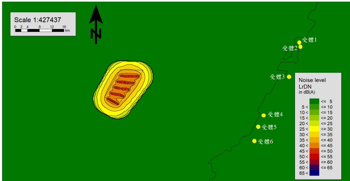
圖 1.9.1-4 變更後營運期間風力機組低頻噪音影響模擬圖
