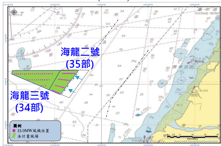
圖 1.9.1-2 本次變更 11MW、15MW 風機配置示意圖
