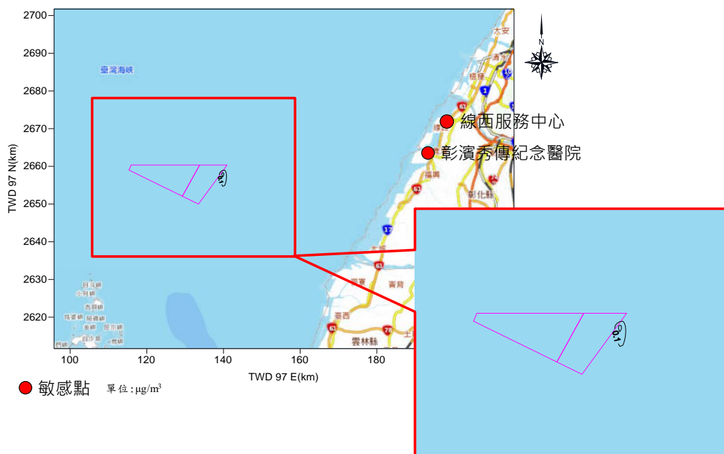
圖 1.9.2-11 原環說船舶海上作業施工期間 TSP 年平均增量模擬圖
