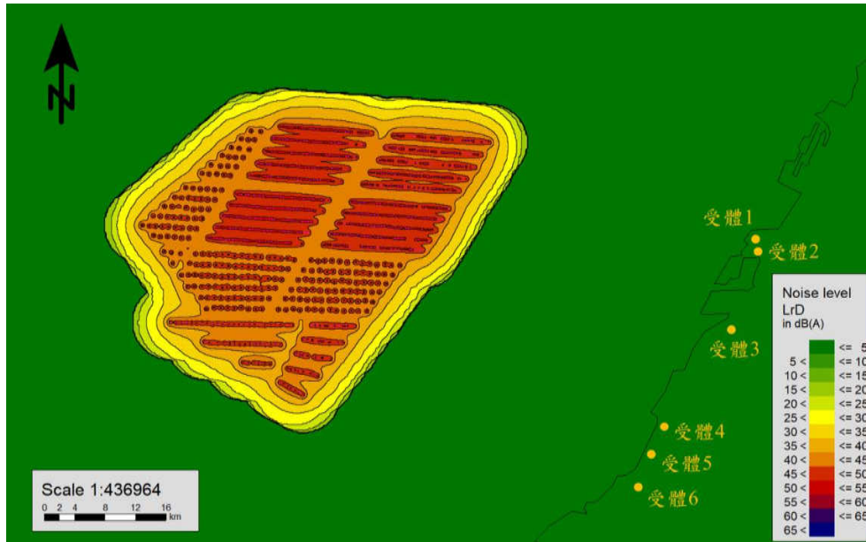
圖 1.2.2-4 彰化地區外海 9 座風場同時運轉之低頻噪音影響模擬圖
