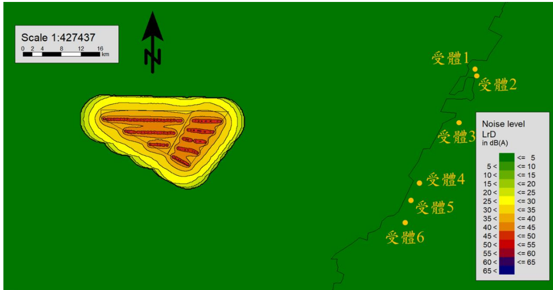
圖 1.1.6-2 變更後海龍二、三號風場-營運期間風力機組低頻噪音影響模擬圖
