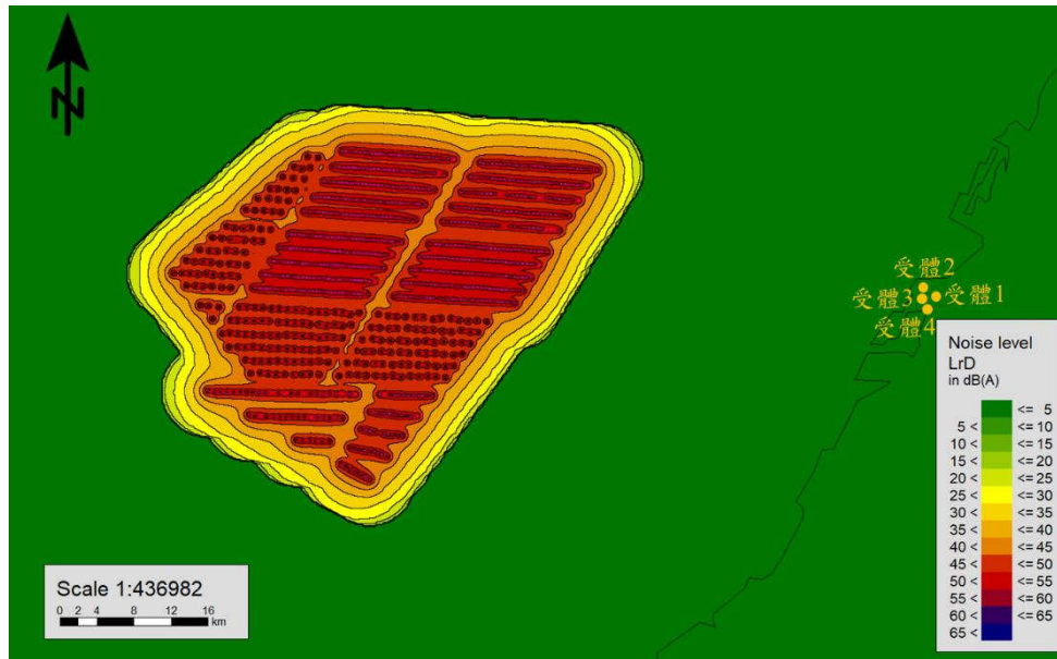
圖 1.2.2-3 彰化地區外海 9 座風場同時運轉之全頻噪音影響模擬圖
