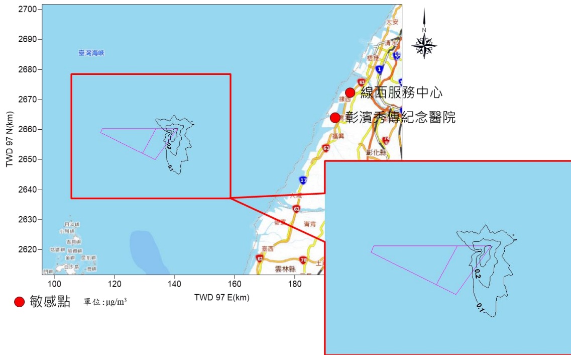
圖 1.4.5-1 船舶海上作業施工期間 TSP 最大日平均值增量模擬圖
