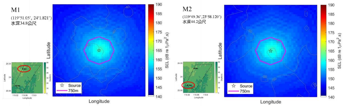
圖 1.7.3-4 M1~M2 點位打樁施工，距離 750 公尺之聲壓分布(減噪後)
