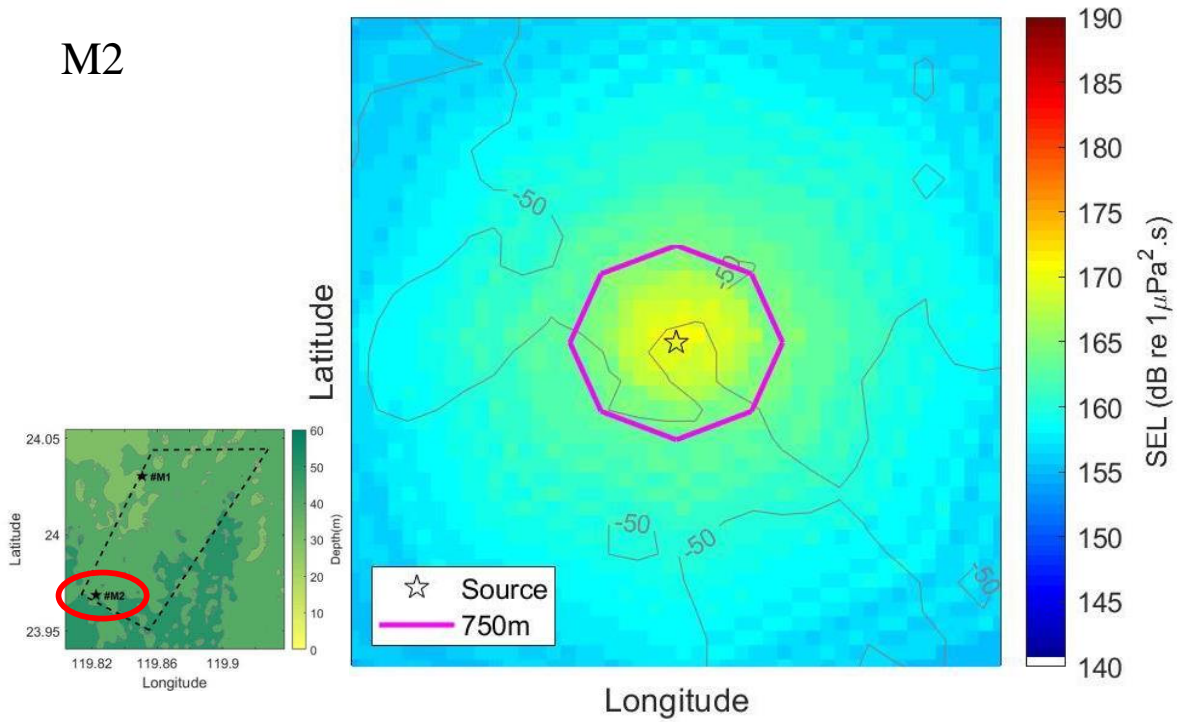
圖 1.1.6-3 M1~M2 點位打樁施工，距離 750 公尺之聲壓分布(減噪前)
