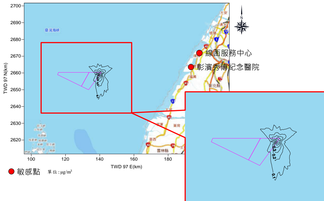
圖 1.9.1-10 原環說船舶海上作業施工期間 TSP 最大日平均值增量模擬圖
