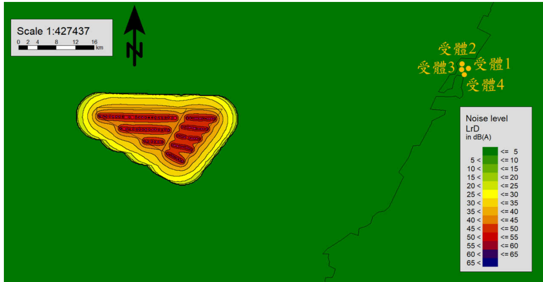
圖 1.1.6-1 變更後海龍二、三號風場-營運期間風力機組全頻噪音影響模擬圖
