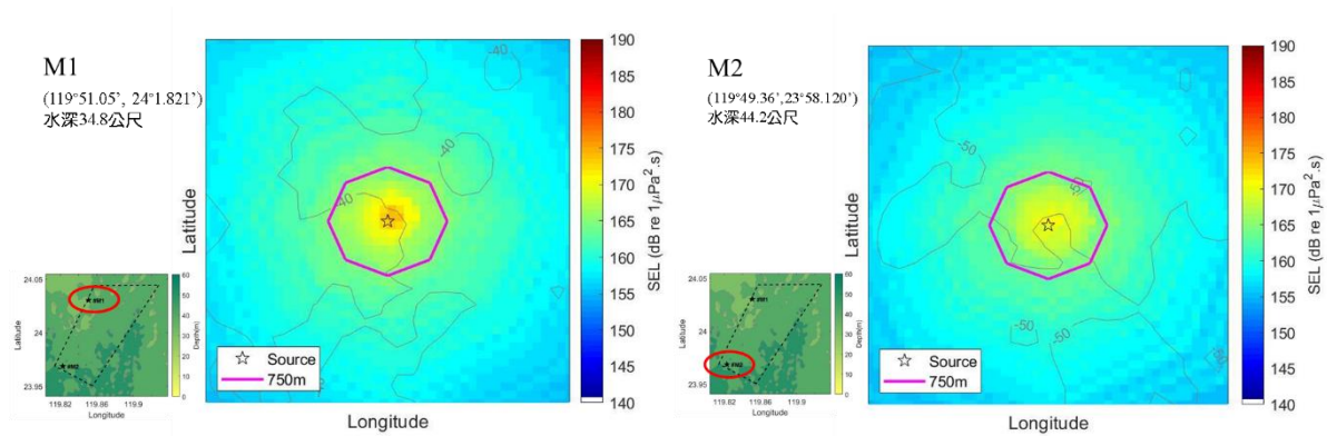
圖 1.9.1-7 M1~M2 點位打樁施工，距離 750 公尺之聲壓分布(減噪前)
