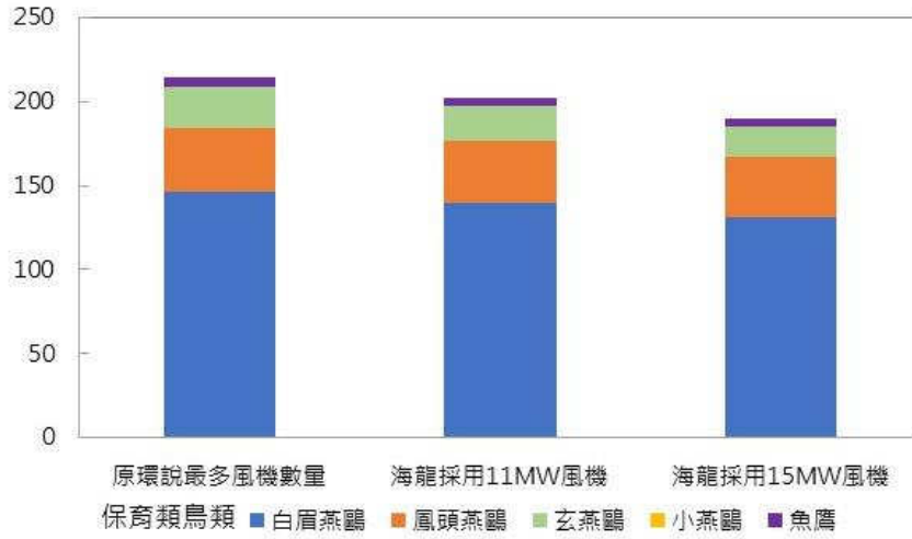
圖 1.2.2-5 彰化地區外海 9 塊風場最多風機數量配置下保育類鳥類之年撞擊隻次
