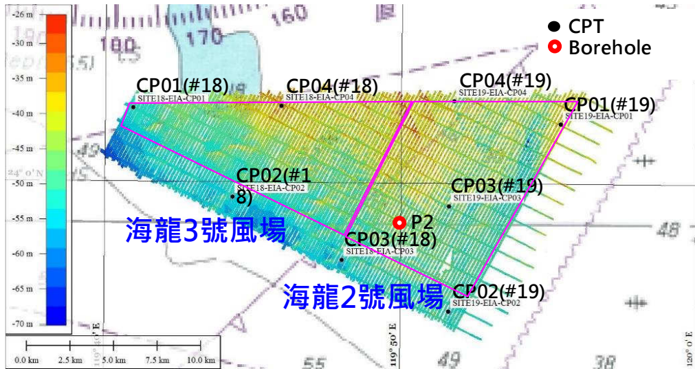
圖 1.3.4-4 地質鑽孔位置圖
