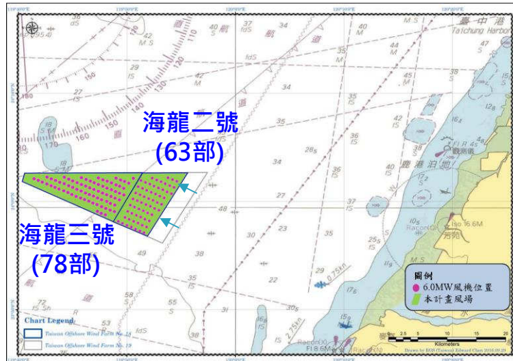
圖 1.9.2-1 原環說 6MW 風機配置示意圖(最多風機數量)
