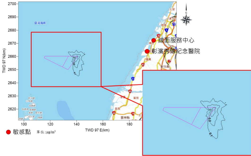
圖 1.9.2-12 本次變更船舶海上作業施工期間 TSP 最大日平均值增量模擬圖
