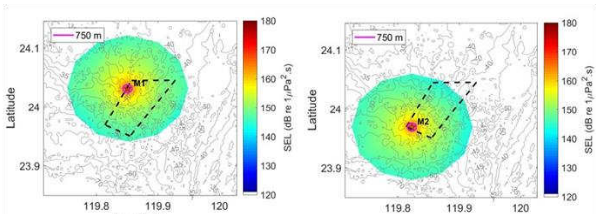
圖 1.9.1-5 原環說 M1~M2 點位打樁施工，距離 750 公尺之聲壓分布
