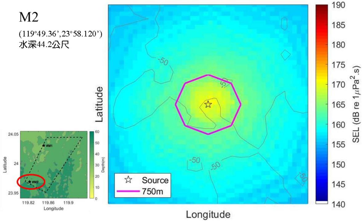
圖 2.8.1-1 M1~M2 點位打樁施工，距離 750 公尺之聲壓分布(減噪前)
