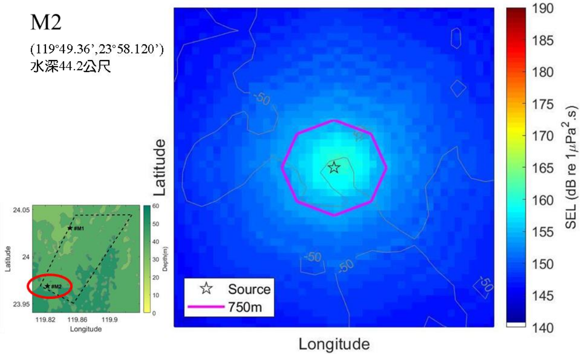
圖 2.8.1-2 M1~M2 點位打樁施工，距離 750 公尺之聲壓分布(減噪後)
