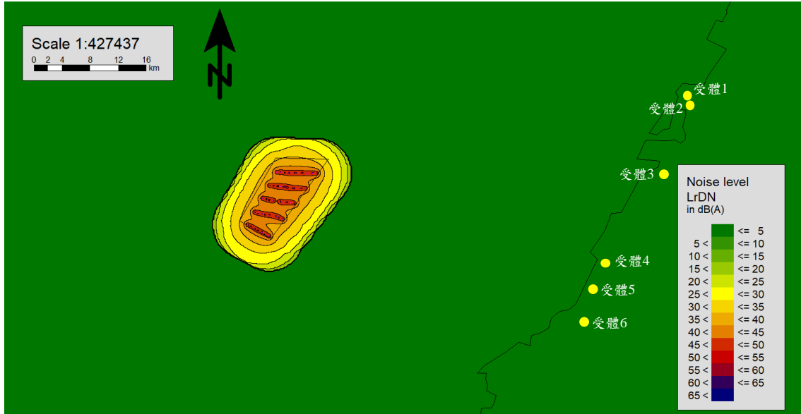
圖 1.4.6-2 變更後營運期間風力機組低頻噪音影響模擬圖
