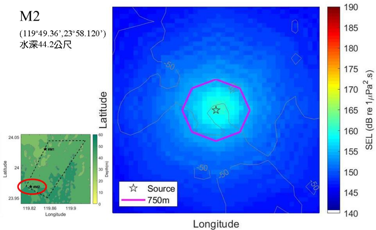
圖 2.2.1-2 M1~M2 點位打樁施工，距離 750 公尺之聲壓分布(減噪後)
