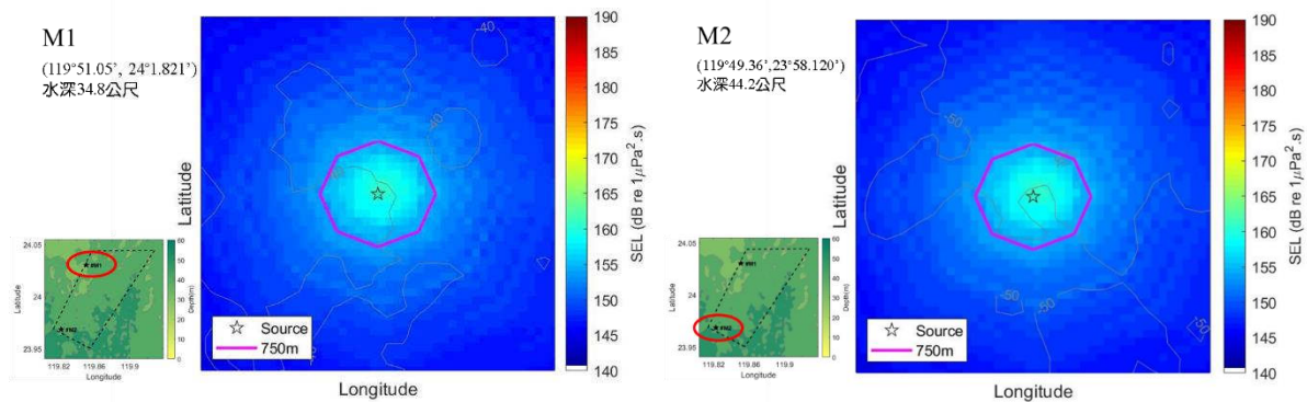
圖 1.9.1-8 M1~M2 點位打樁施工，距離 750 公尺之聲壓分布(減噪後)
