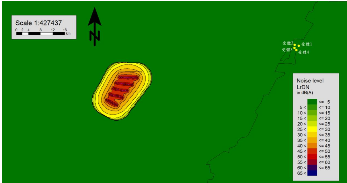
圖 1.1.5-1 變更後營運期間風力機組全頻噪音影響模擬圖
