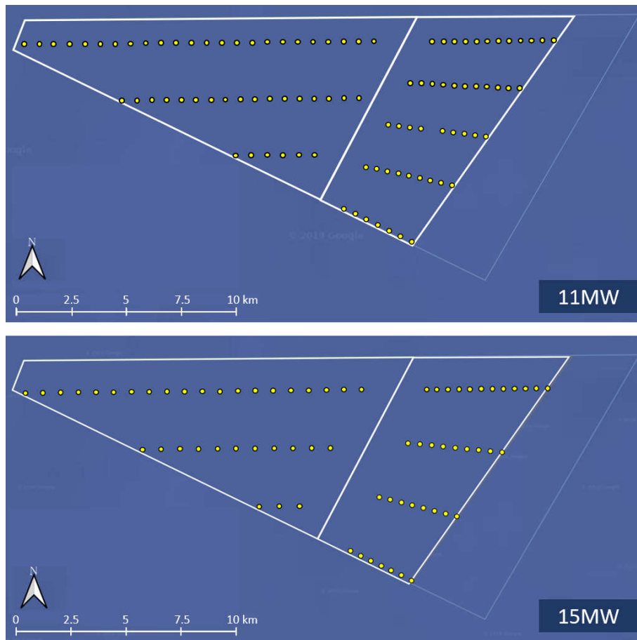
圖 1.2.1-2 本次變更 11MW 及 15MW 風機佈設示意圖
