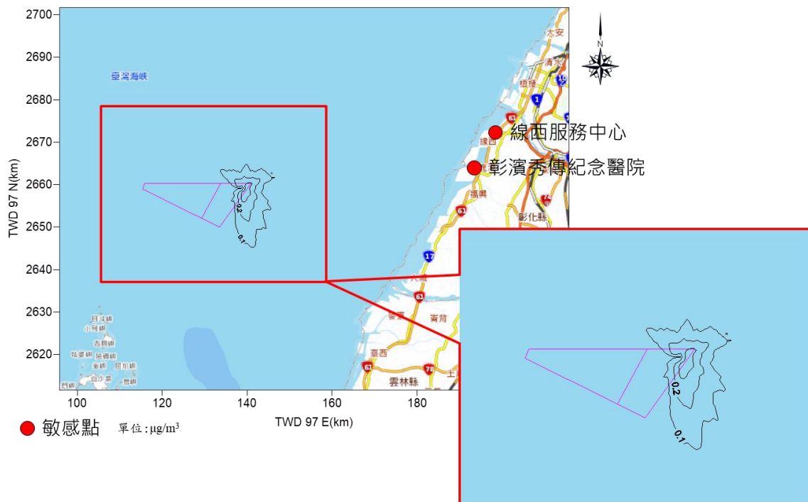
圖 1.1.3-1 船舶海上作業施工期間 TSP 最大日平均值增量模擬圖
