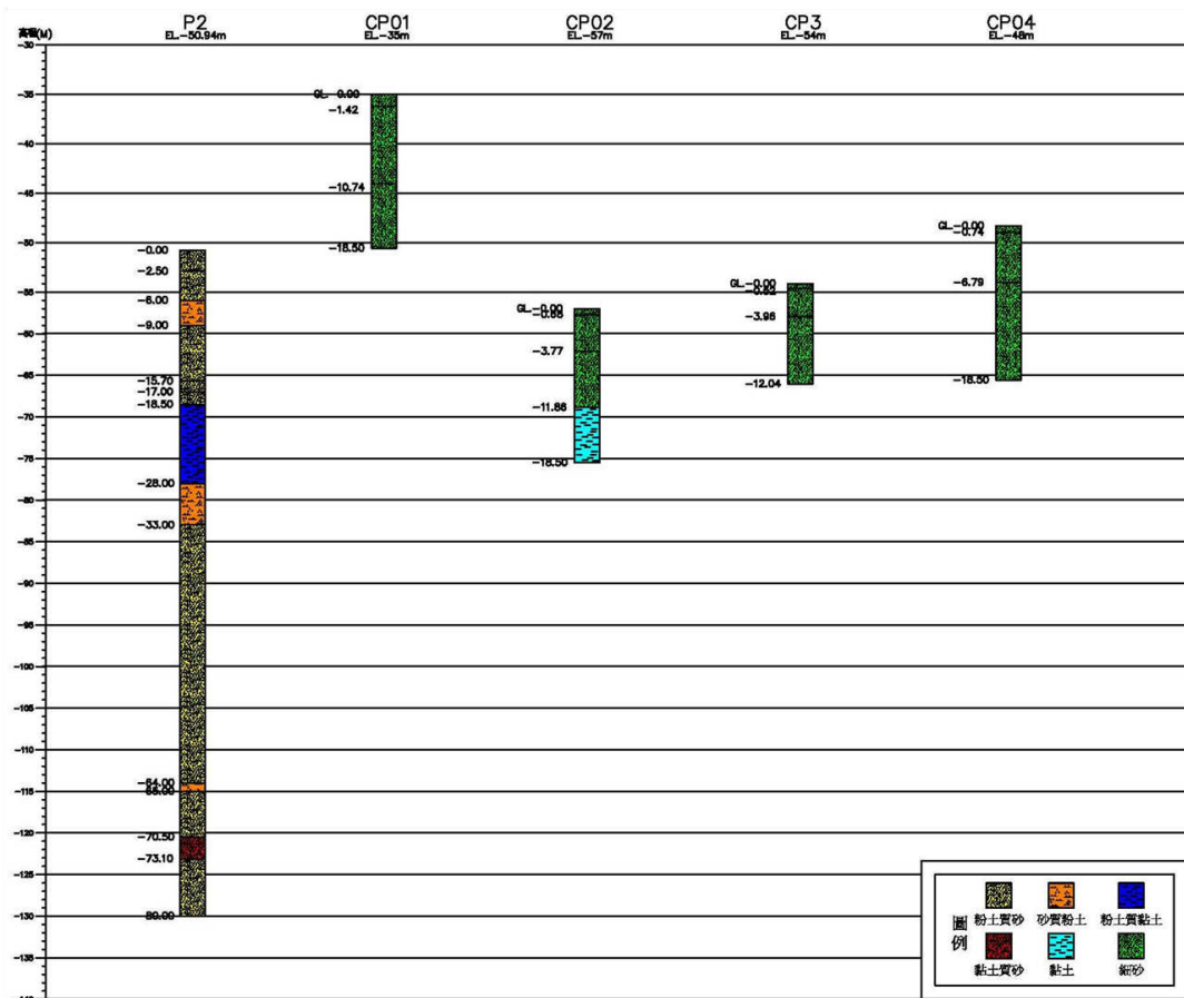
圖 1.3.4-5 地層地質柱狀圖
