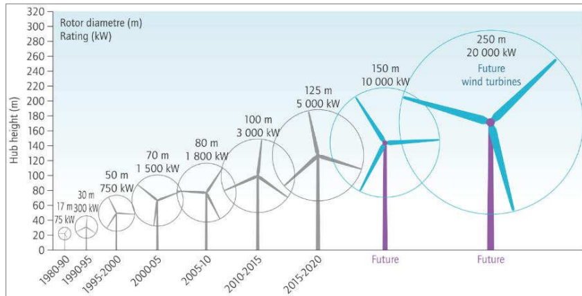
圖 2.5.3-1 國際間風機大型化趨勢
