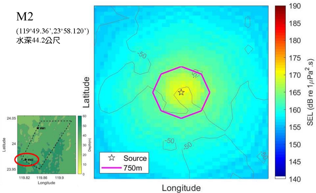
圖 1.4.7-1 M1~M2 點位打樁施工，距離 750 公尺之聲壓分布(減噪前)
