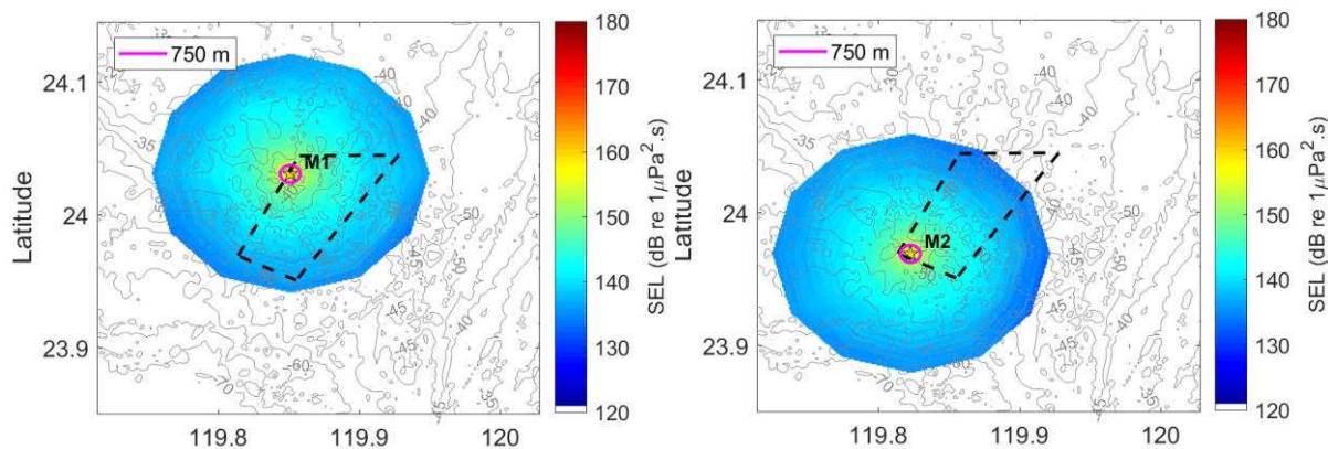
圖 1.9.2-6 原環說 M1~M2 點位打樁施工，經減噪措施後距離 750 公尺之聲壓分布
