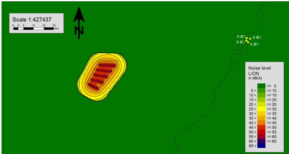
圖 1.4.6-1 變更後營運期間風力機組全頻噪音影響模擬圖
