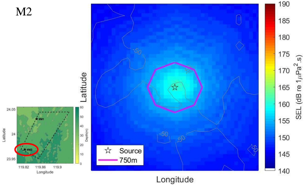
圖 1.1.6-4 M1~M2 點位打樁施工，距離 750 公尺之聲壓分布(減噪後)
