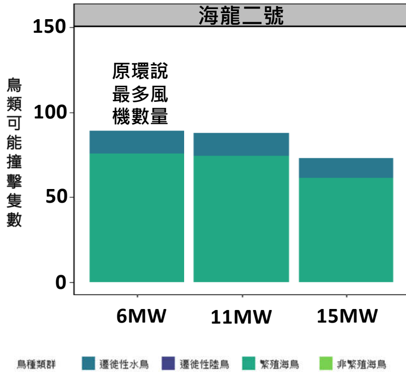
圖 1.6.1-1 海龍二號不同風機配置下各類群鳥種之年撞擊隻次
