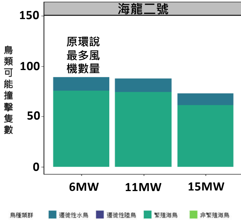
圖 1.9.2-9 海龍二號不同風機配置下各類群鳥種之年撞擊隻次
