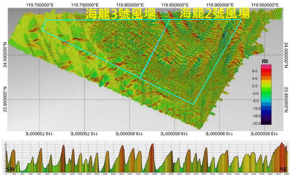
圖 1.8.1-3 海底地形圖
