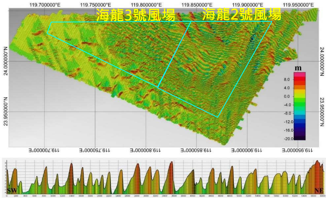
圖 1.3.4-3 海底地形圖
