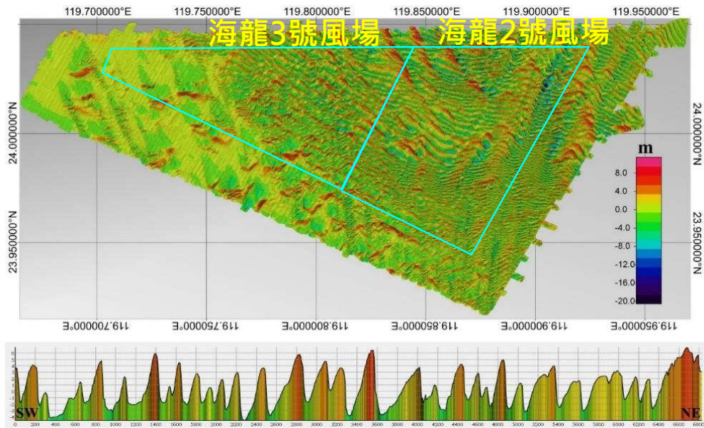
圖 1.6.2-1 海底地形圖
