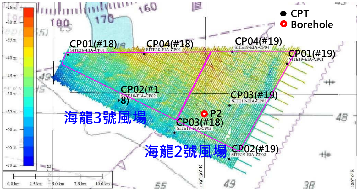
圖 1.8.1-4 地質鑽孔位置圖
