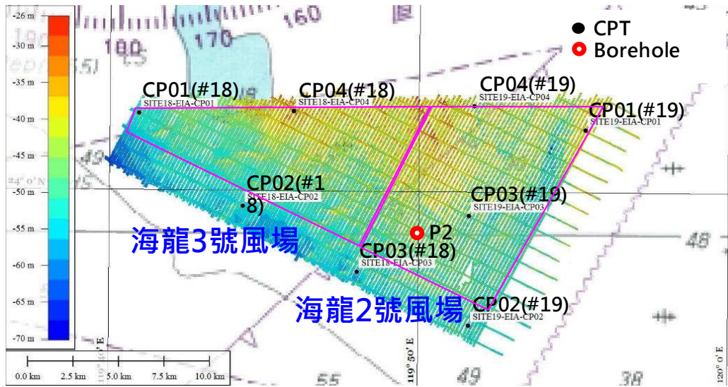
圖 1.6.2-2 地質鑽孔位置圖
