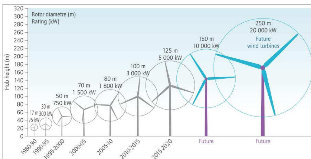
圖 1.3.1-1 國際間風機大型化趨勢
