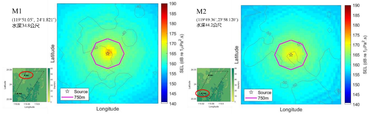
圖 1.7.3-3 M1~M2 點位打樁施工，距離 750 公尺之聲壓分布(減噪前)
