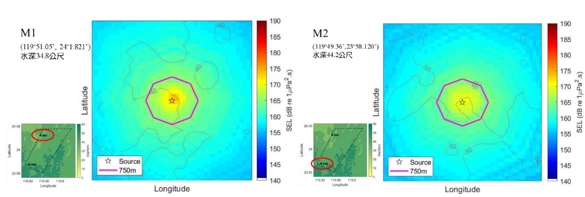
圖 1.3.4-1 M1~M2 點位打樁施工，距離 750 公尺之聲壓分布(減噪前)
