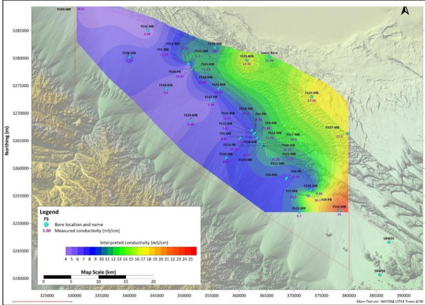
عکس 4-8: فروری 2024 ء EC کچ ء ردا زمینی آب ء سوری
