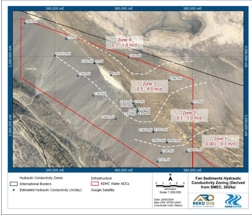
عکس 4-7: ہائیڈرالیک کنڈکٹیویٹی زوننگ
